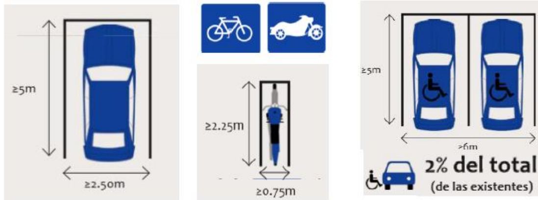
Figura 3. Diseño de estacionamientos (DDE) Fuente: Elaboración propia
