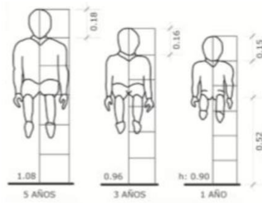
Figura 6. Medidas promedio latinoamericanas Fuente: Arquitectura Habitacional Plazola, volumen III, 1990
