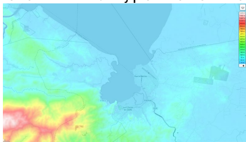
Ilustración 17 / Mapa topográfico de Puerto Barrios, Izabal.
