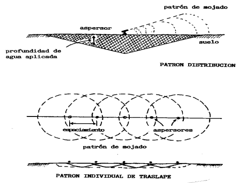
Figura 2.3 Patrón de humedecimiento de un aspersor y efecto del traslape.
