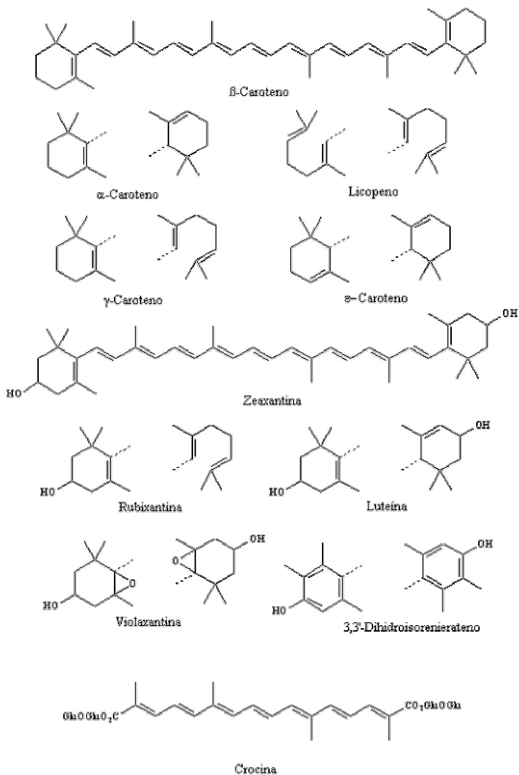
Figura 5. Ejemplos de carotenoides naturales que se encuentran ampliamente distribuidos (6).
