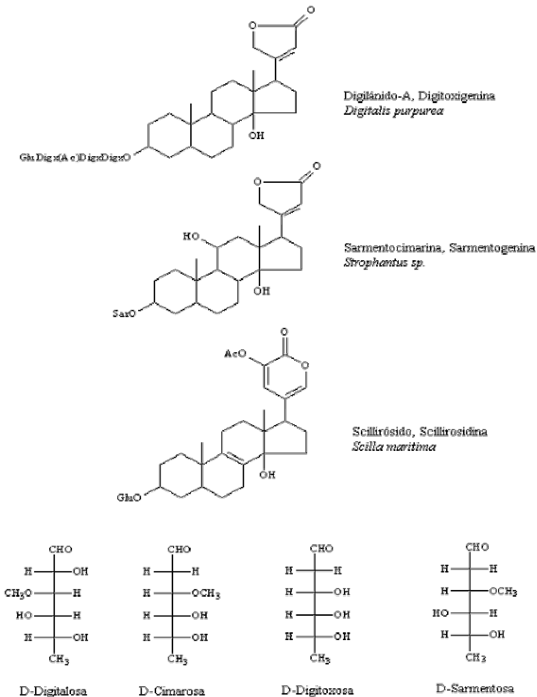
Figura 18. Algunos ejemplos de cardiotónicos y desoxiazúcares naturales (23).
