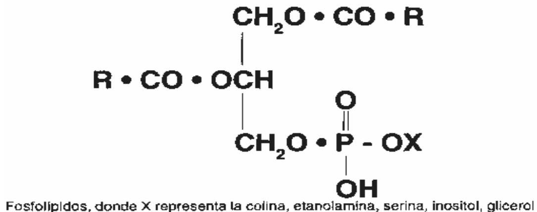
Figura 8. Estructura de fosfolípidos (9).
