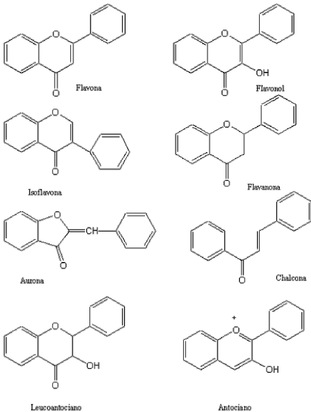
Figura 10. Clasificación de los flavonoides (19).
