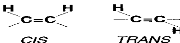
Figura 7. - Estructura en cis y en trans de los dobles enlaces (8)
