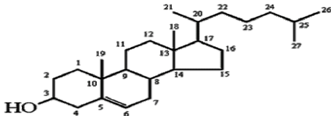
Figura 1 Enumeración de los átomos de carbono en la molécula de colesterol, se observan cadenas laterales de 8 carbonos y un doble enlace en el C-5 (3).
