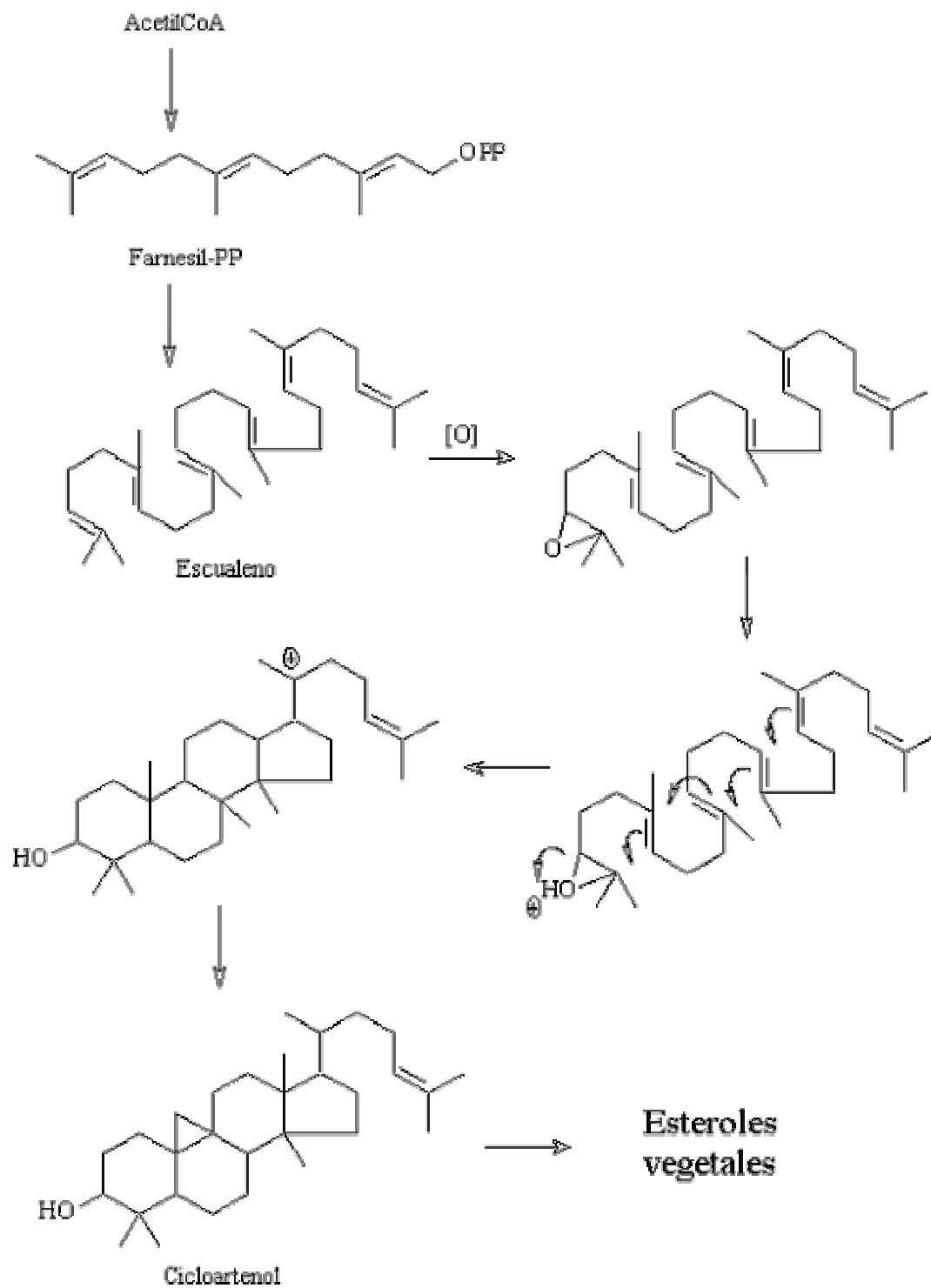
Figura 4. Los esteroides vegetales tienen como precursor inmediato al cicloartenol, a diferencia de los esteroides animales, en los cuales el precursor inmediato es el lanosterol (3).
