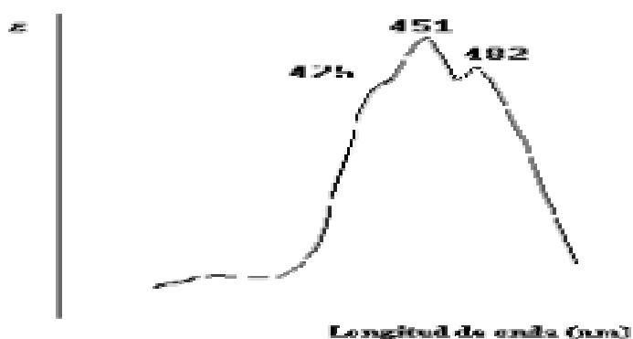
Figura 6. Espectro visible del \beta -caroteno en n-hexano (7).
