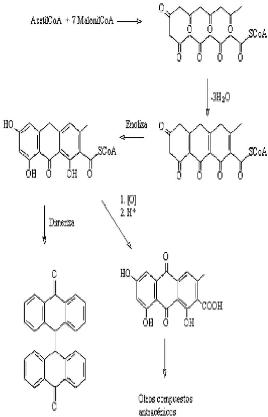
Figura 13. Biogénesis de compuestos antracénicos vía MaloniCoA (23).
