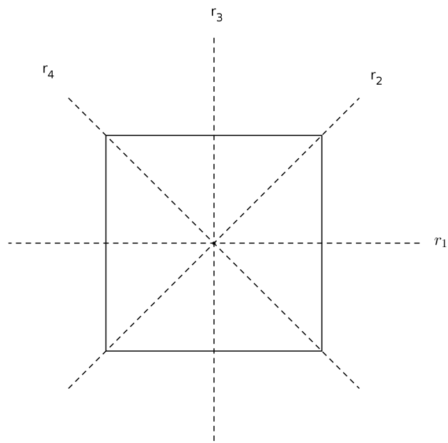
Figura 5. Forma gráfica del grupo D_4
