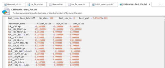
Figura 88. Ventana Best_Par.txt
