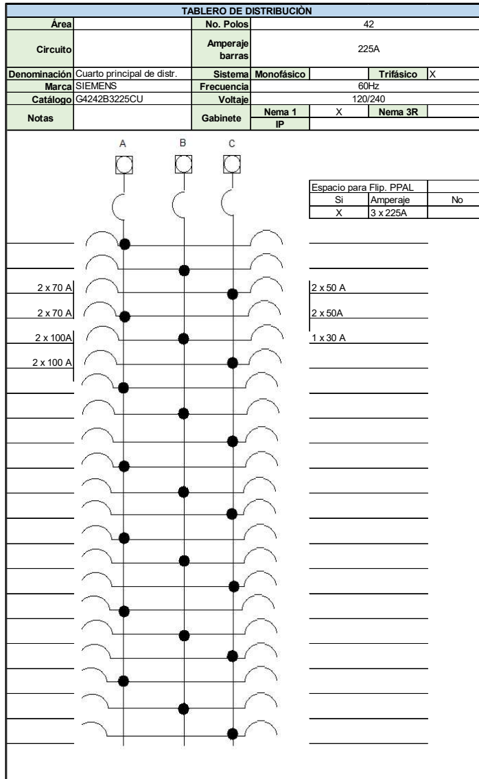
Figura 71. Detalle de elementos en centro de carga área 2
