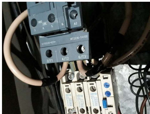
Figura 53. Contactores en módulo de control principal
