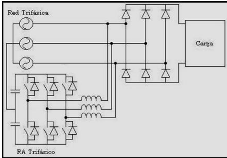
Figura 51. Filtro reductor armónico trifásico
