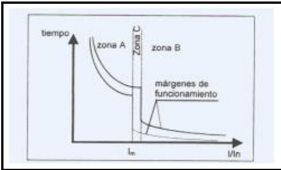
Figura 5. Curva de disparo interruptor termomagnético
