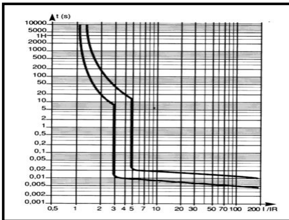
Figura 6. Curva B de disparo
