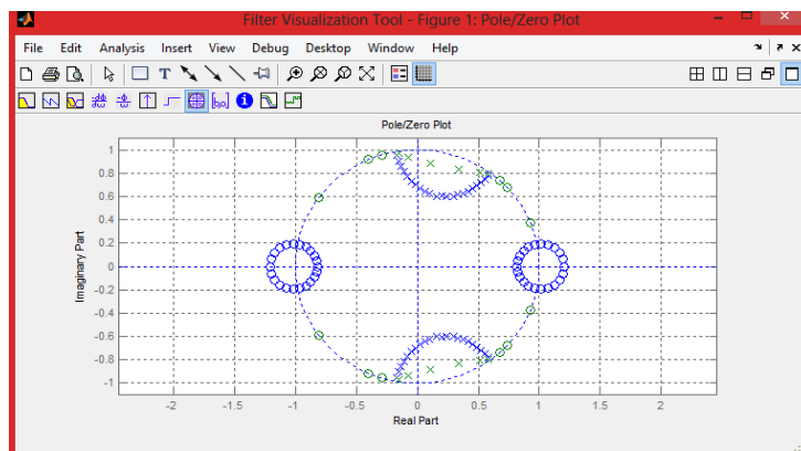
Figura 57. Polos y ceros filtro IIR
