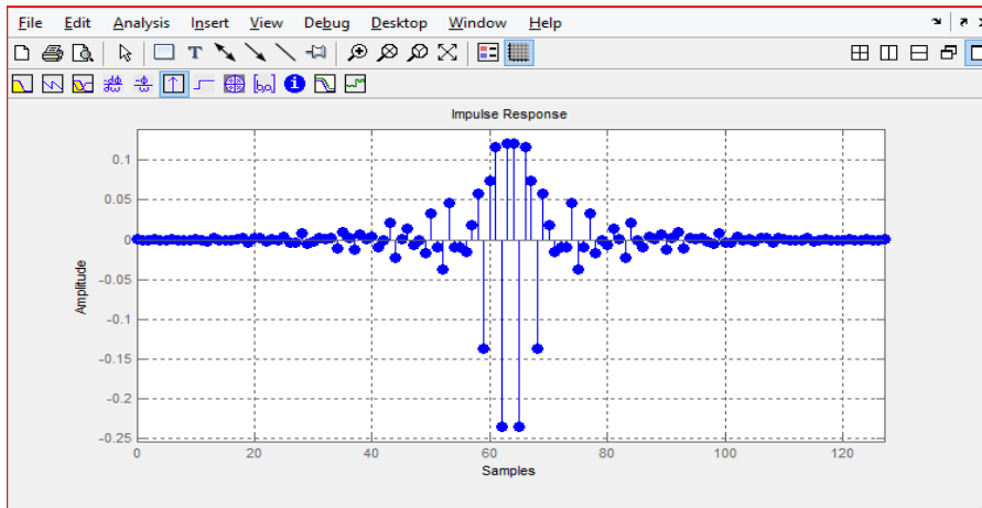
Figura 62. Respuesta al impulso filtro FIR
