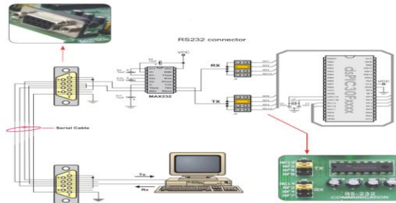
Figura 30. Diagrama de conexión RS-232
