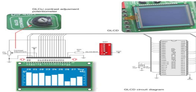
Figura 29. Diagrama de conexión de la GLCD
