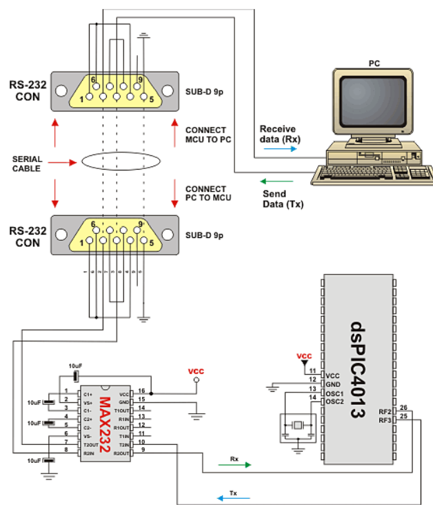
Figura 92. Diagrama de conexión del USAR
