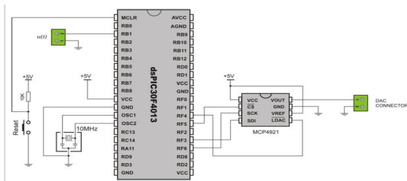
Figura 79. Diagrama de conexión del dsPIC30F4013
