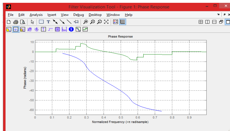
Figura 53. Respuesta de fase filtro IIR
