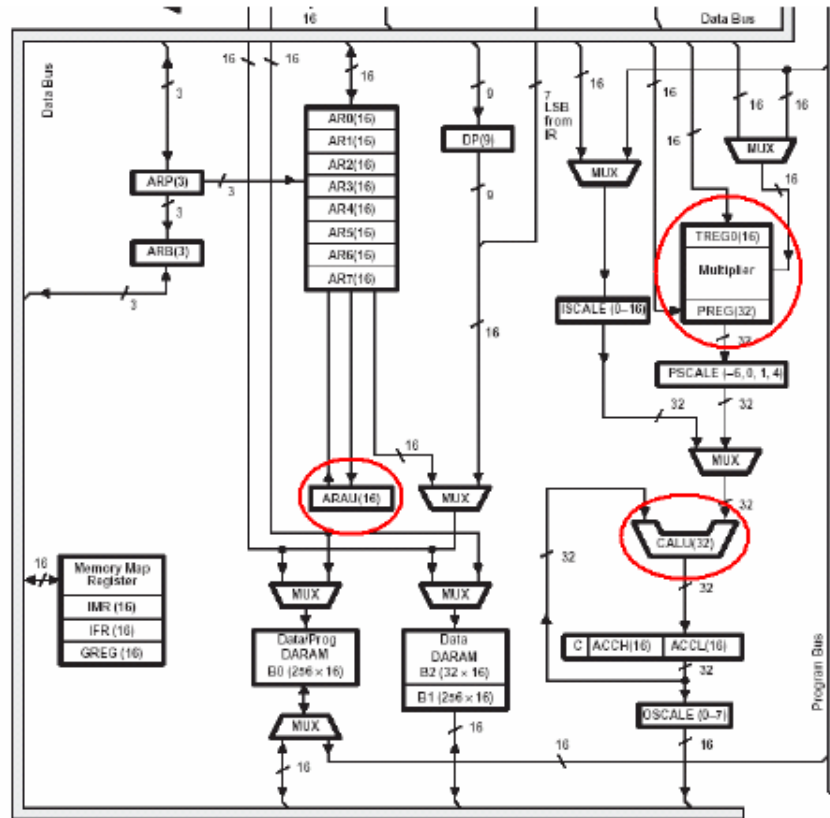
Figura 18. Diagrama de bloques del DSP TMS320F241
