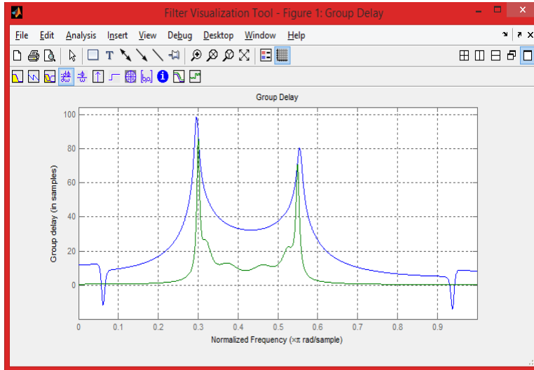
Figura 54. Grupo delay filtro IIR
