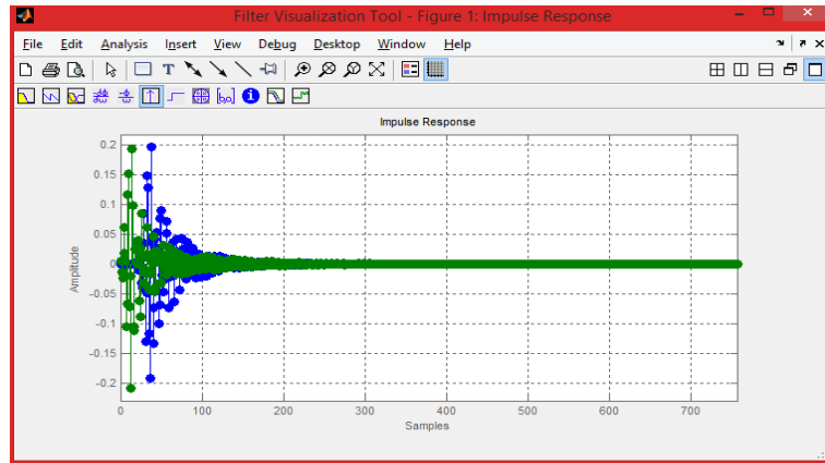
Figura 56. Respuesta al impulso filtro IIR
