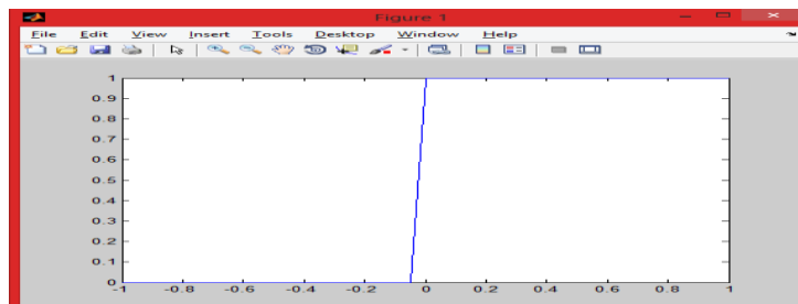
Figura 43. Escalón unitario
