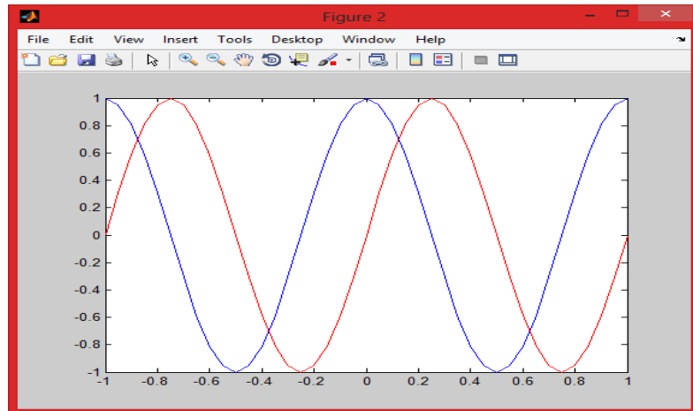
Figura 35. Señal compleja
