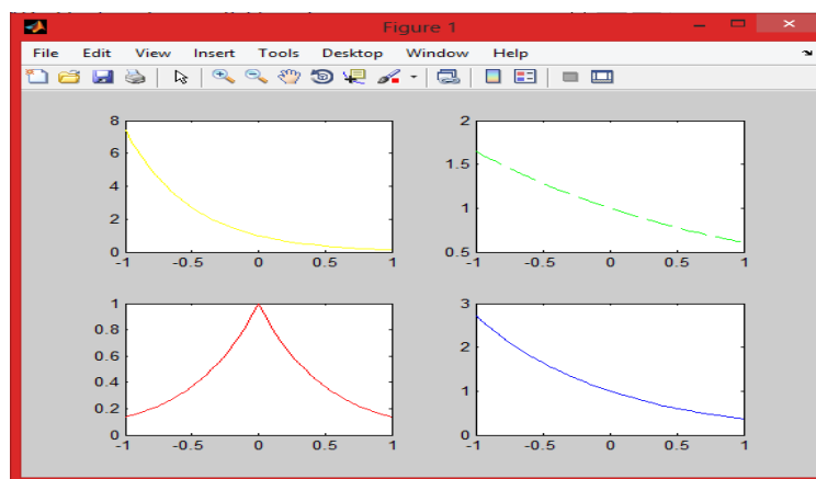
Figura 33. Señales exponenciales
