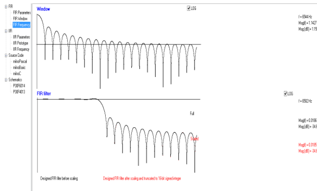
Figura 84. Respuesta en frecuencia filtro FIR
