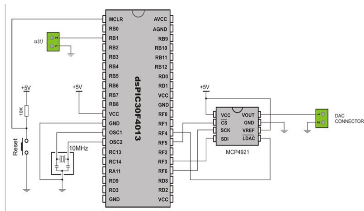
Figura 86. Diagrama de conexión para el filtro FIR
