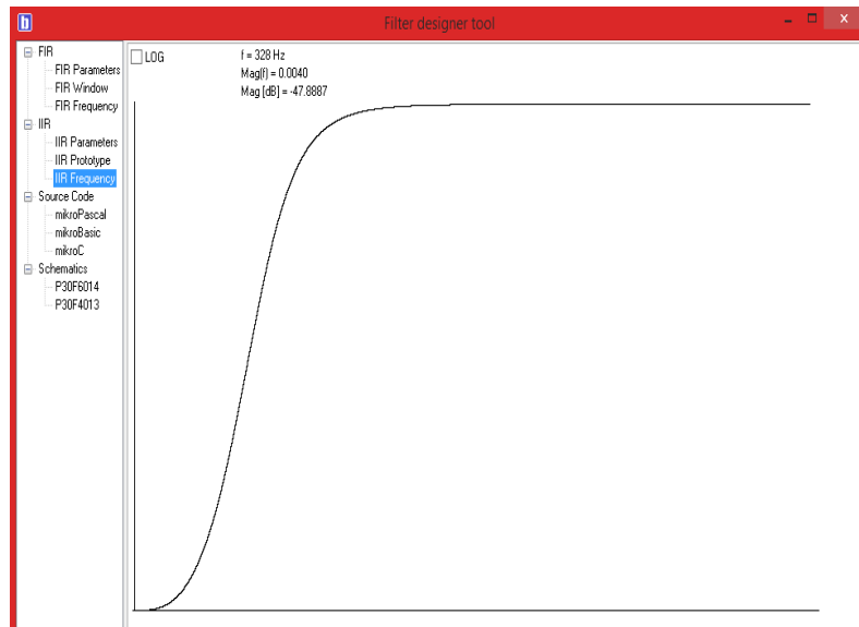
Figura 77. Respuesta en frecuencia de un filtro IIR
