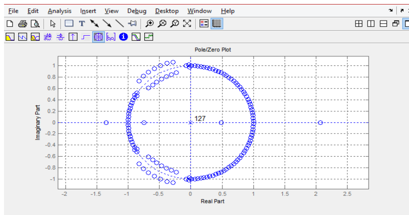
Figura 63. Polos y ceros filtro FIR
