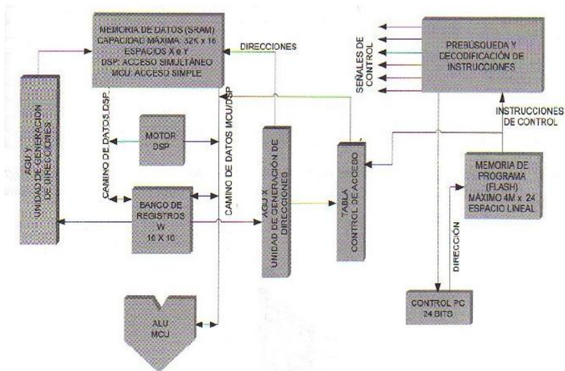
Figura 20. Arquitectura básica de la CPU de los dsPIC30F
