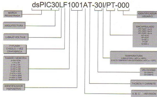
Figura 22. Nomenclatura de la familia dsPIC30F
