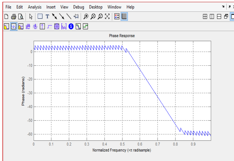
Figura 61. Respuesta de fase filtro FIR
