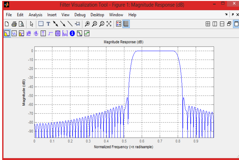
Figura 60. Respuesta de magnitud filtro FIR
