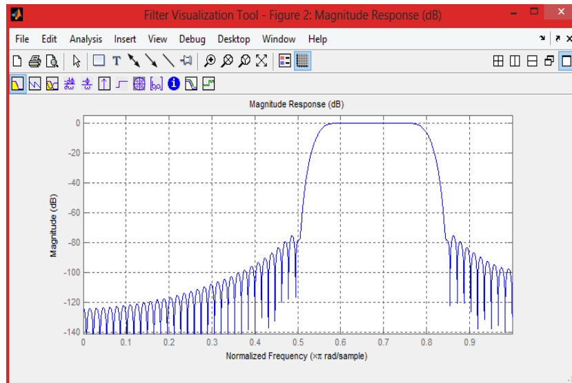
Figura 66. Respuesta en magnitud utilizando una ventana blackman
