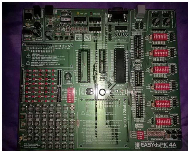
Figura 25. Foto Real de la placa entrenadora EasydsPIC4A
