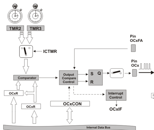
Figura 88. Diagrama Output compare Module
