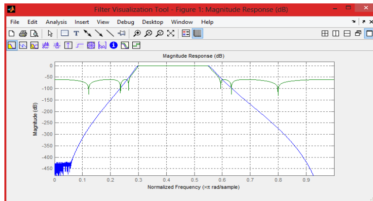
Figura 52. Respuesta en magnitud filtro IIR
