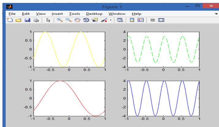
Figura 37. Señales sinusoidales
