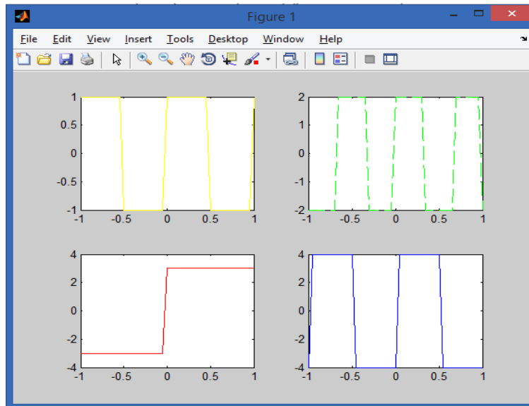
Figura 39. Señales cuadradas
