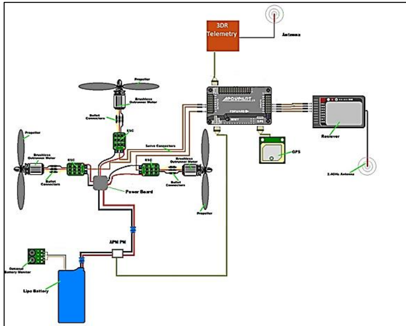
Figura 38. Esquema general de conexión de los componentes
