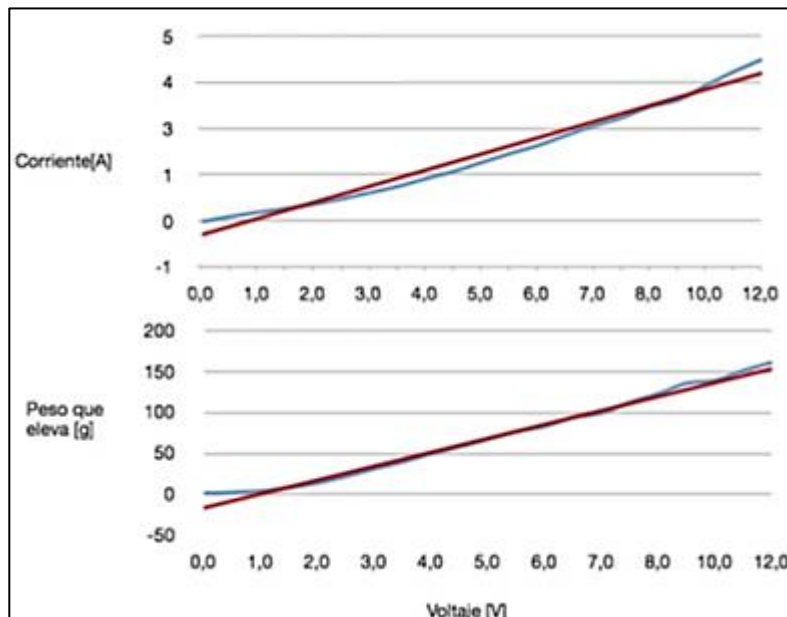
Figura 25. Rectas de respuesta de motor
