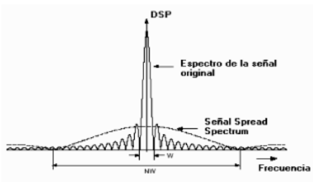
Figura 16. Densidad espectral de una señal spread spectrum
