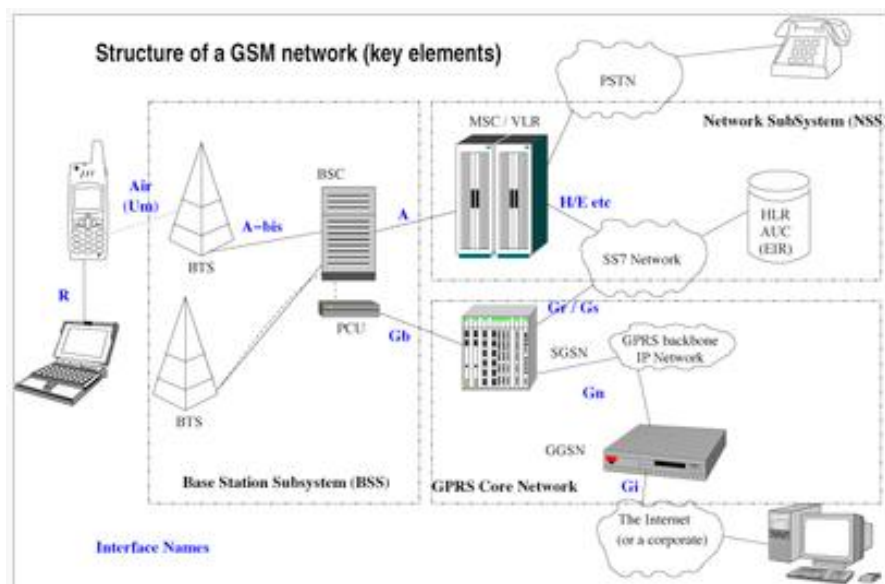
Figura 25. Esquema de itinerancia en red GSM
