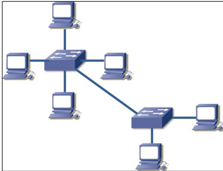
Figura 6. Topología en estrella extendida
