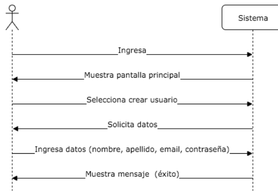
Figura 2. Diagrama de secuencia de creación de usuario
