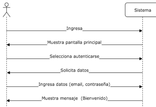
Figura 3. Diagrama de secuencia de autenticación de usuario
