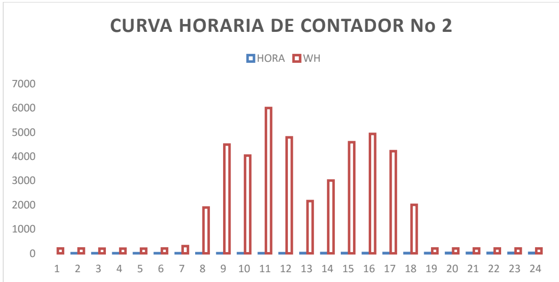
Figura 14. Curva de consumo de energía contador número 2
