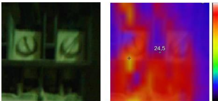
Figura 16. Termografía contador No.1
