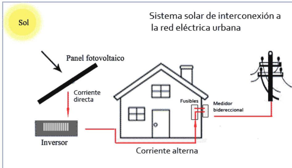
Figura 3. Sistema fotovoltaico para conexión a la red
