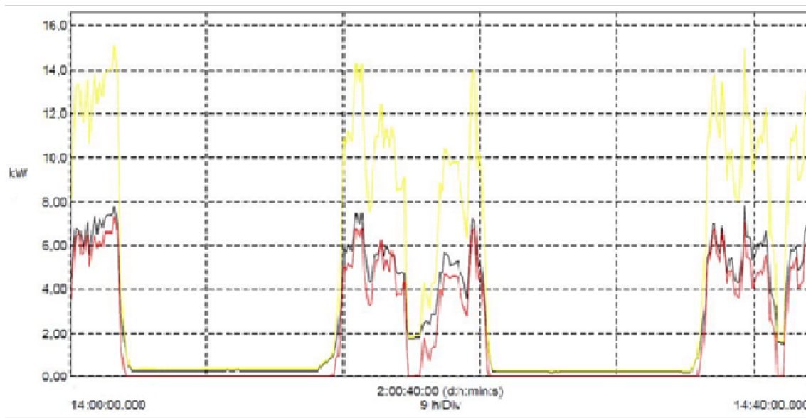
Figura 8. Análisis de demanda en Kw
