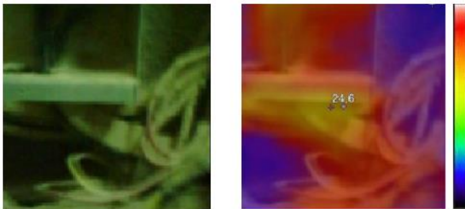
Figura 22. Cableado contador No 1
