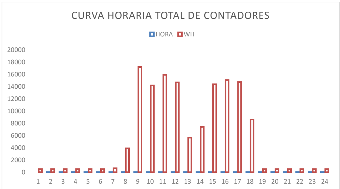
Figura 15. Curva de consumo de energía total de contadores
