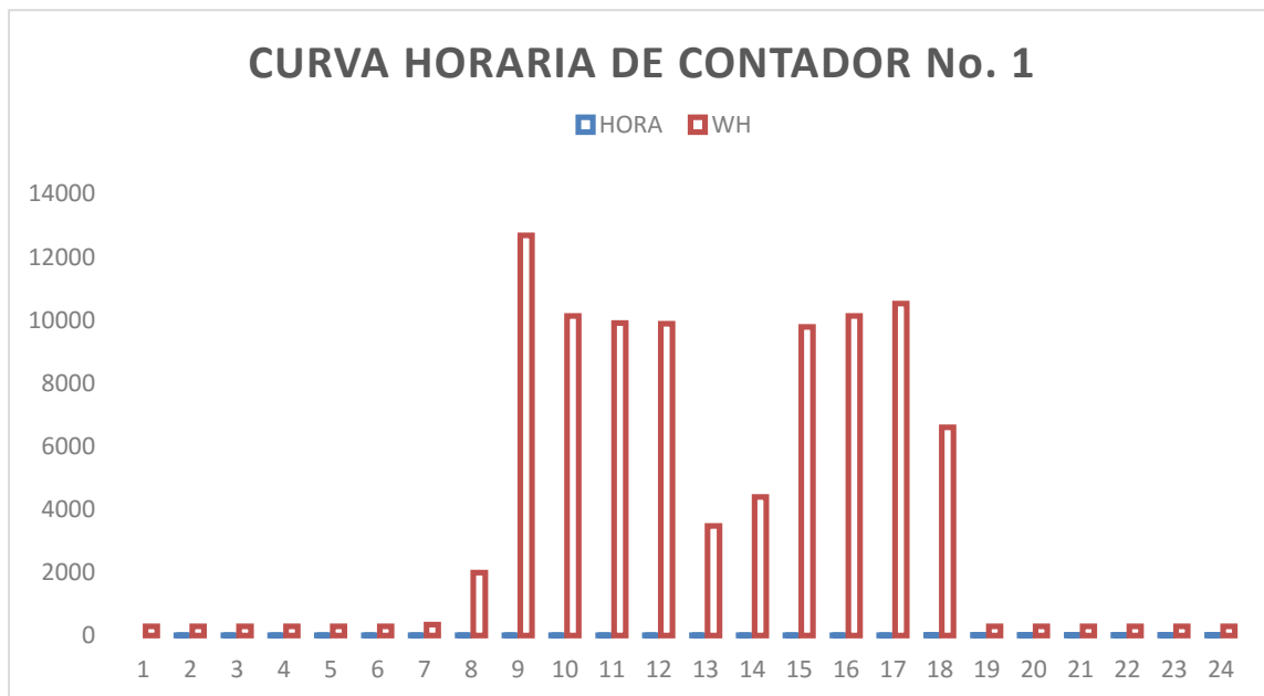
Figura 13. Curva de consumo de energía contador número 1
