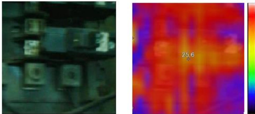
Figura 21. Breaker principal contador No 2
