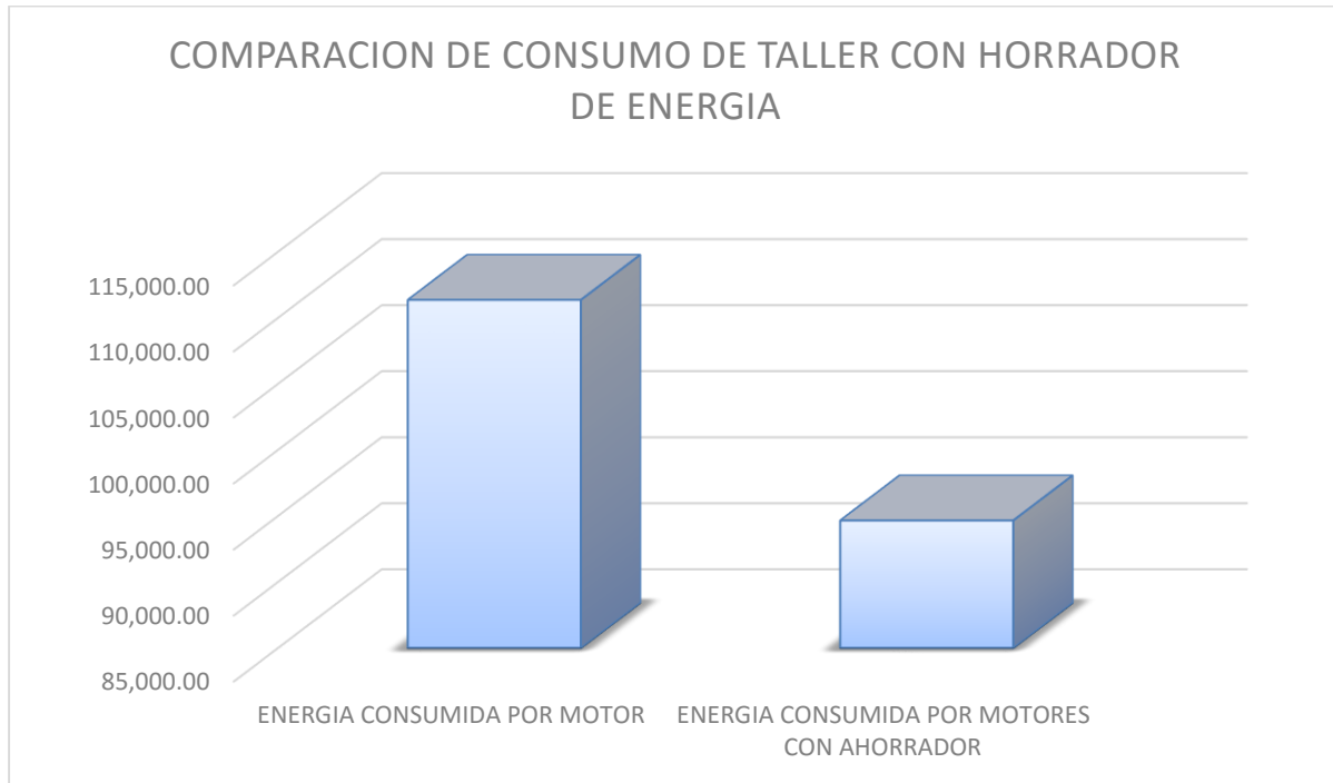
Figura 27. Comparación de consumo de taller con ahorrador de energía
