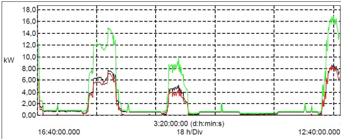
Figura 12. Diagrama de consumo de energía contador número 1
