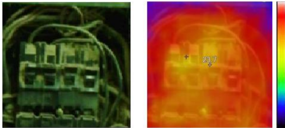
Figura 19. Flipón principal de cortadora
