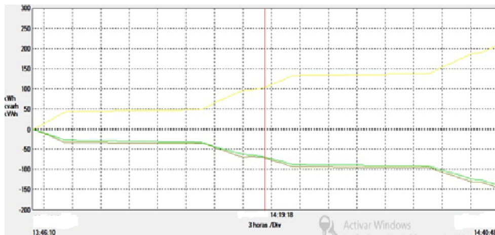
Figura 11. Curva de potencia acometida principal
