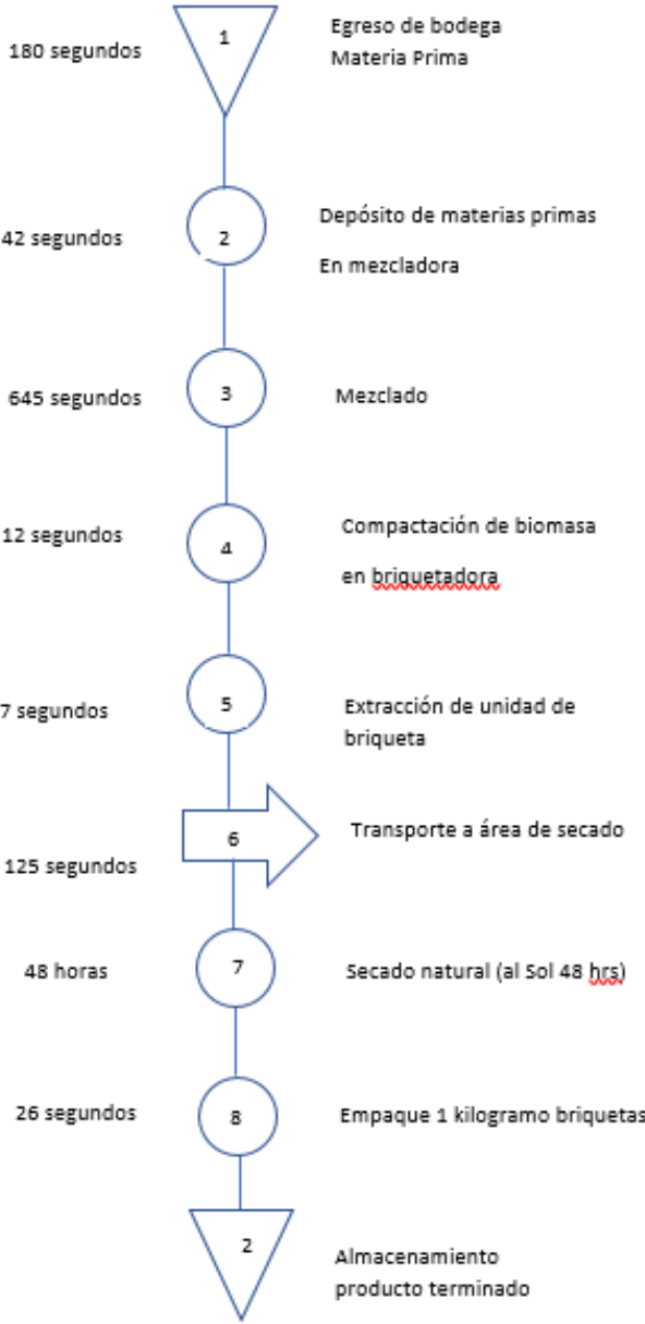
Figura 17. Diagrama de flujo para elaboración de briqueta Aserrín 60% , Cascarilla de café 25 % olote 10 % aglutinante 5 %
