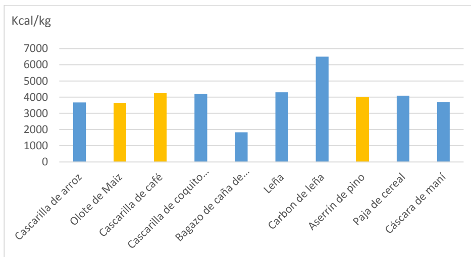
Figura 7. Gráfica de poder calorífico de biomásas
