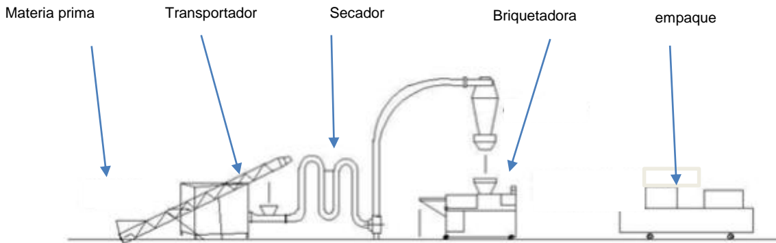
Figura 25. Maquinaria para producción industrial
