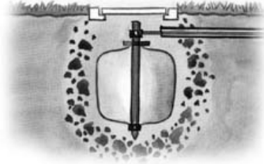
Figura 68. Ejemplo de un SPT con su registro
