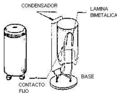
Figura 8. Arrancador
