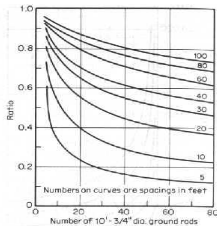
Figura 71. Porcentaje de conductividad de electrodos de tierra en paralelo en un área de electrodos aislados
