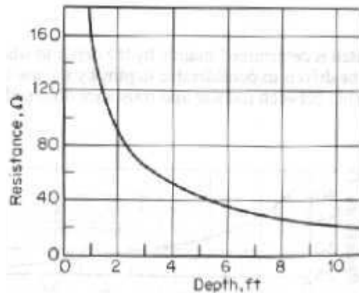
Figura 70. Variación de la resistencia con la profundidad, para un electrodo de 1.02 plg de diámetro en suelo muy húmedo
