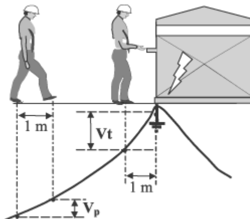
Figura 73. Potenciales peligrosos de toque y de paso en subestación de media y baja tensión
