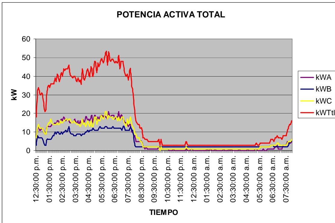
Figura 48. Potencia activa trifásica del edificio T1
