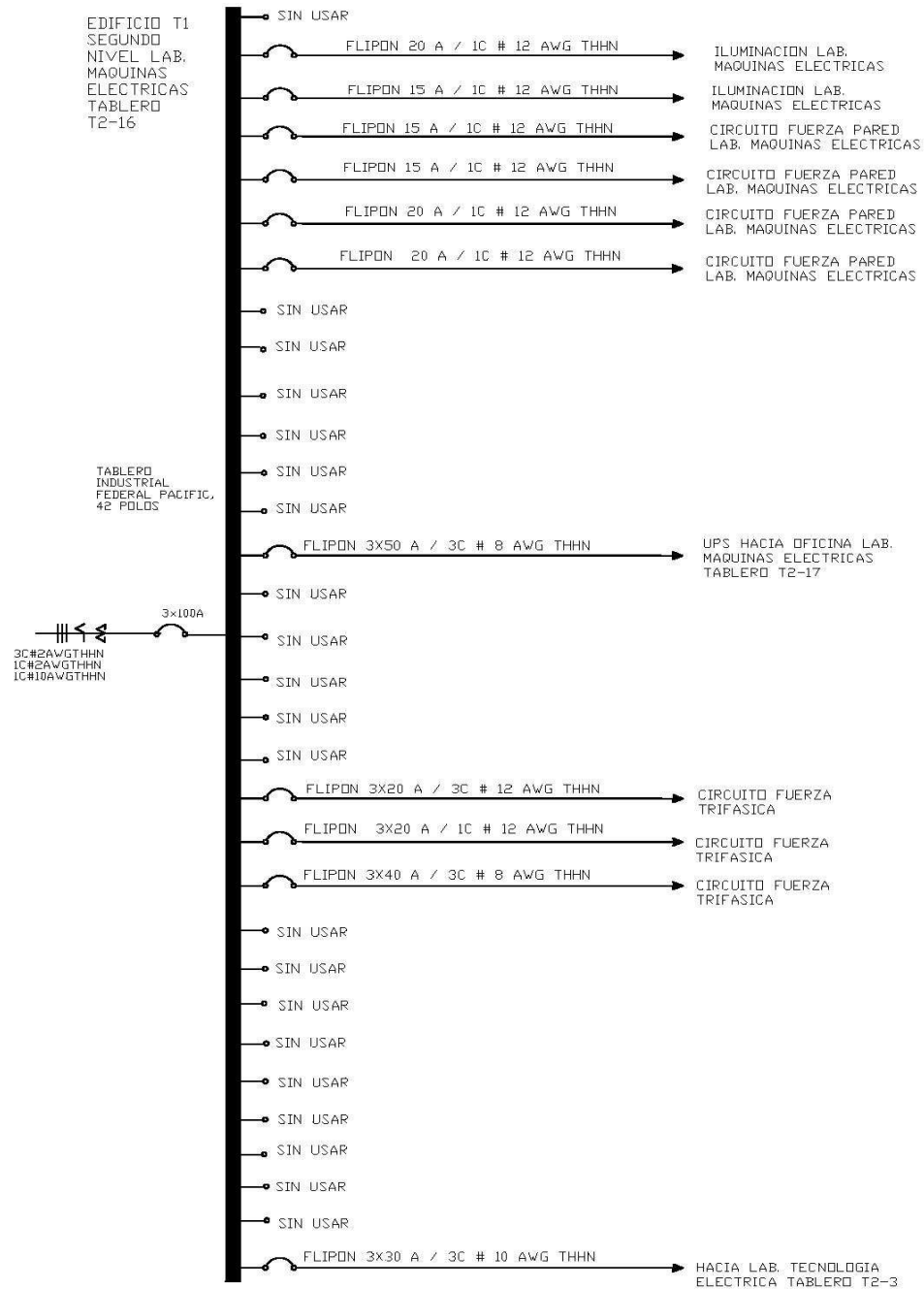
Figura 29. Diagrama unifilar tablero de distribución T2-16 edificio T1
