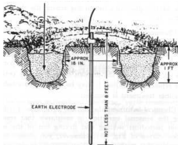
Figura 63. Zanja alrededor del electrodo de tierra con compuestos químicos que mejoran la resistividad
