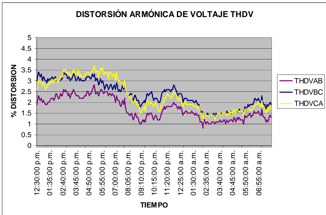
Figura 52. Distorsión armónica de voltaje en porcentaje del edificio T1
