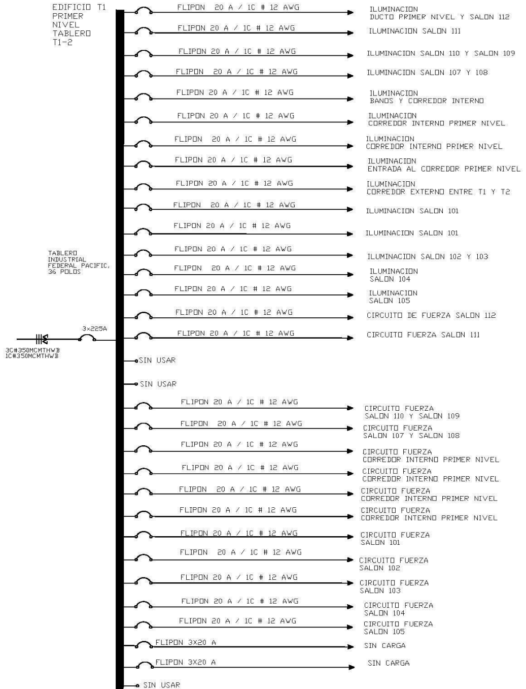
Figura 19. Diagrama unifilar tablero de distribución T1-2 edificio T1
