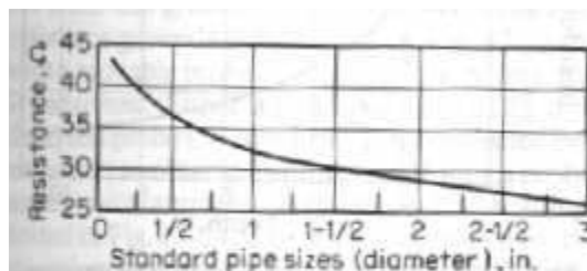
Figura 69. Relación entre el diámetro de la varilla y la resistencia de tierra
