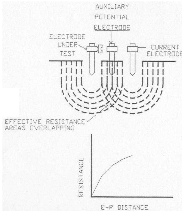
Figura 81. Áreas de disimulación de las áreas de influencia de los electrodos P y C respecto a E
