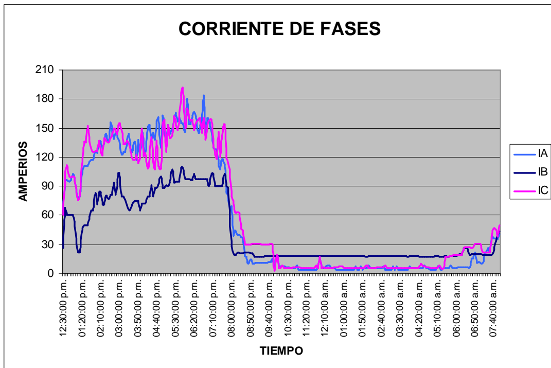
Figura 46. Gráfica corriente de fases – tiempo del edificio T1
