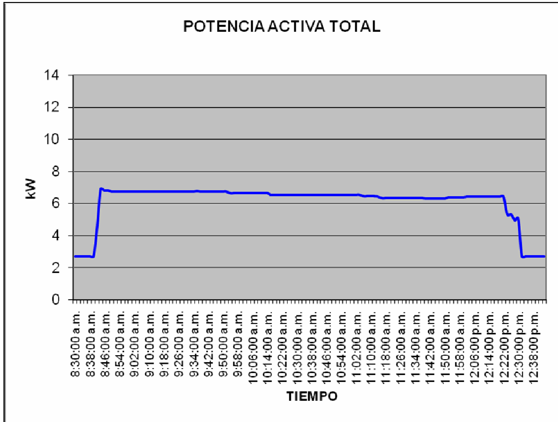
Figura 55. Potencia activa total del edificio T6
