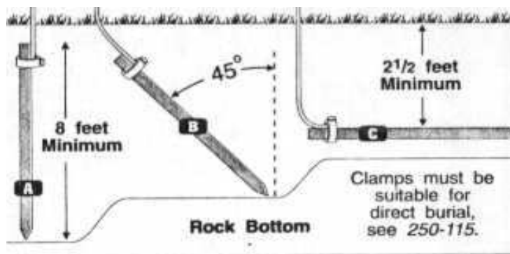
Figura 65. Formas en las que se puede enterrar un electrodo en la tierra
