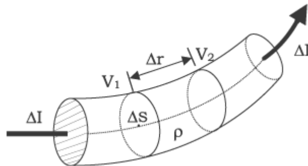
Figura 60. Modelo analítico de suelo conductor de resistividad ( \Delta\rho ) homogénea
