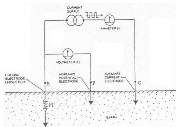
Figura 79. Descripción gráfica de cómo utilizar el medidor EECOS modelo 2300
