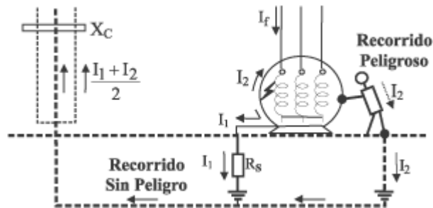
Figura 72. Protección en caso de energización de las masas
