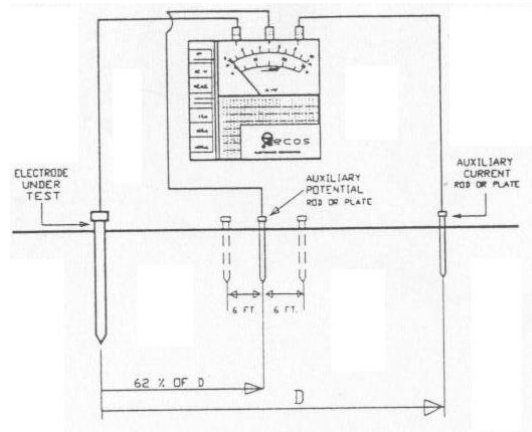
Figura 80. Descripción grafica del Método del 62%
