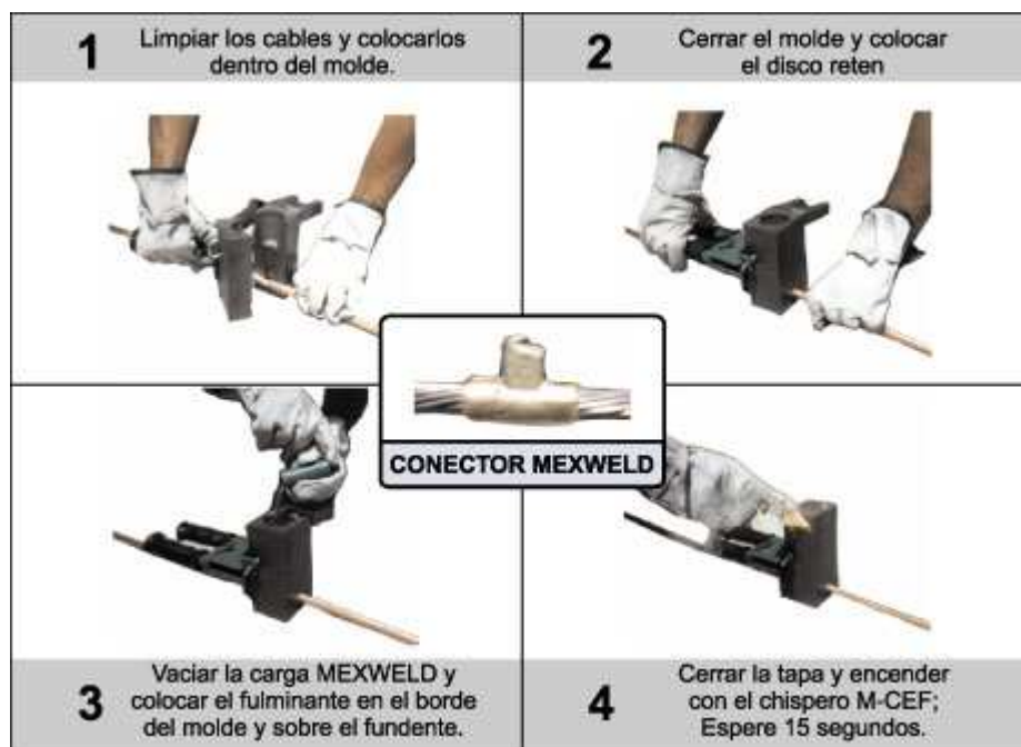
Figura 83. Proceso del conector soldable exotérmico
