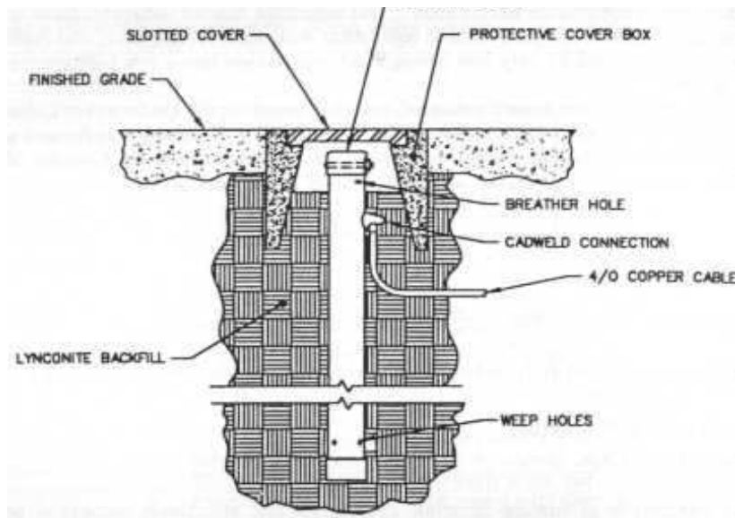
Figura 62. Varilla electroquímica
