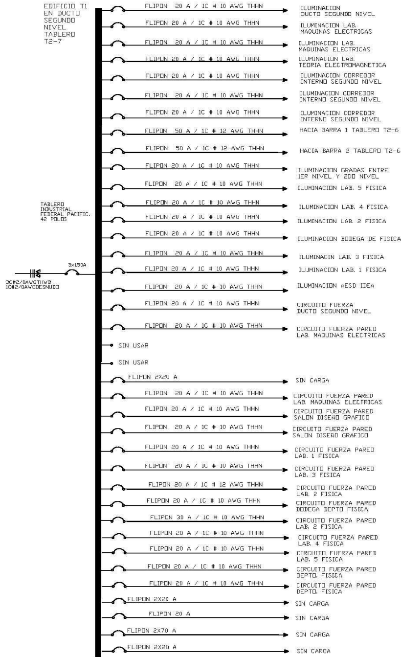
Figura 20. Diagrama unifilar tablero de distribución T2-7 edificio T1
