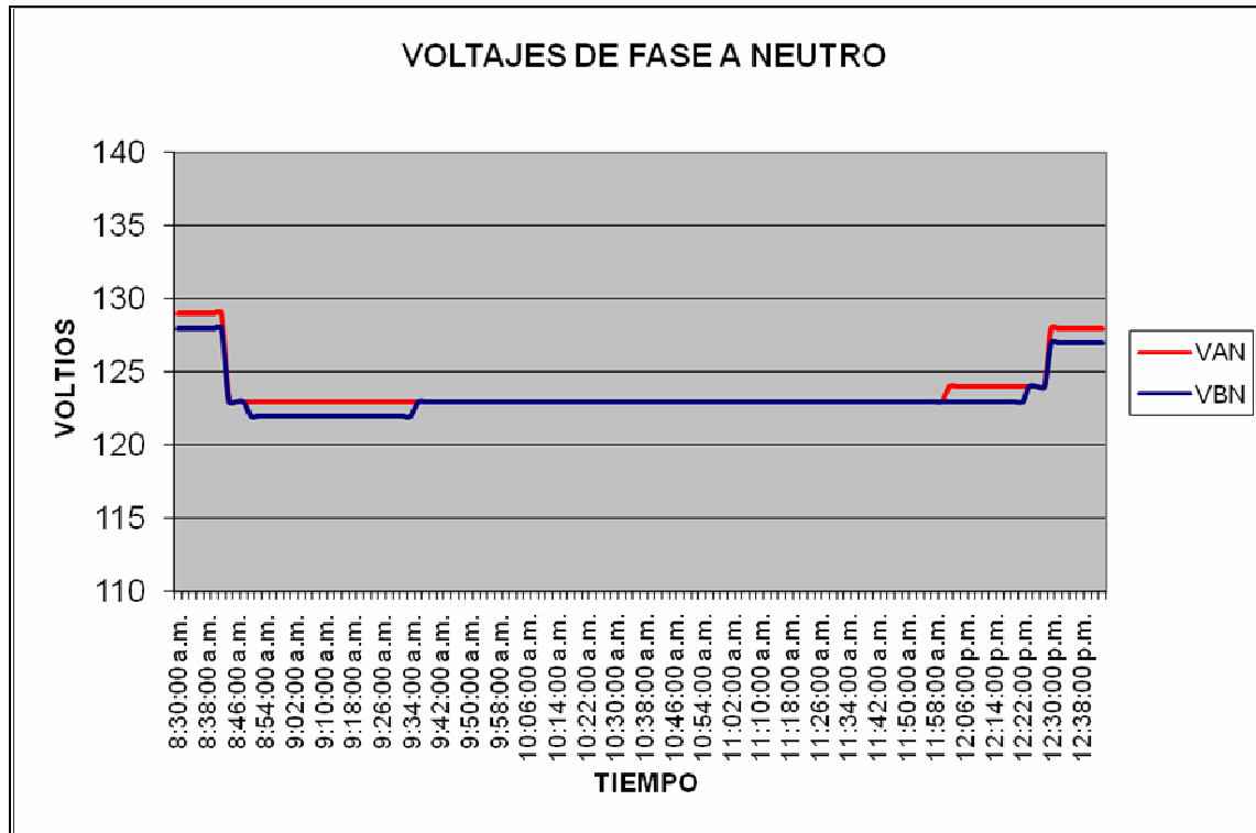
Figura 54. Tensión de fases del edificio T6
