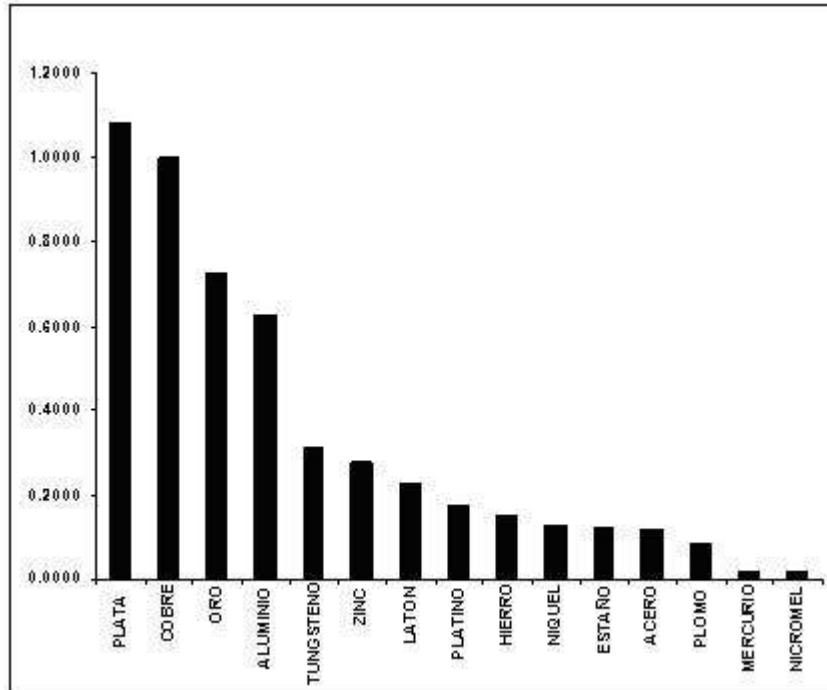
Figura 1. Conductancias de diferentes metales
