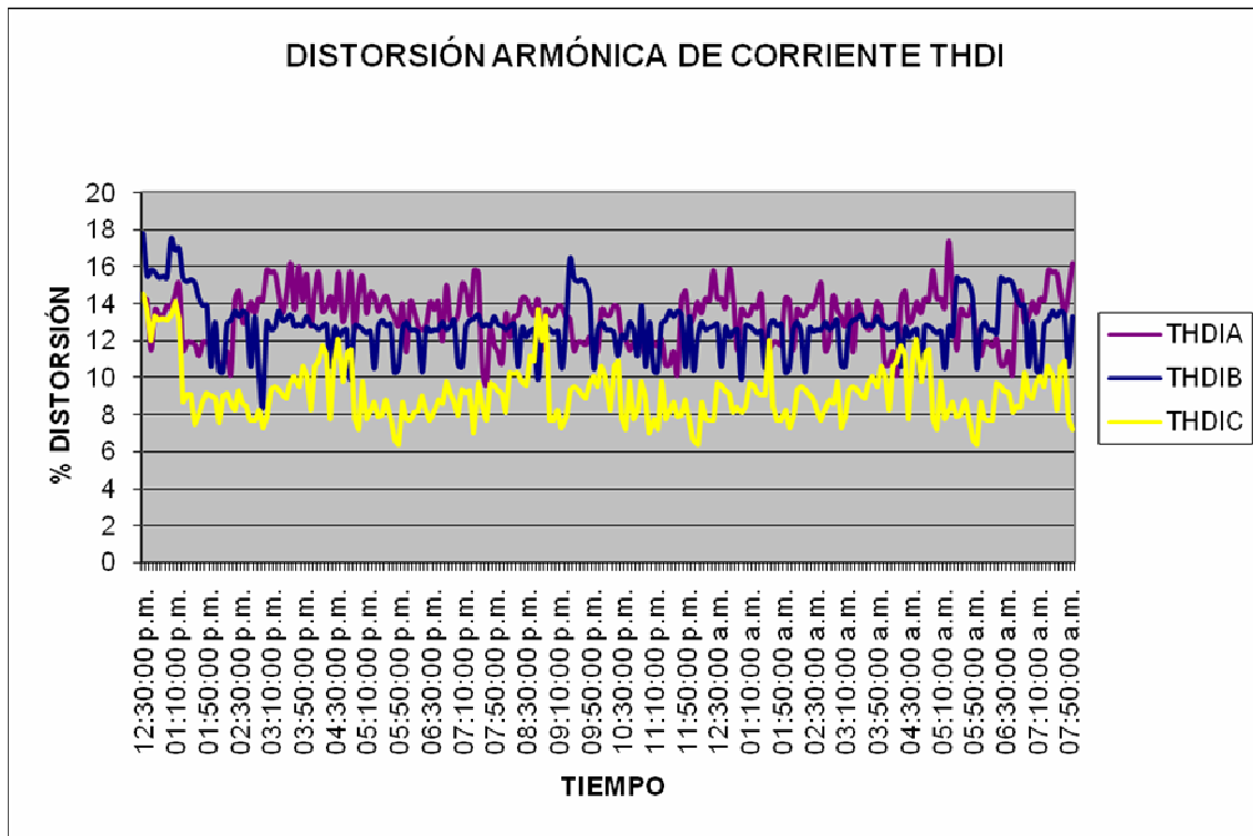
Figura 51. Distorsión armónica de corriente en porcentaje del edificio T1
