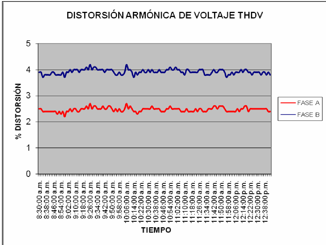
Figura 59. Distorsión armónica de voltaje en porcentaje del edificio T6
