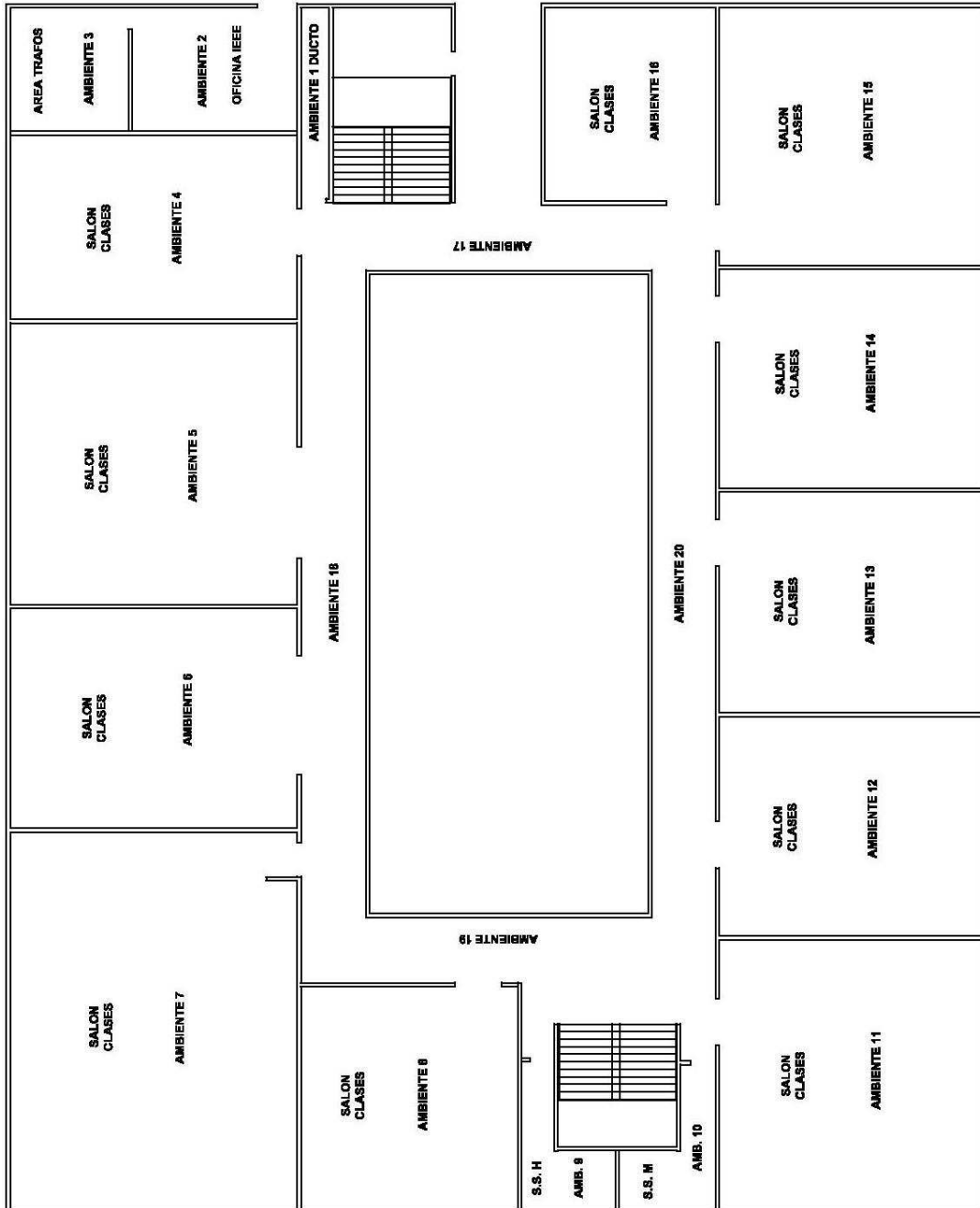
Figura 43. Nivel 1 edificio T1 por ambiente
