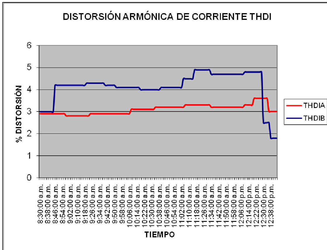
Figura 58. Distorsión armónica de corriente en porcentaje del edificio T6
