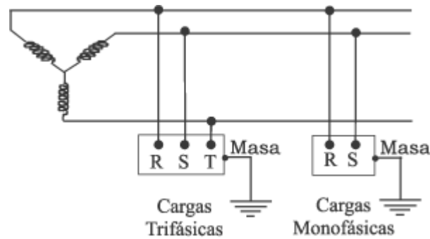
Figura 75. Conexión de cargas en sistema delta o estrella sin neutro a tierra
