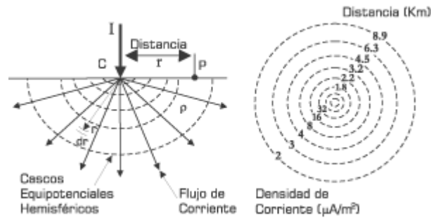
Figura 76. Dispersión de corrientes a frecuencia industrial en el suelo hemisferios concéntricos
