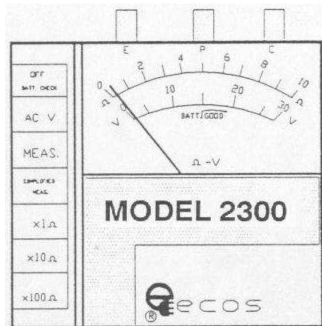
Figura 78. Instrumento de medición de tierra física EECOS modelo 2300
