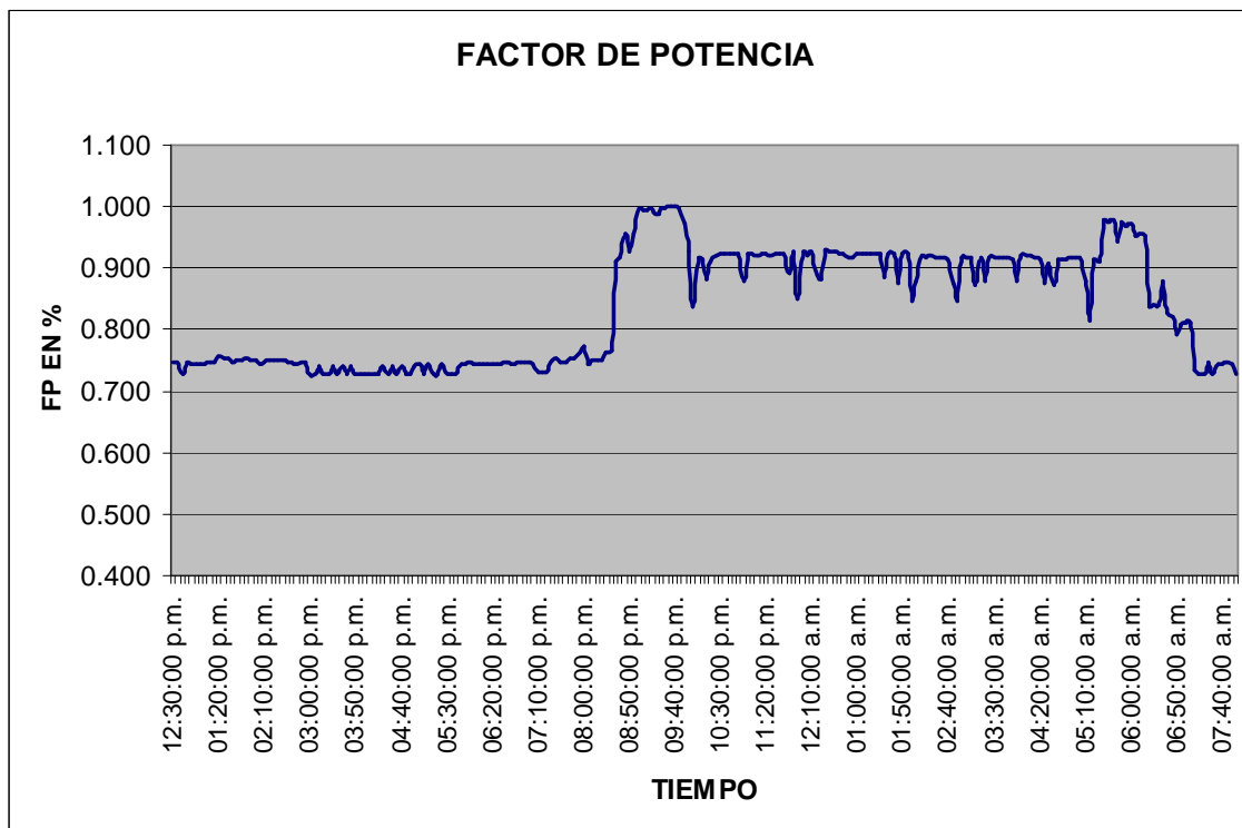
Figura 50. Análisis del Factor de potencia del edificio T1
