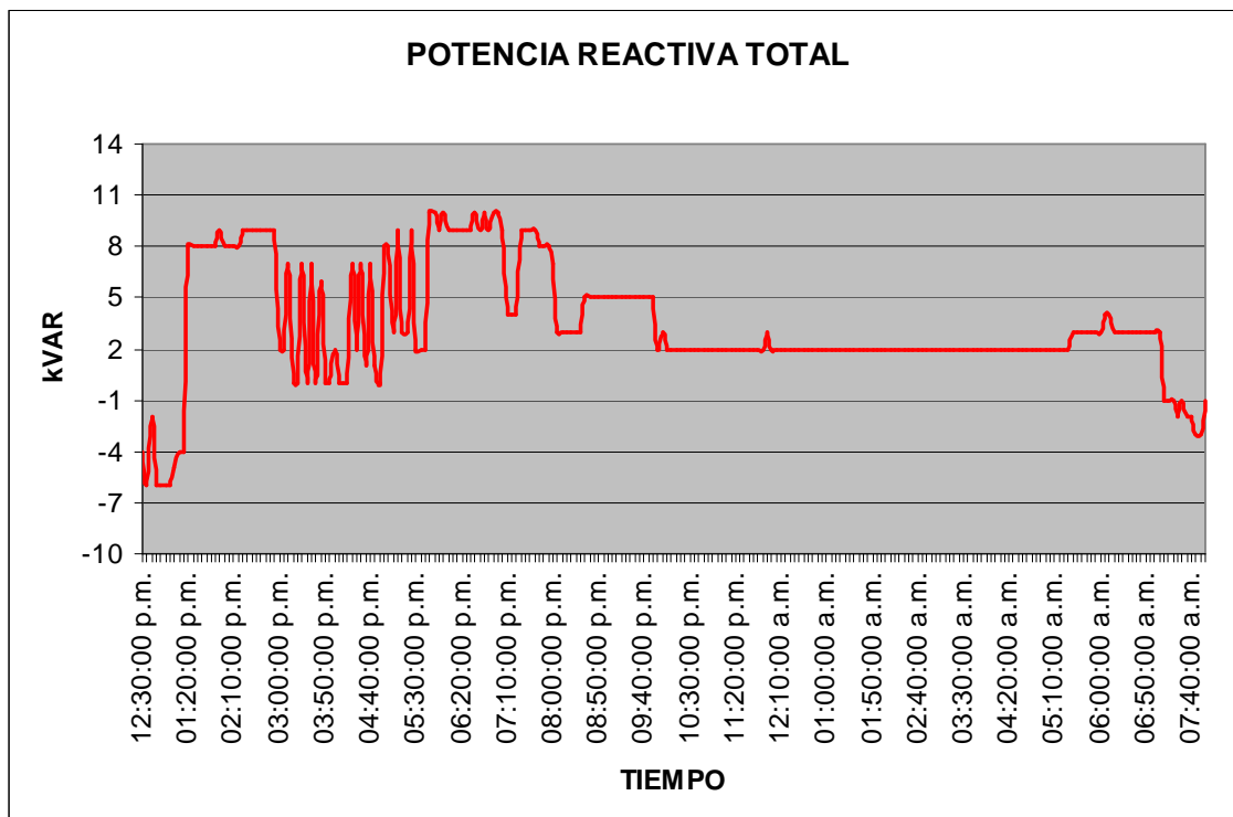
Figura 49. Potencia reactiva del edificio T1
