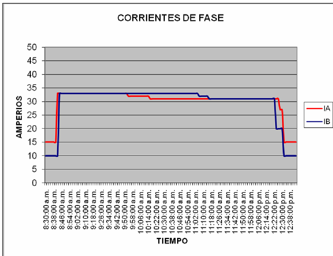
Figura 53. Corrientes de fase del edificio T6
