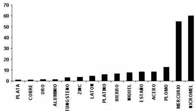
Figura 2. Conductancias relativas de diferentes metales
