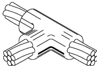
CONEXION DE CABLE PARA VARRILA CADWELD TIPO "TA" DETALLE 2
