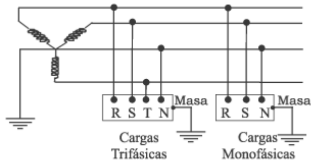
Figura 74. Conexión de cargas en sistemas estrella con neutro a tierra
