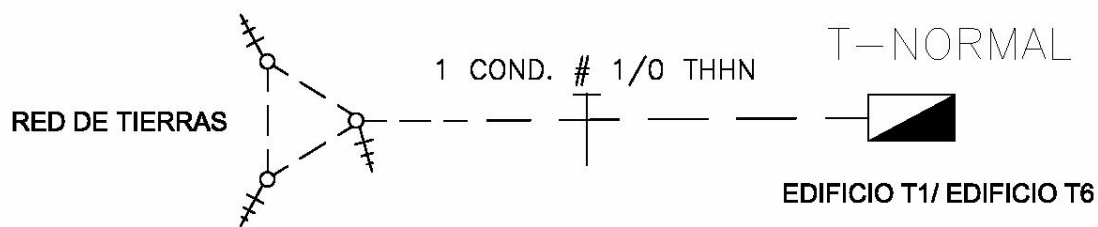
Figura 88. Introducción de la red de tierras al tablero principal de los edificios T1 y T6
