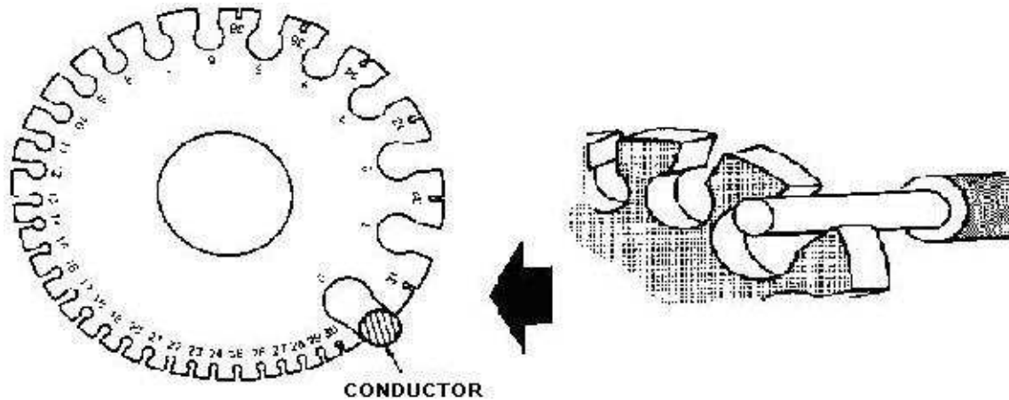
Figura 4. Calibrador o galga para conductores eléctricos
