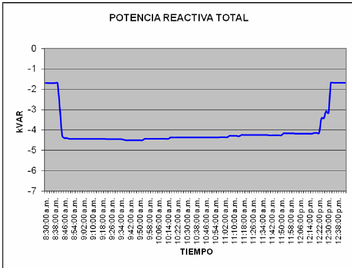
Figura 56. Potencia reactiva del edificio T6
