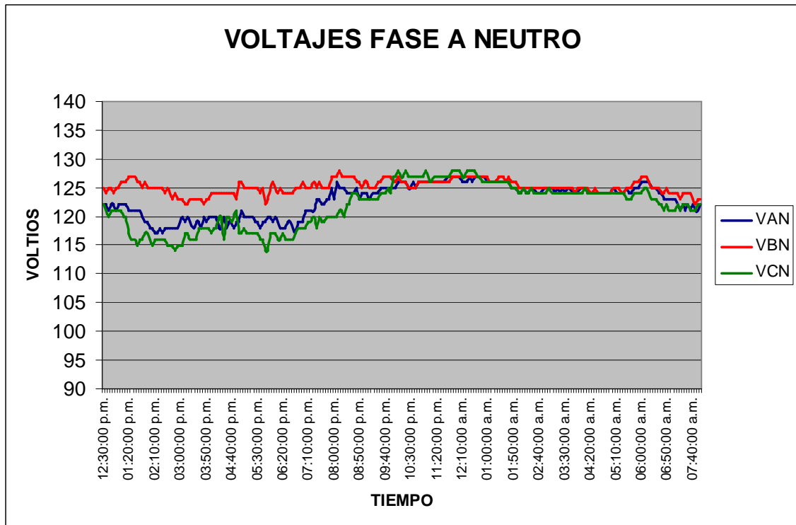
Figura 47. Tensión de fases del edificio T1
