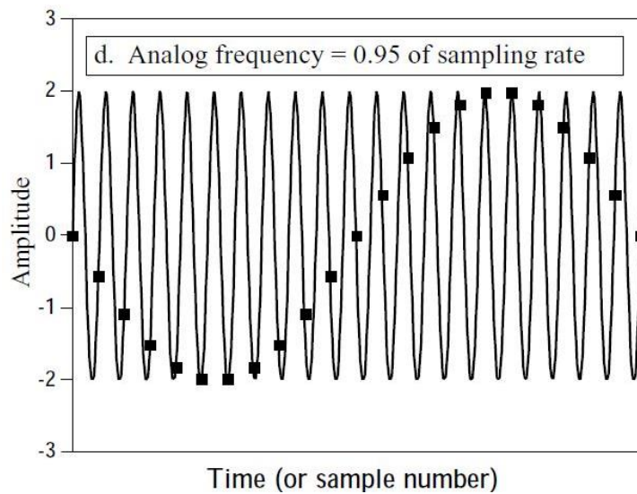
Figura 3. Efecto de aliasing
