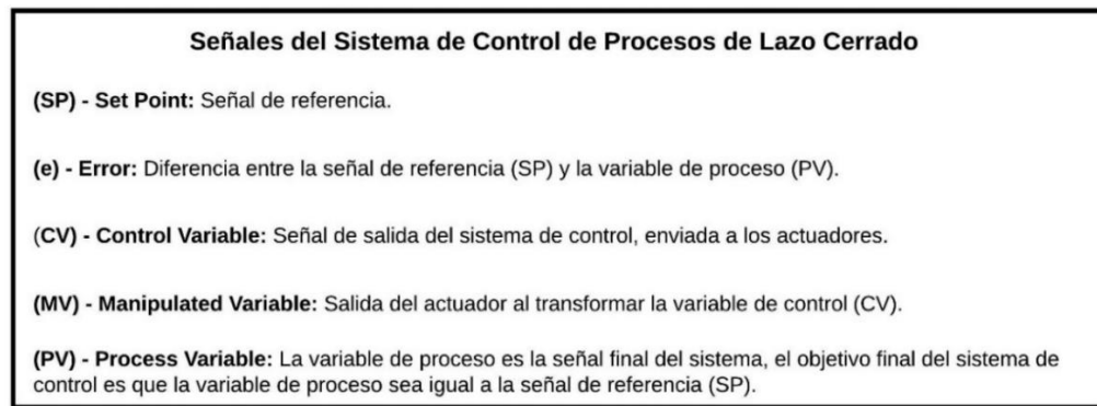
Figura 6. Señales del sistema de control de lazo cerrado
