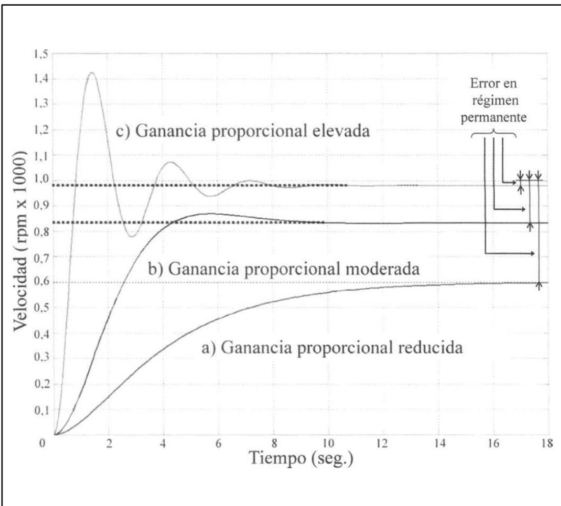
Figura 11. Respuesta de un motor a diferentes ganancias ( K_p )
