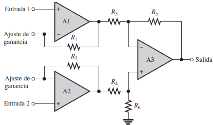
Figura 1. Amplificador de instrumentación básico
