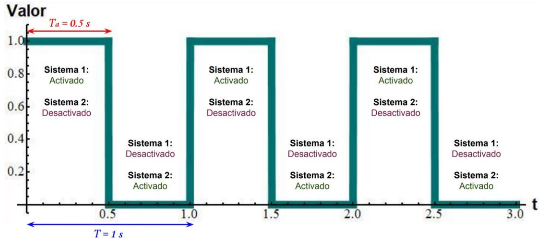
Figura 45. Ejemplo de señal de control
