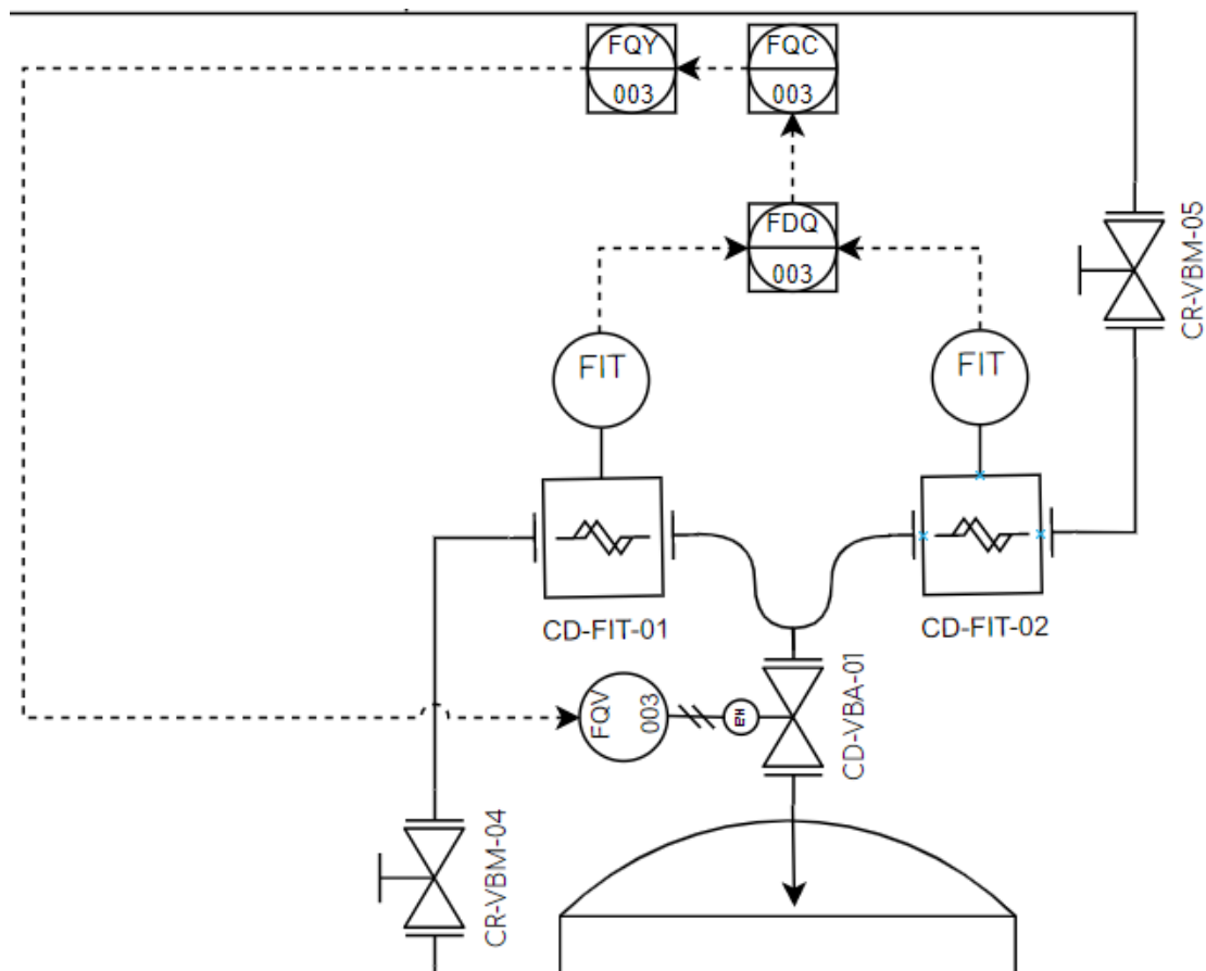
Figura 58. Diagrama P&ID con sistema de control 003
