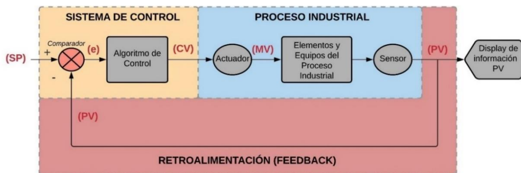
Figura 7. Diagrama del sistema de control de lazo cerrado
