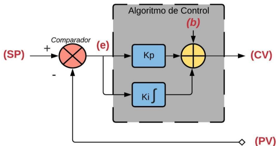
Figura 15. Sistema de control proporcional – integral
