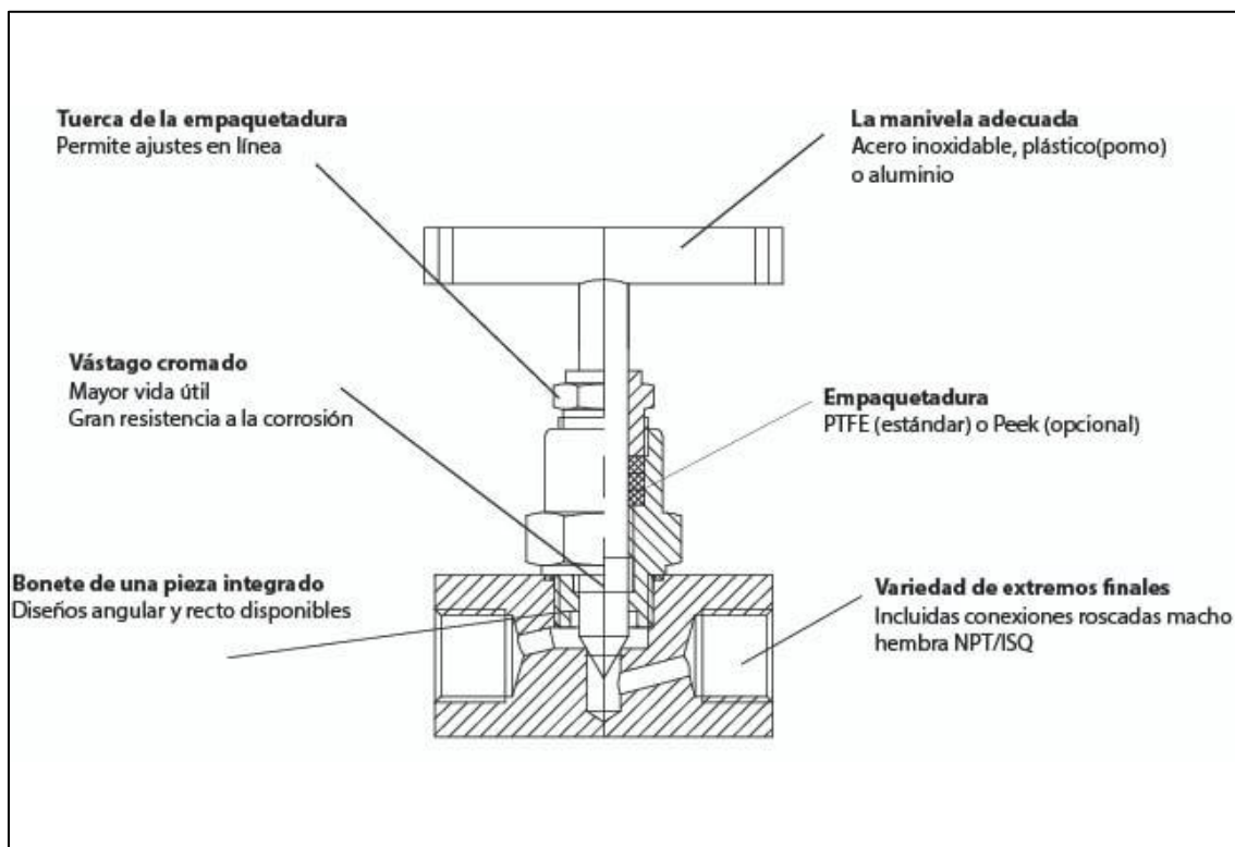
Figura 31. Partes de una válvula de aguja
