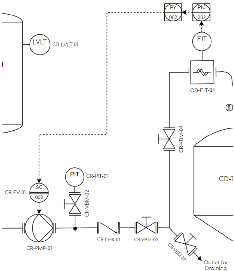
Figura 56. Diagrama P&ID con sistema de control 002
