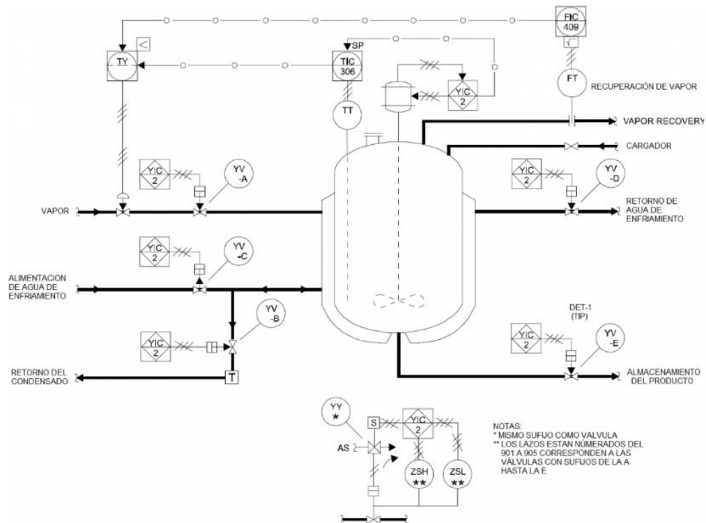
Figura 21. Ejemplo de un P&ID
