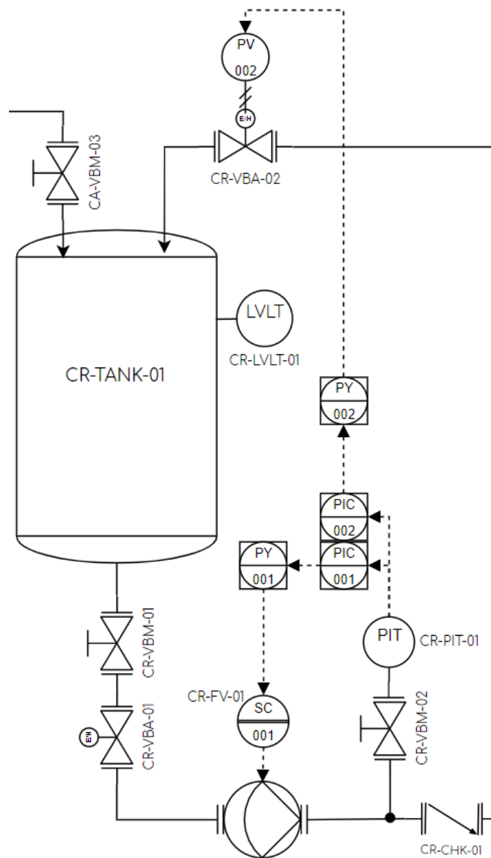
Figura 43. Diagrama P&ID con sistema de control 002
