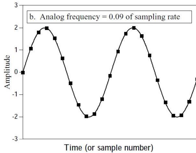
Figura 2. Muestreo correcto de una señal
