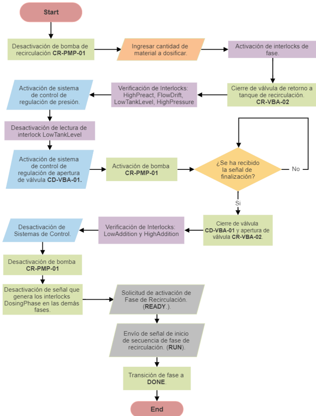
Figura 39. Secuencia de fase de adición
