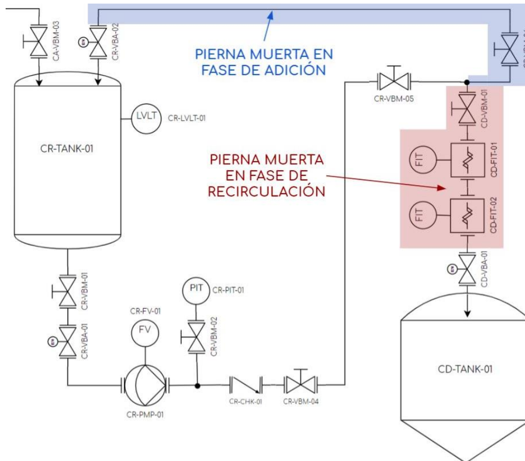
Figura 47. Piernas muertas en sistema de dosificación no sanitario
