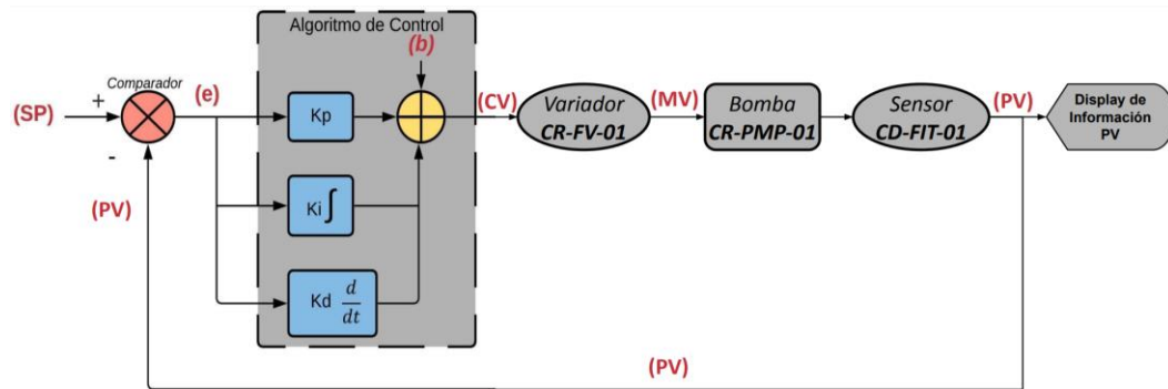
Figura 55. Elementos del sistema de control PID
