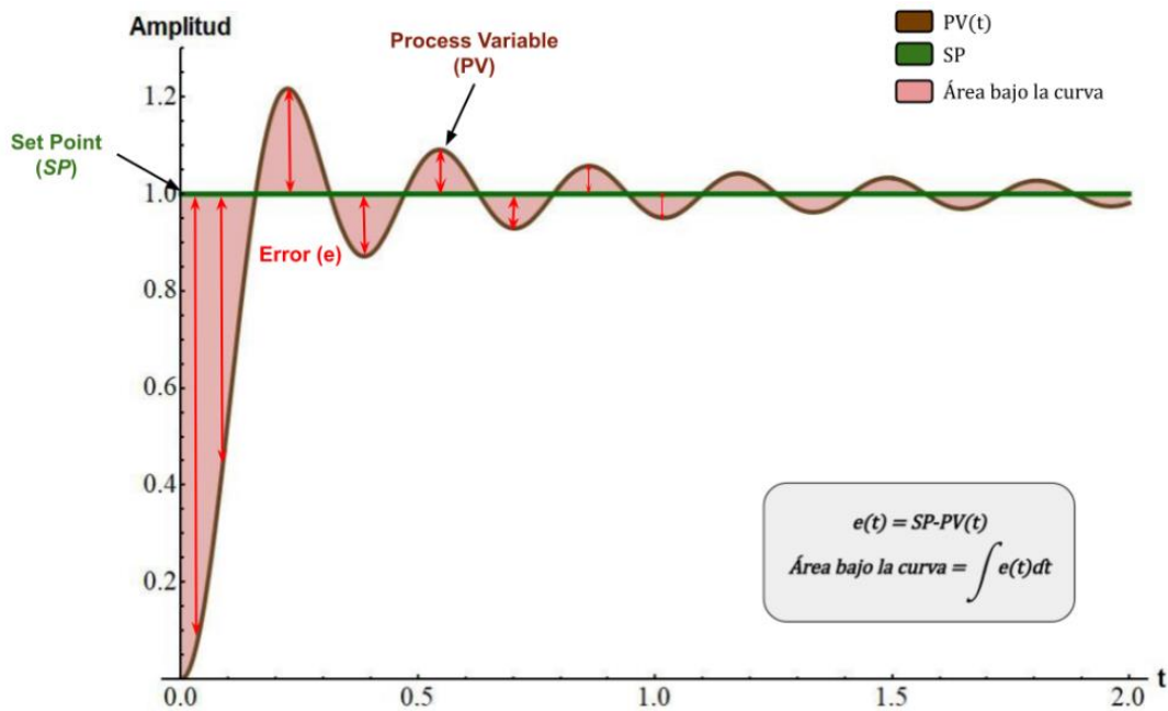
Figura 13. Integración de la señal de error
