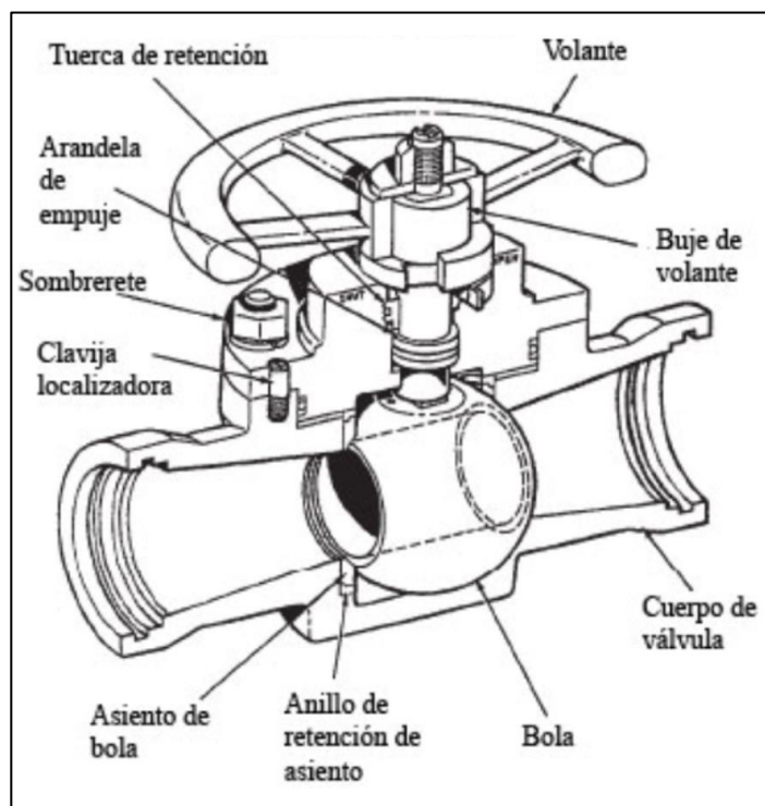
Figura 30. Partes de una válvula de bola
