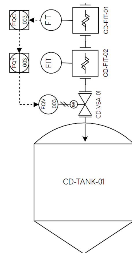
Figura 44. Diagrama P&ID con sistema de control 003
