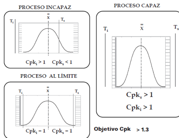
Figura 61. Ejemplo de distribución normal con distintos valores C_{pk}
