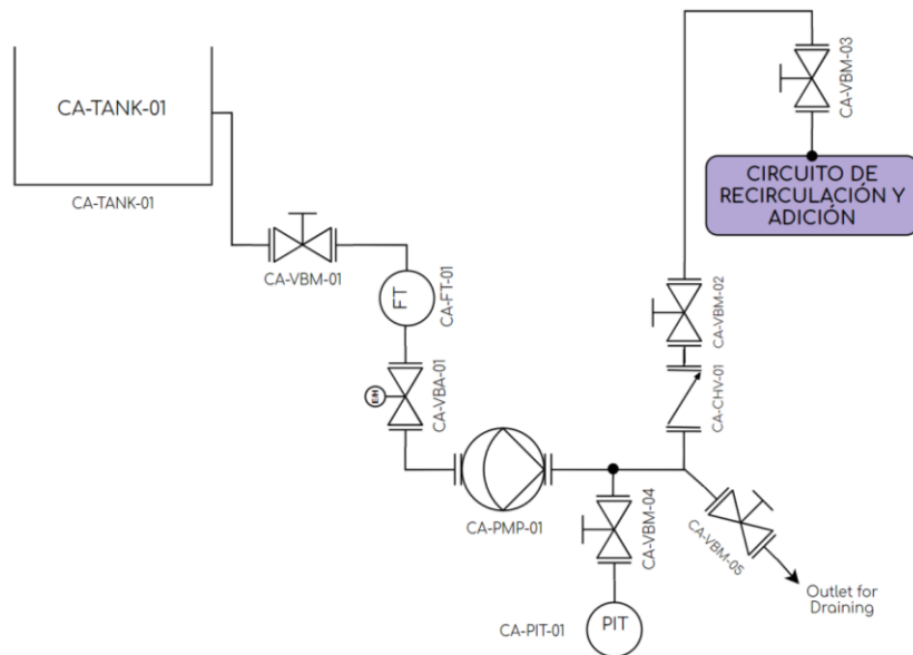
Figura 48. P&ID de circuito de alimentación para sistemas sanitarios
