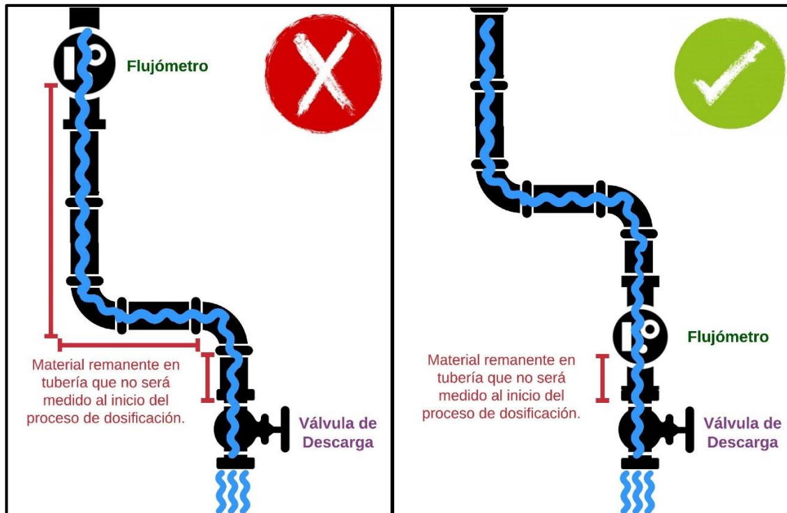
Figura 28. Posición recomendada para flujómetros
