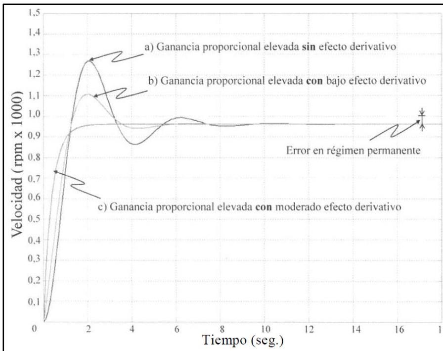
Figura 16. Respuesta de un motor a diferentes ganancias ( K_d )
