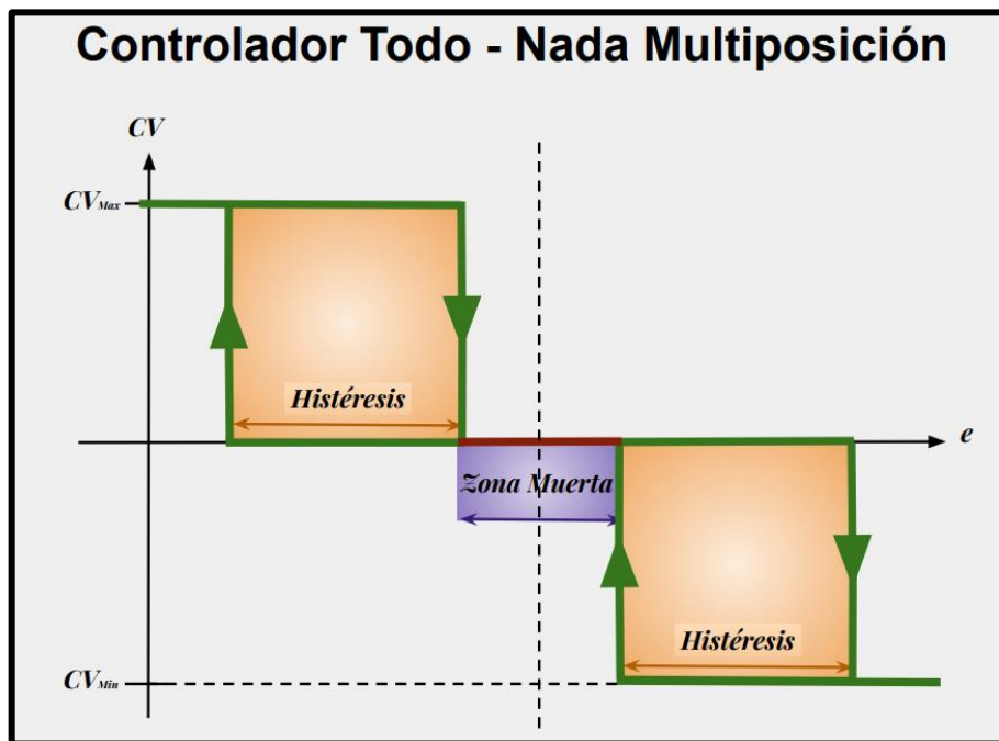
Figura 9. Controlador todo – nada multiposición
