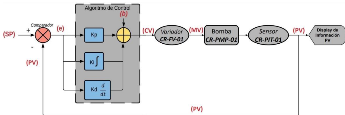
Figura 40. Elementos del sistema de control PID
