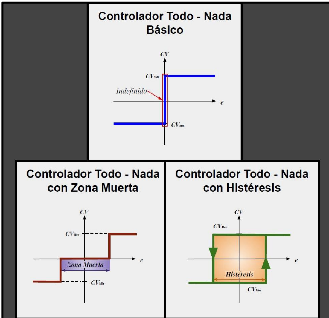
Figura 8. Variantes del controlador todo – nada
