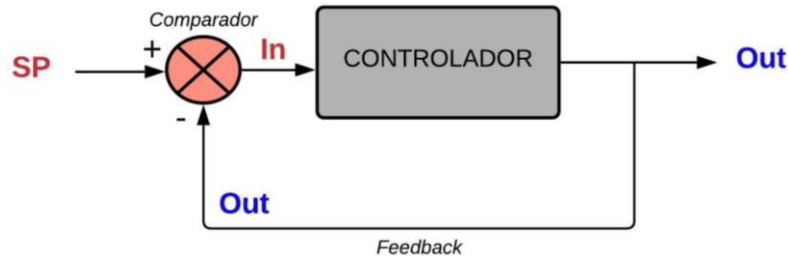
Figura 5. Sistema de control de lazo cerrado
