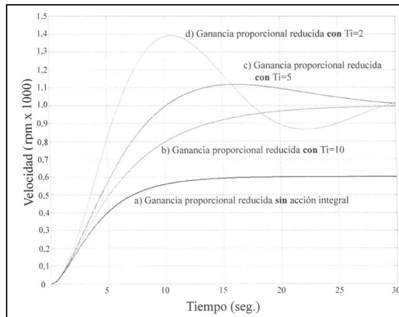
Figura 14. Respuesta de un motor a diferentes ganancias ( K_i )
