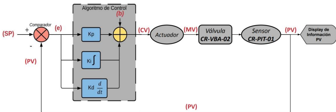
Figura 42. Elementos del sistema de control PID
