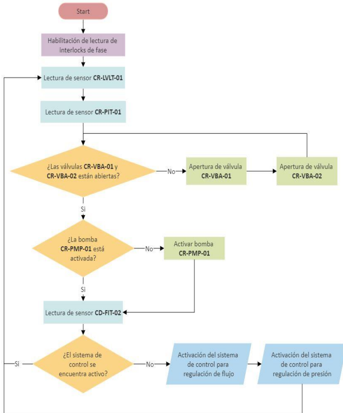
Figura 51. Secuencia de fase de recirculación
