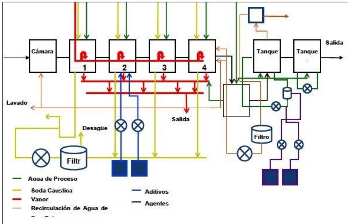
Figura 9. Lavado de botellas
