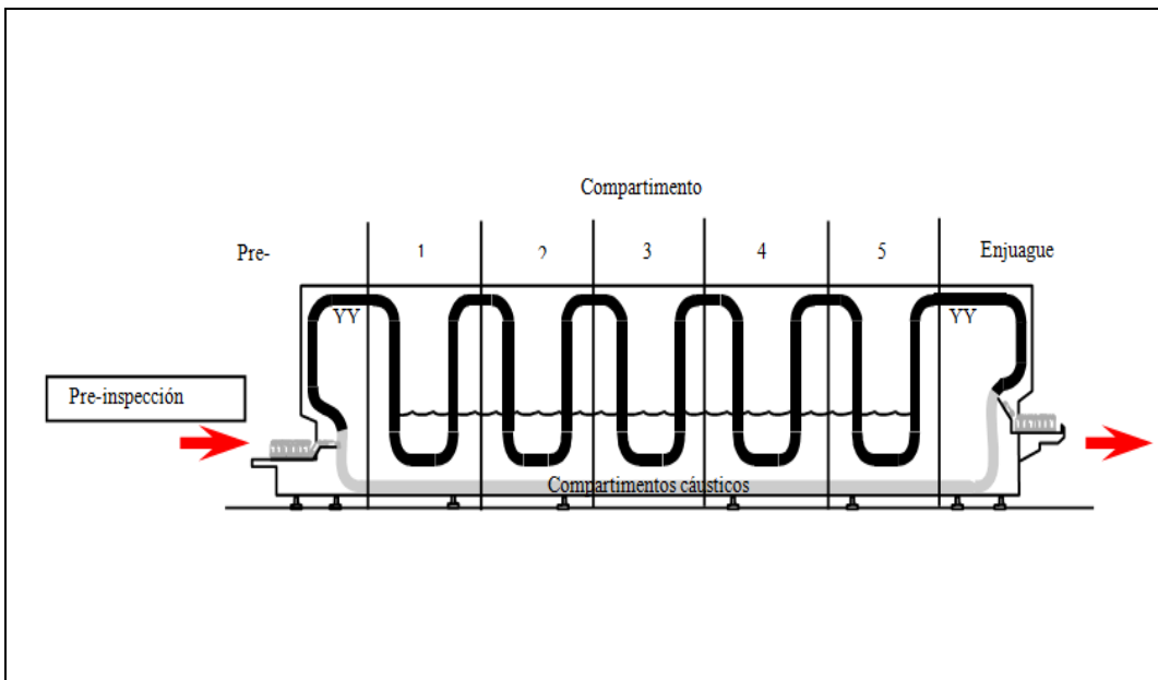
Figura 4. Lavado de botella de vidrio
