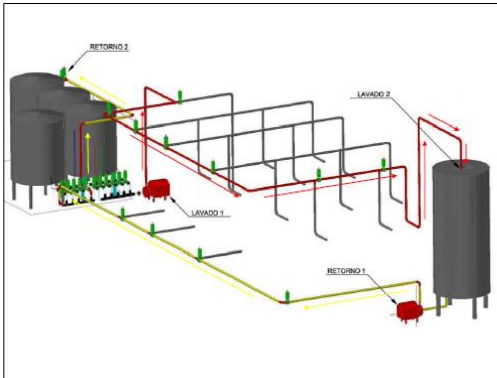
Figura 8. Proceso de sanitizado
