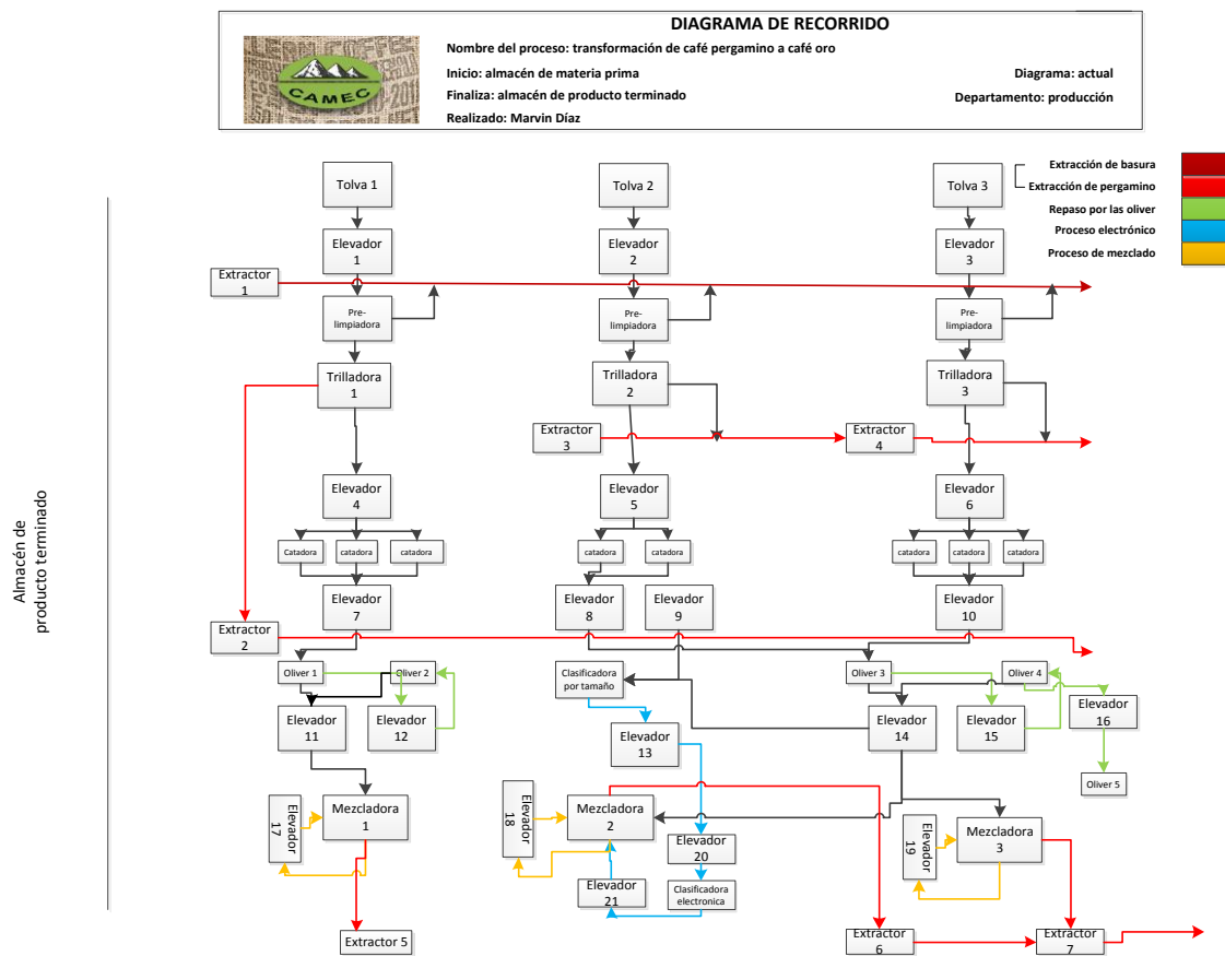
Figura 3. Diagrama de recorrido del proceso
