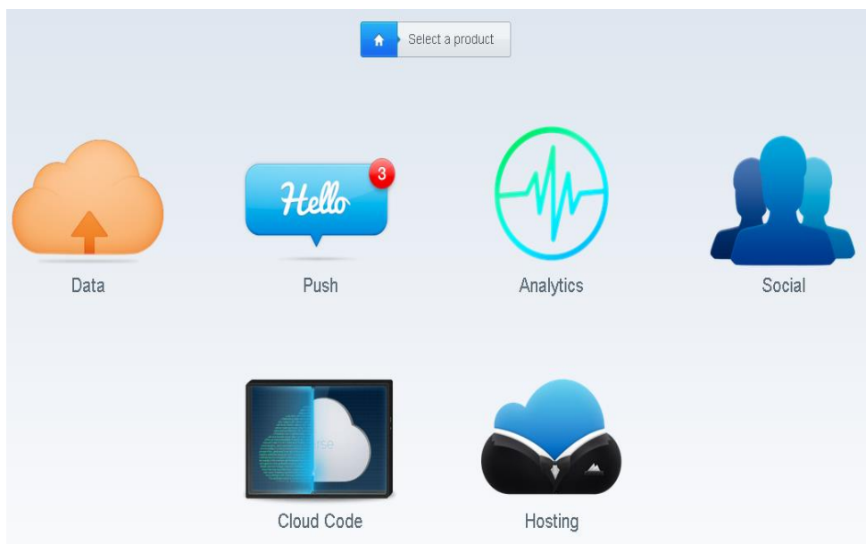
Figura 44. Quickstart Parse
