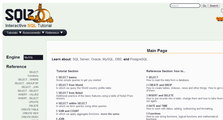
Figura 2. SQLzoo.net inicio
