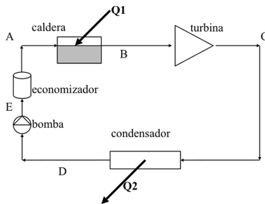
Figura 17. Recuperación de calor con economizador
