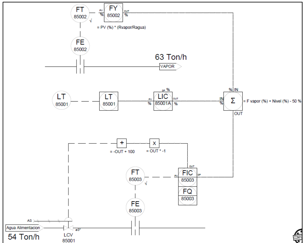
Figura 21. Diagrama PID de proceso para control de tres elementos
