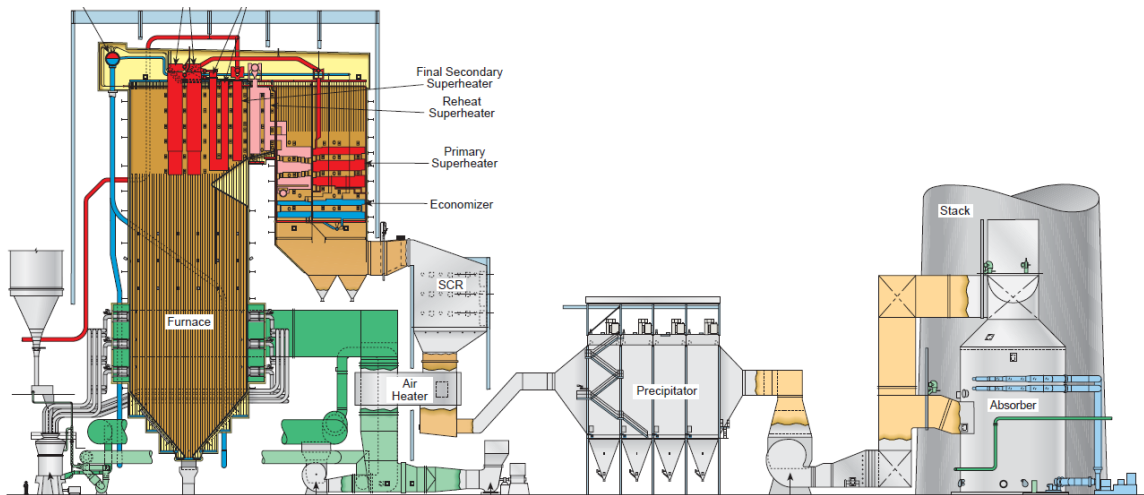
Figura 10. Ciclo completo de una caldera acuotubular
