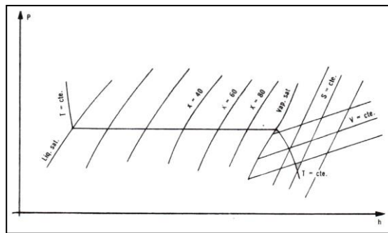
Figura 6. Diagrama presión-entalpia de un refrigerante
