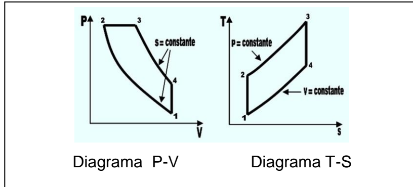
Figura 35. Diagramas ciclo diésel
