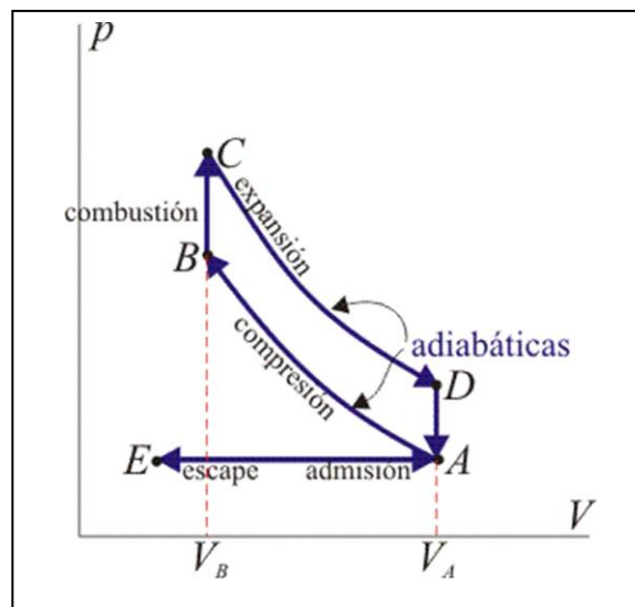
Figura 32. Ciclo Otto
