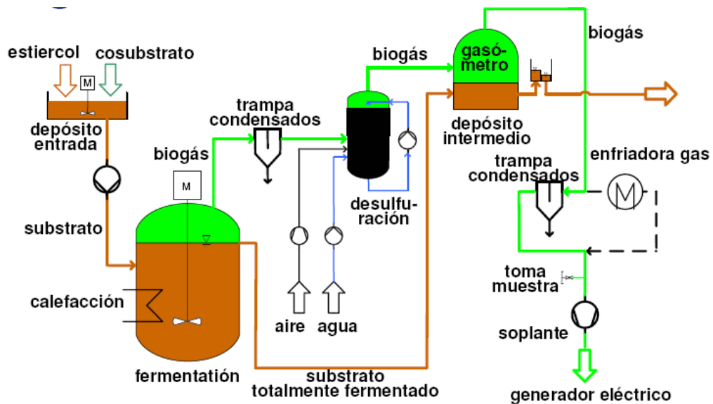
Figura 5. Esquema típico de una planta de biogás
