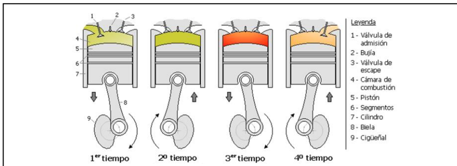
Figura 36. Motores de cuatro tiempos
