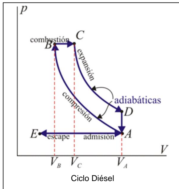
Figura 34. Ciclo diésel
