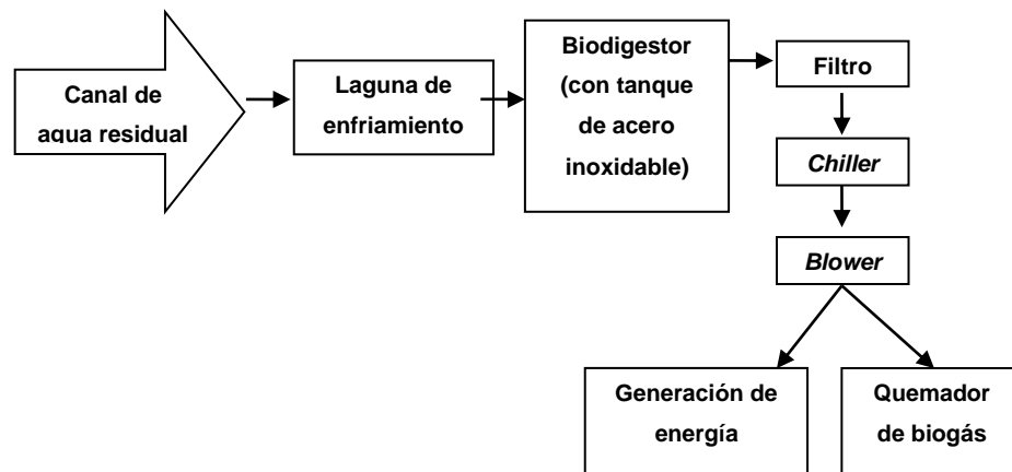
Figura 6. Esquema de planta de biogás en la extractora La Francia
