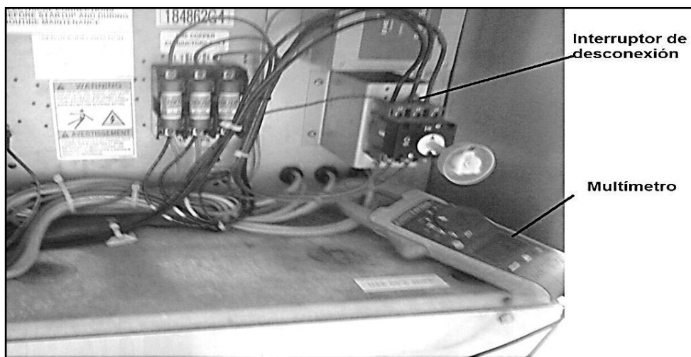
Figura 47. Medición de parámetros eléctricos
