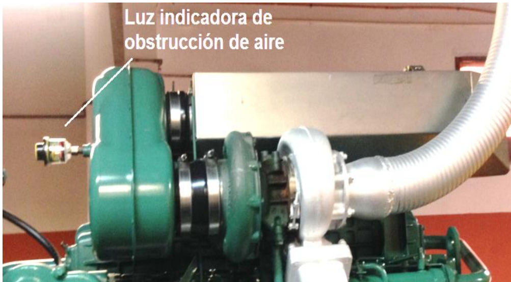
Figura 27. Indicador de obstrucción de aire
