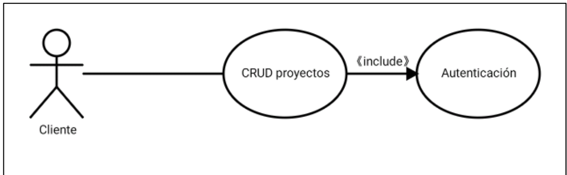
Figura 8. Caso de uso CRUD de proyectos
