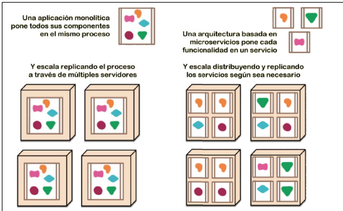
Figura 5. Comparativa entre arquitectura monolítica y microservicios
