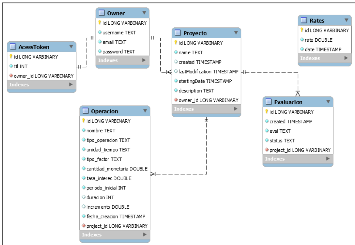
Figura 18. Modelo lógico de datos
