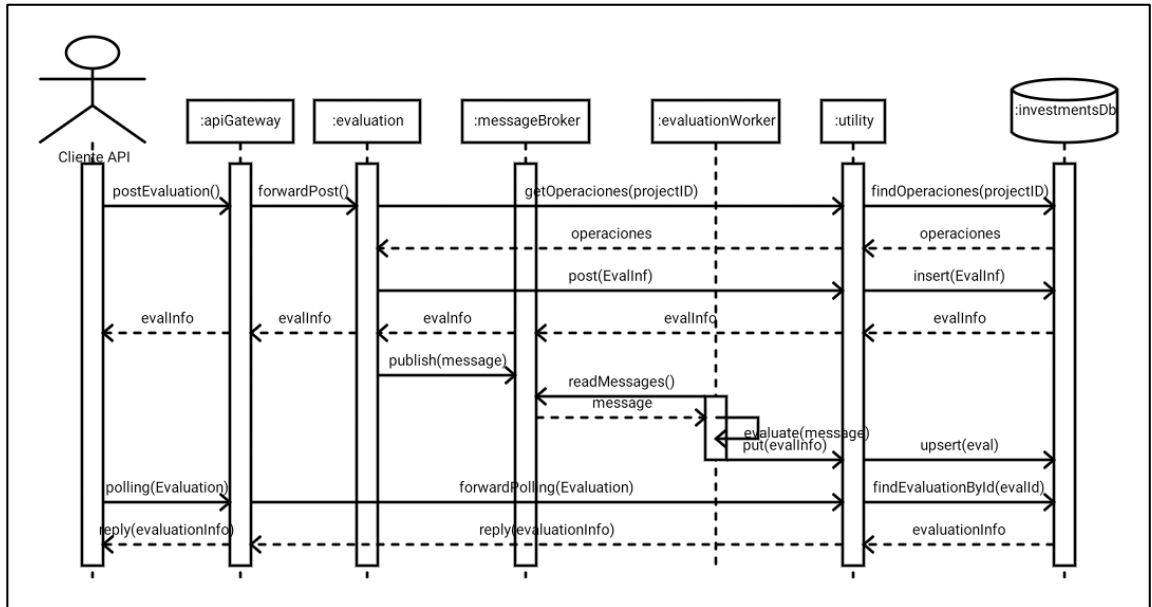
Figura 17. Diagrama de secuencias del proceso de evaluación
