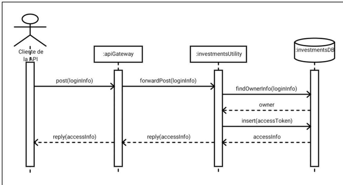
Figura 14. Diagrama de secuencia de autenticación de usuarios
