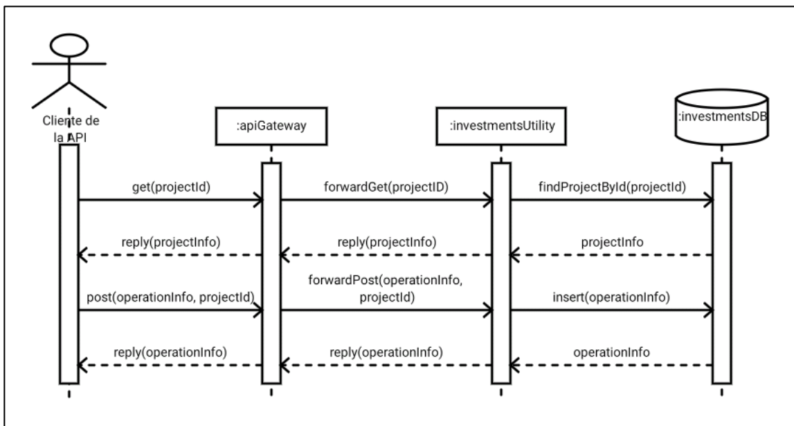
Figura 16. Diagrama de secuencia de creación de nuevas operaciones
