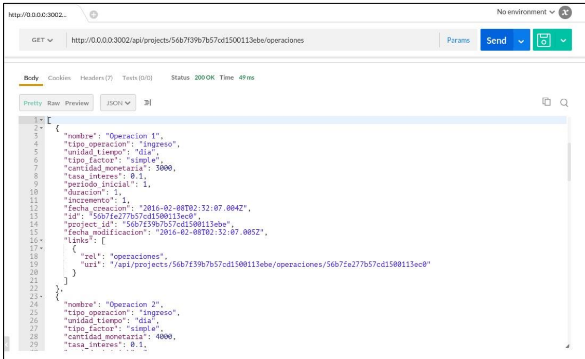
Figura 28. Solicitud GET para obtener una operación
