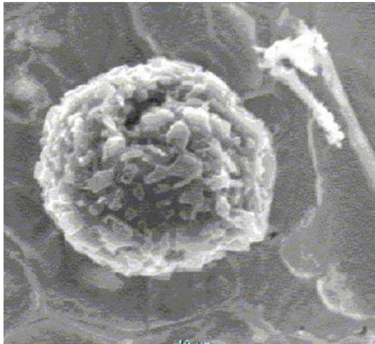
Figura 13. Grafito esferoidal
