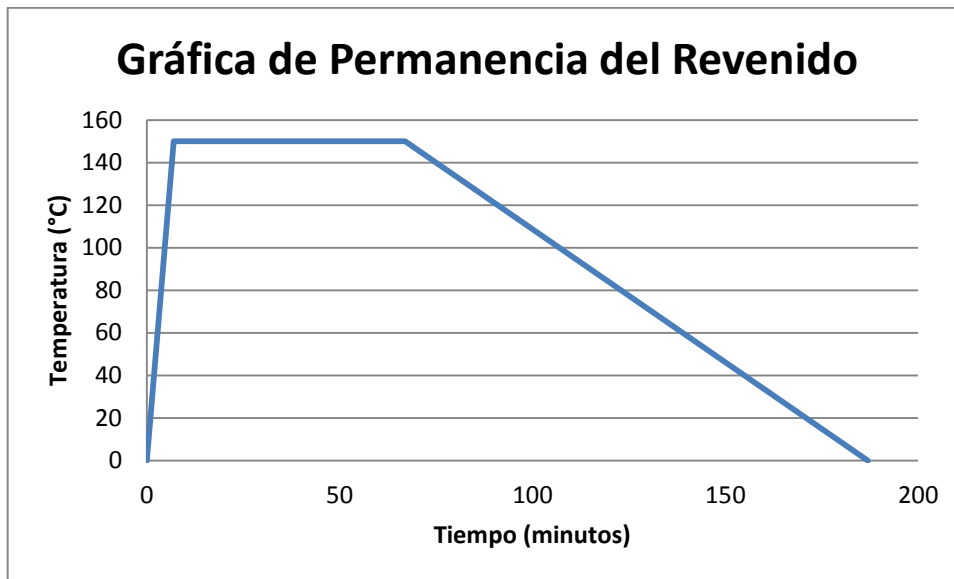
Figura 54. Gráfica de permanencia del revenido
