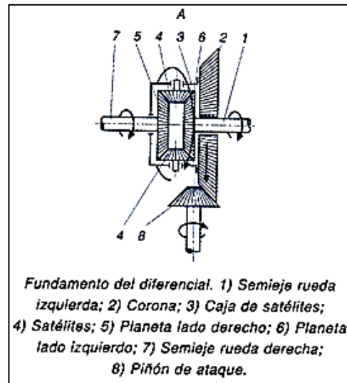
Figura 18. Descripción de piezas del diferencial
