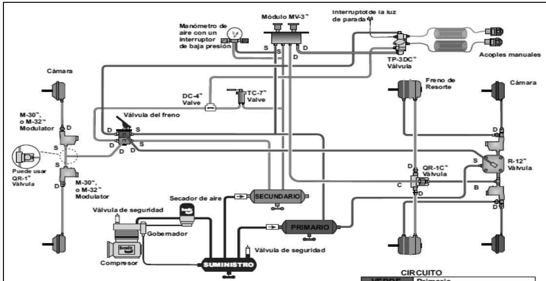
Figura 22. Esquema de circuito de aire
