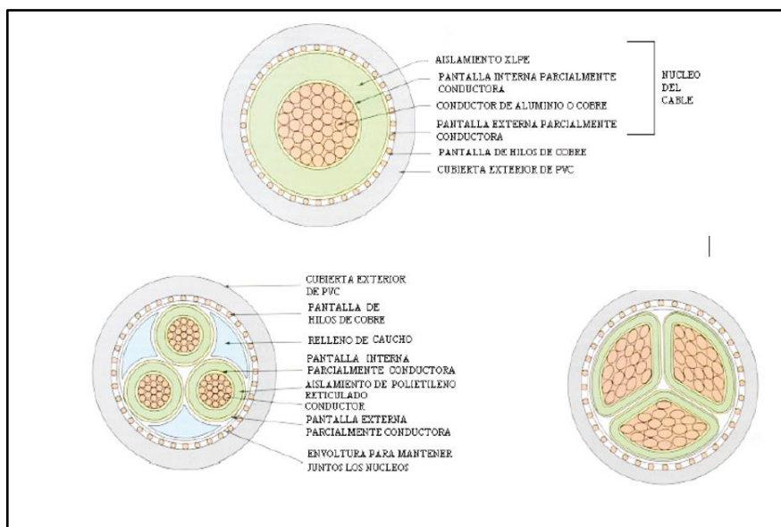
Figura 1. Estructura de cable
