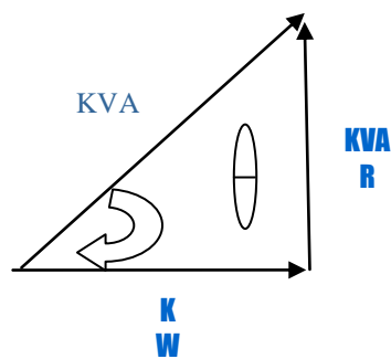
Figura 3. Triángulo de potencias
