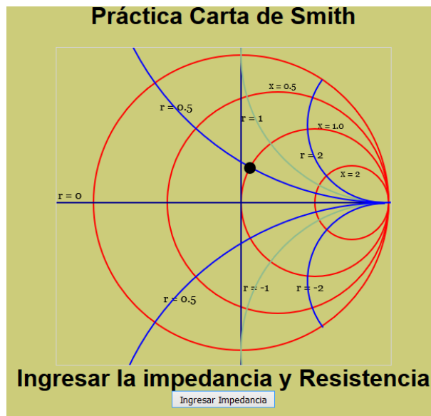
Figura 30. Presentación en la carta de Smith de punto más cercano para los valores ingresados
