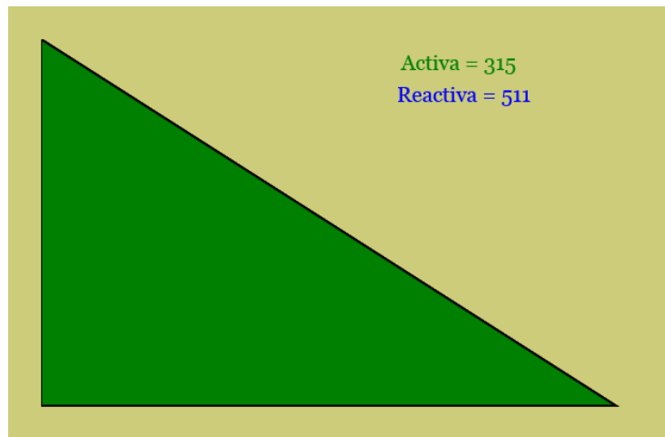
Figura 21. Triángulo de potencias
