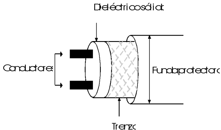
Figura 6. Corte transversal de un conductor
