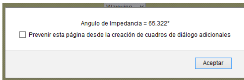
Figura 70. Angulo de la impedancia de línea corta
