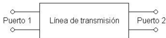
Figura 4. Línea de transmisión (red bipuerto)
