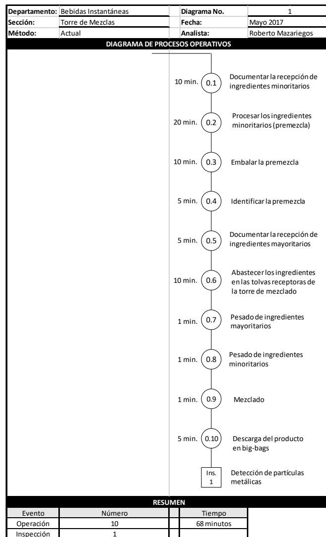
Figura 21. Diagrama de procesos operativos torre de mezcla
