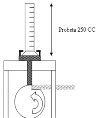
Figura 20. Volumenómetro utilizado para determinar el índice de compresibilidad
