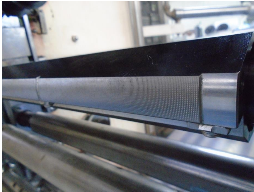
Figura 37. Mordaza termoselladora horizontal
