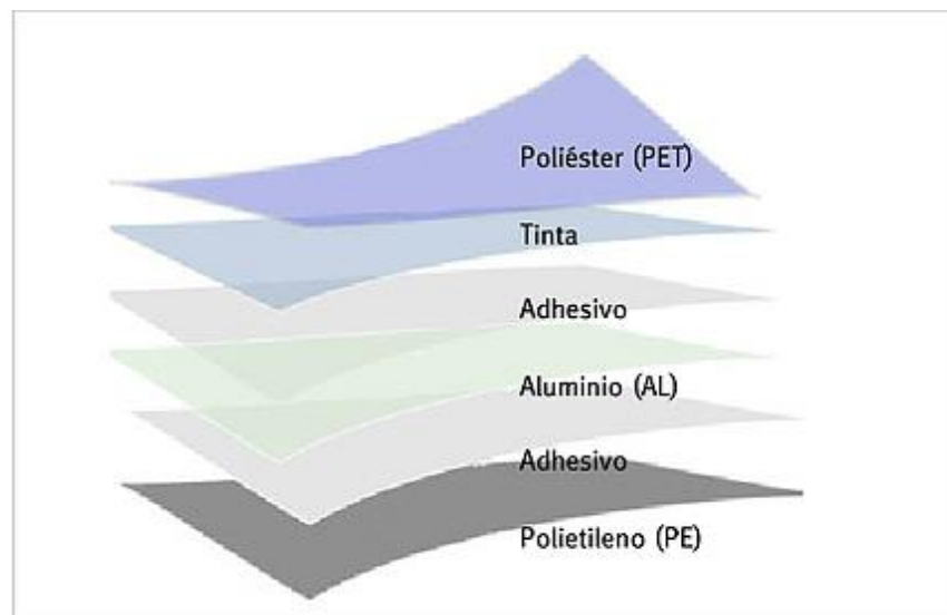
Figura 25. Estructura de una película trilaminada termosellable
