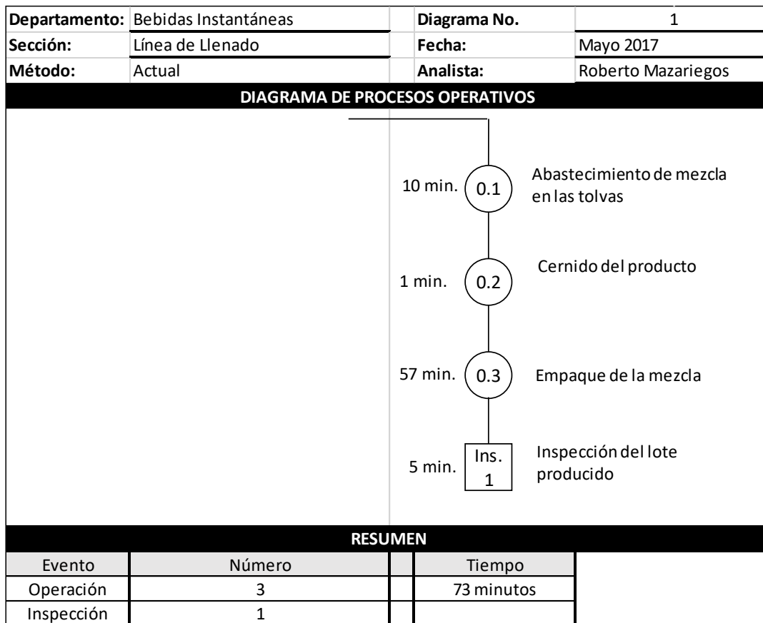
Figura 26. Diagrama de procesos operativos línea de llenado
