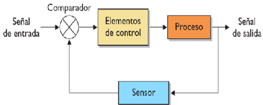
Figura 14. Lazo de control cerrado
