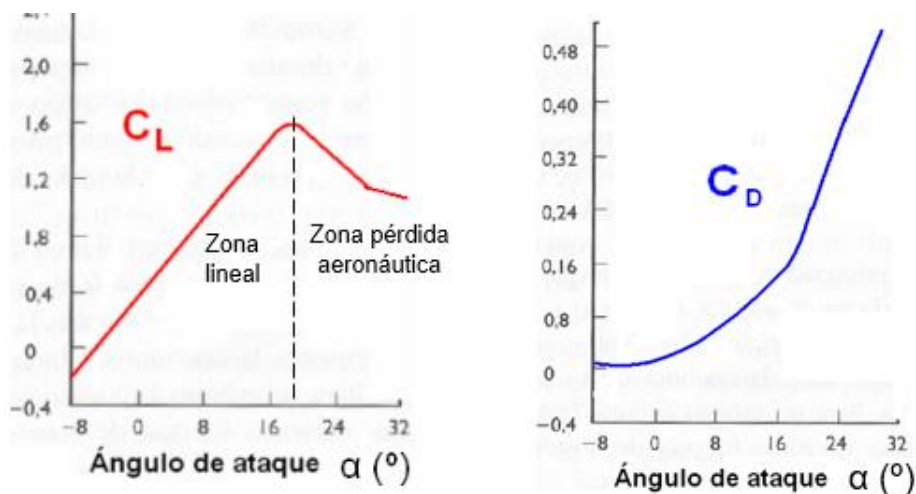
Figura 5. Comportamiento de los coeficientes de sustentación y arrastre
