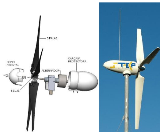
Figura 17. Aerogenerador sotavento
