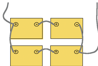
Figura 47. Cableado módulo acumulador
