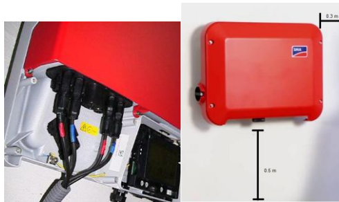
Figura 45. Cableado y distancia mínima rectificador
