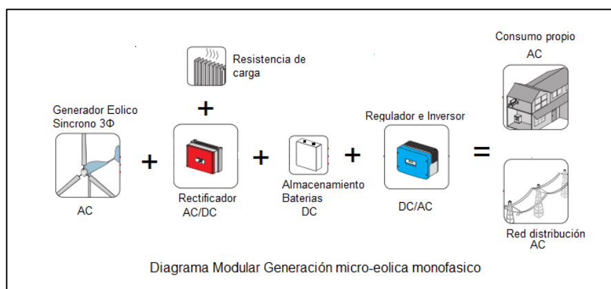
Figura 13. Diagrama monofásico
