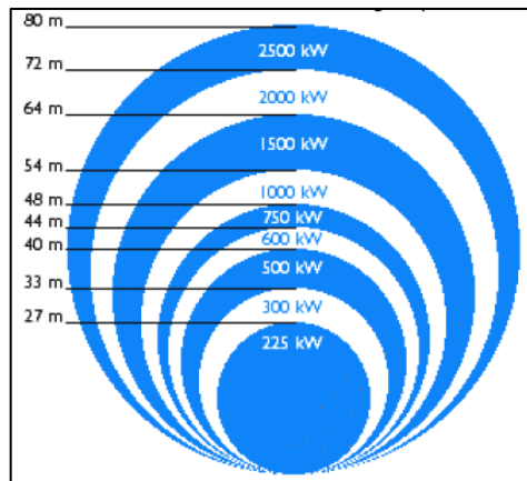
Figura 20. Potencia según diámetro de hélices
