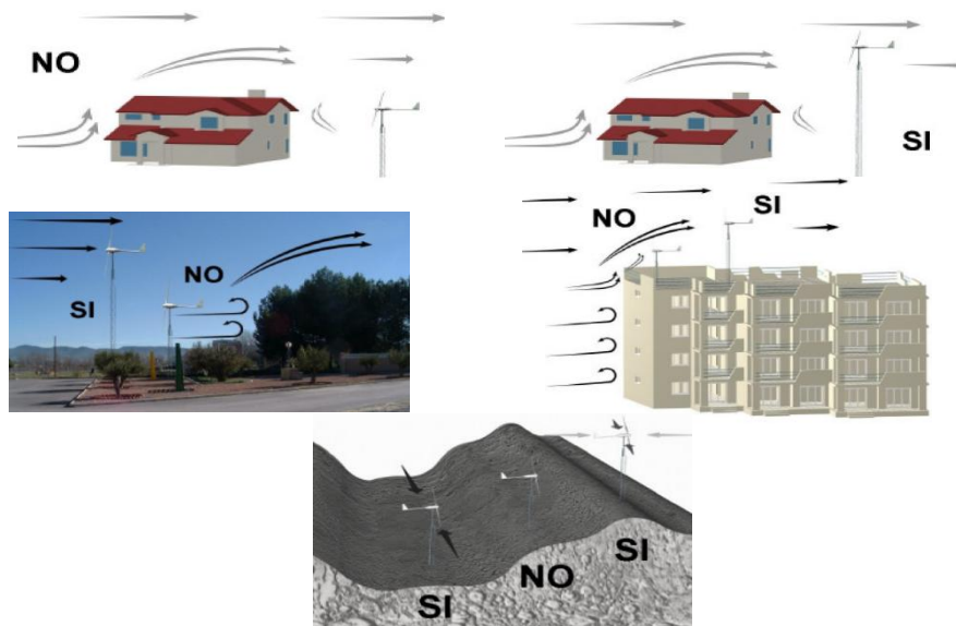
Figura 29. Viento afectado por viviendas y edificios
