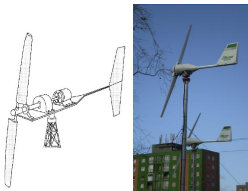
Figura 16. Aerogenerador barlovento
