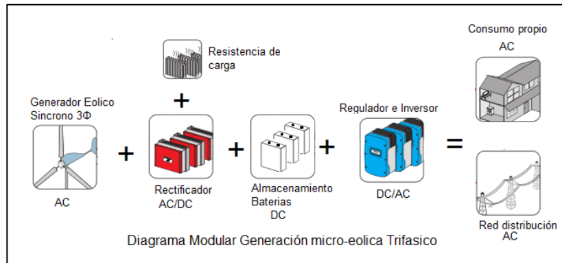
Figura 14. Diagrama modular trifásico
