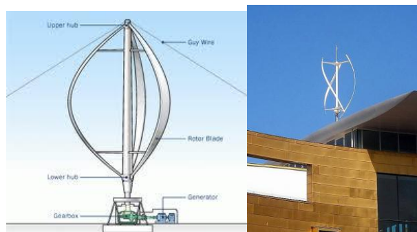
Figura 19. Aerogenerador Diarreus
