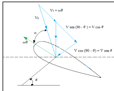
Figura 8. Ángulo variante del flujo de viento respecto a \theta
