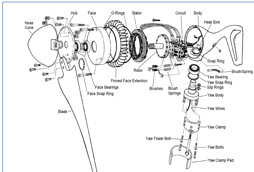
Figura 36. Componentes internos de un generador microeólico
