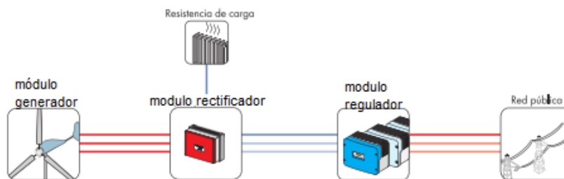
Figura 44. Instalación rectificador
