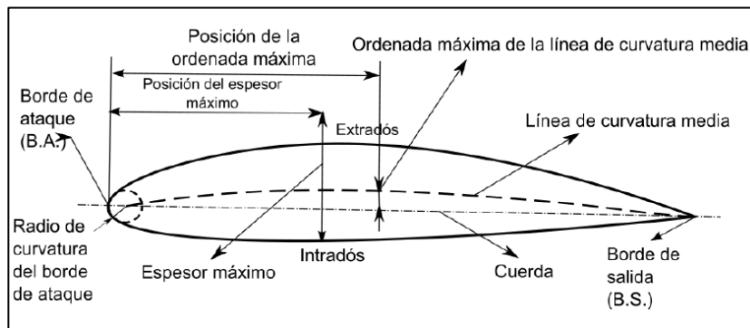
Figura 1. Componentes de un perfil de aspa de un aerogenerador
