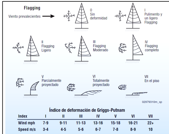
Figura 9. Efecto flagging
