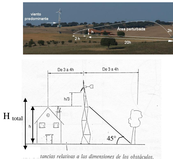
Figura 32. Distancias relativas a las dimensiones de los obstáculos
