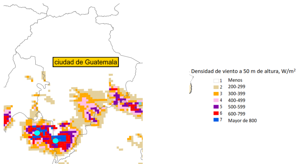
Figura 28. Densidad de viento, región central de Guatemala
