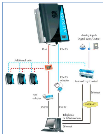
Figura 48. Opciones de transmisión de datos para regulación y control
