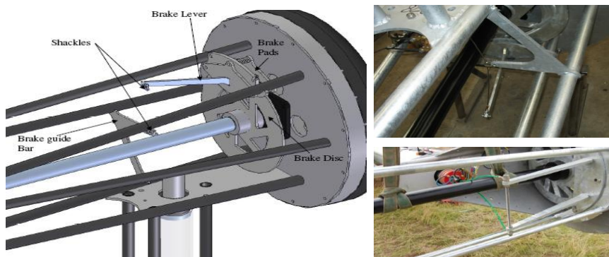
Figura 34. Instalación de frenos mecánicos
