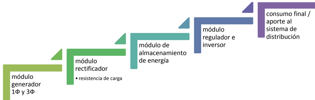
Figura 12. Módulos que conforman una instalación microeólica
