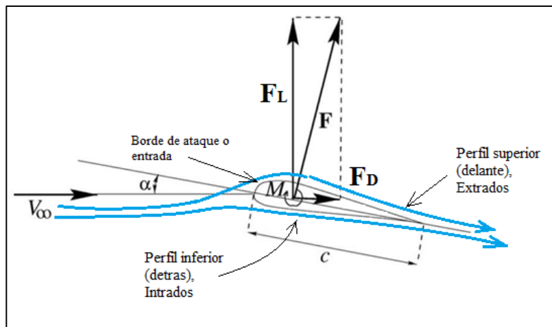
Figura 2. Fuerzas que actúan sobre un aspa de un aerogenerador
