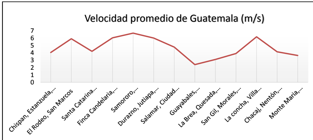
Figura 11. Gráfica de velocidad promedio en Guatemala
