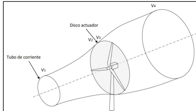
Figura 6. Esquema de aerogenerador según modelo de disco actuador
