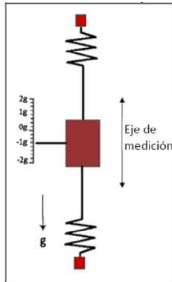
Figura 8. Diagrama de sistema MEMS para medición de aceleración
