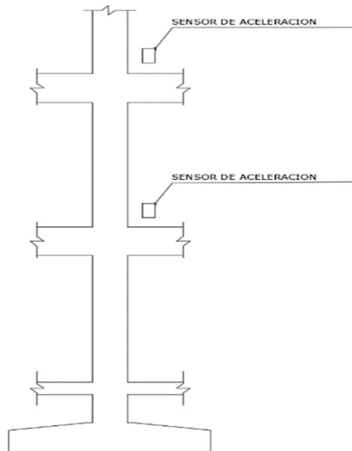
Figura 14. Colocación de sensores en la estructura
