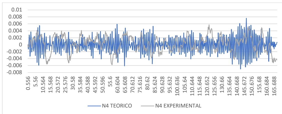
Figura 48. Aceleraciones nivel 4
