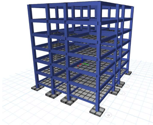
Figura 19. Modelo de edificio en programa de análisis estructural
