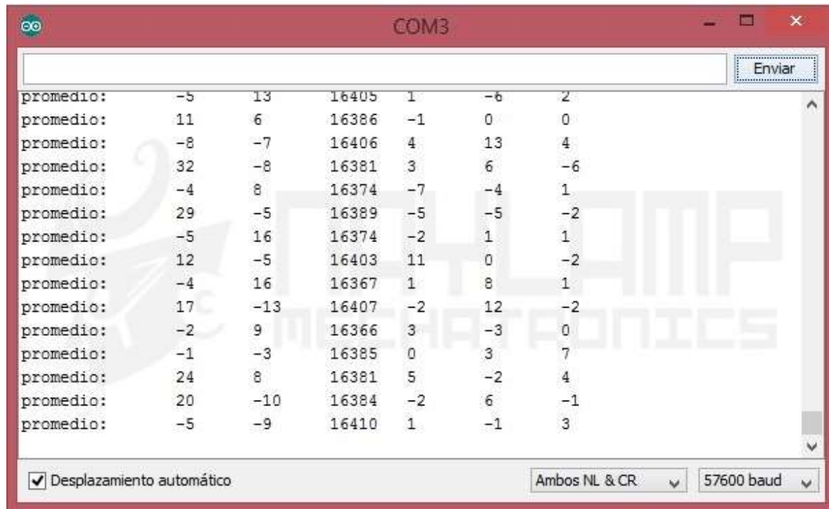
Figura 40. Monitor serial de calibración del sensor
