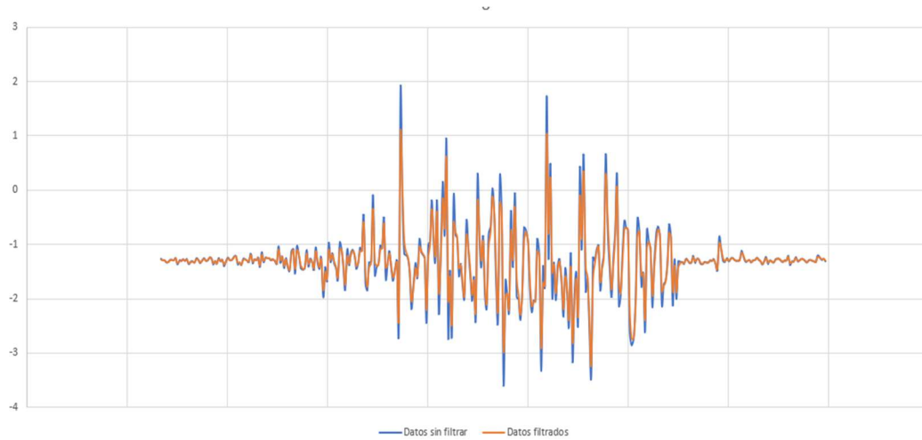
Figura 10. Datos filtrados con una constante de 0.80
