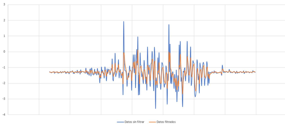
Figura 11. Datos filtrados con una constante de 0.50
