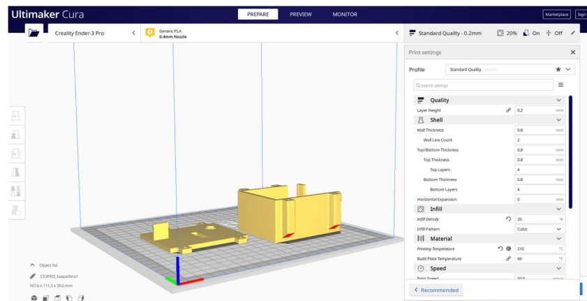
Figura 31. Configuraciones de impresión 3D de la caja
