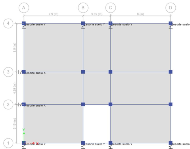
Figura 18. Asignación de resortes de confinamiento de suelo
