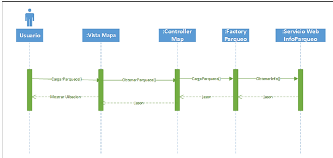
Figura 46. Diagrama de secuencia: obtener información de parques
