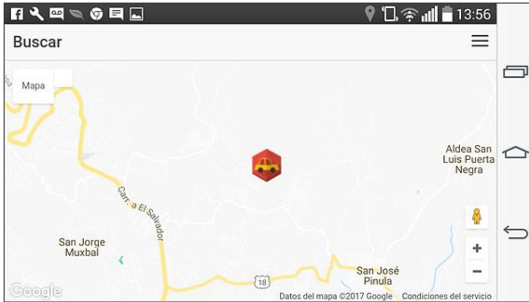
Figura 51. Interfaz Pfinder
