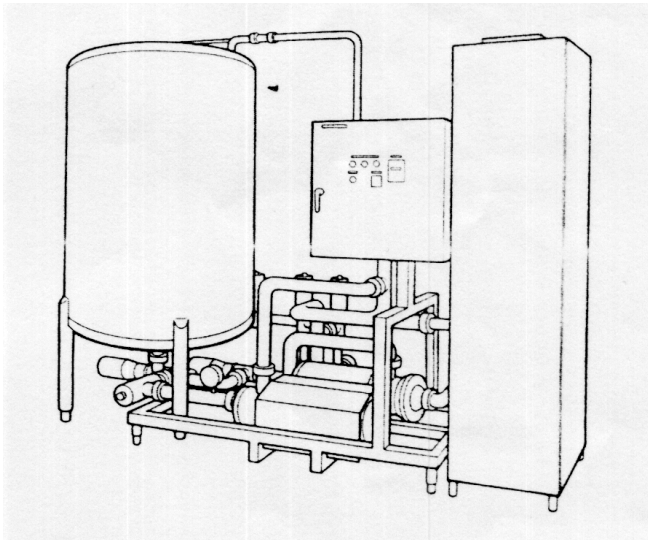
Figura 4. Unidad CIP correspondiente a un sistema descentralizado de limpieza
