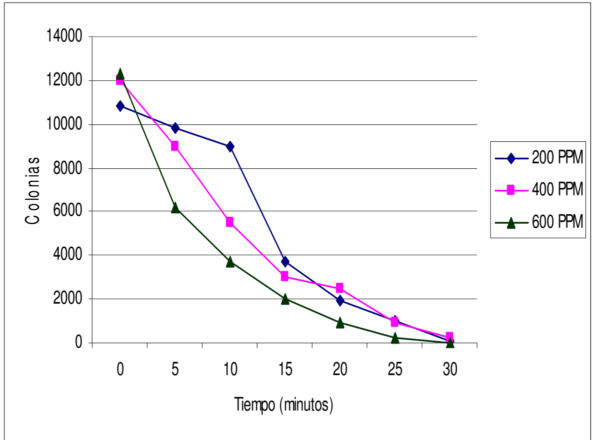
Figura 6. Gráfico que muestra la curva de muerte de bacterias en función del tiempo para el sanitizante: Amonio Cuaternario
