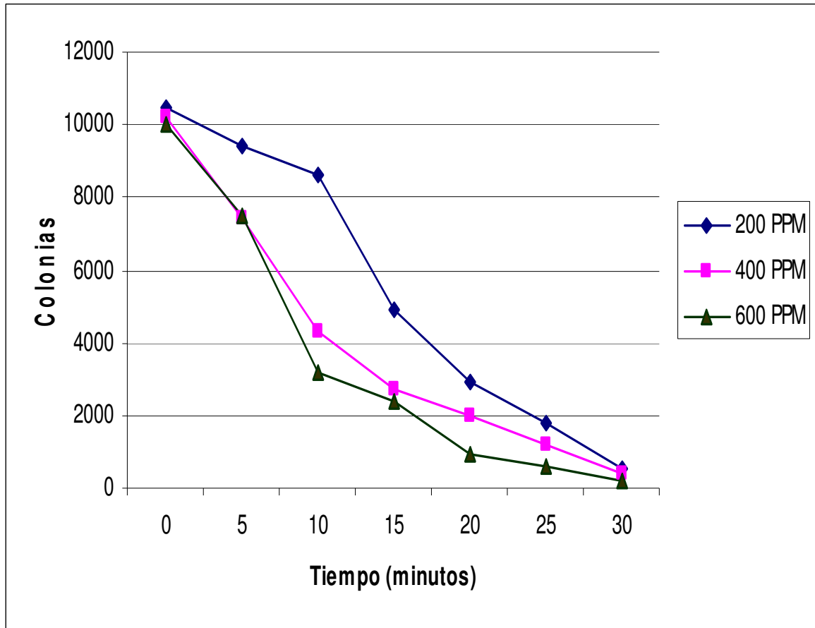
Figura 7. Gráfico de muestra la curva de muerte de bacterias en función del tiempo para el sanitizante: Hipoclorito de Sodio
