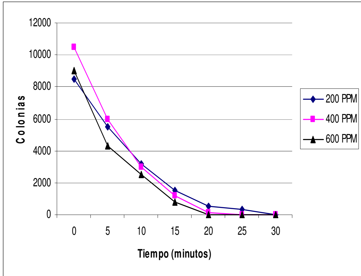
Figura 8. Gráfico que muestra la curva de muerte de bacterias en función del tiempo para el sanitizante: Yodo Polimérico
