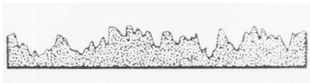
Figura 1. Vista microscópica de la superficie de una tubería de acero inoxidable (Aumento: Horizontal*100, Vertical * 1000)
