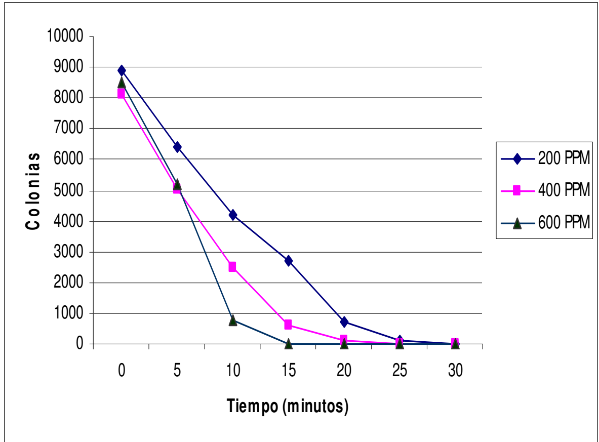
Figura 5. Gráfico que muestra la curva de muerte de bacterias en función del tiempo para el sanitizante: Ácido Peroxacético
