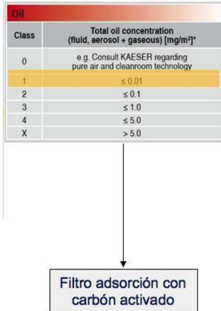
Figura 19. Selección del filtro de aceite
