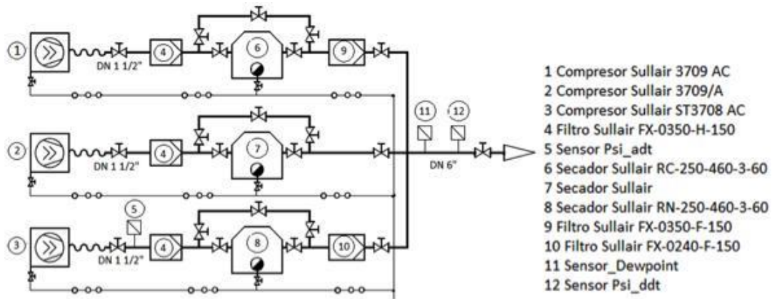
Figura 2. Diagrama del sistema
