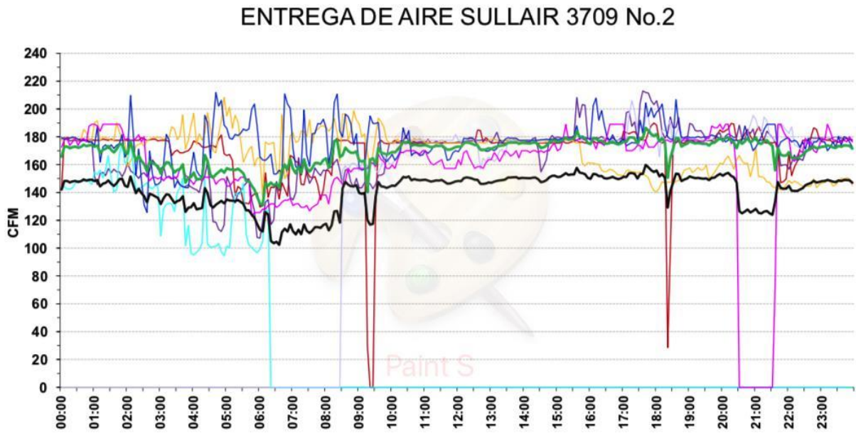
Figura 11. Caudal compresor No.2
