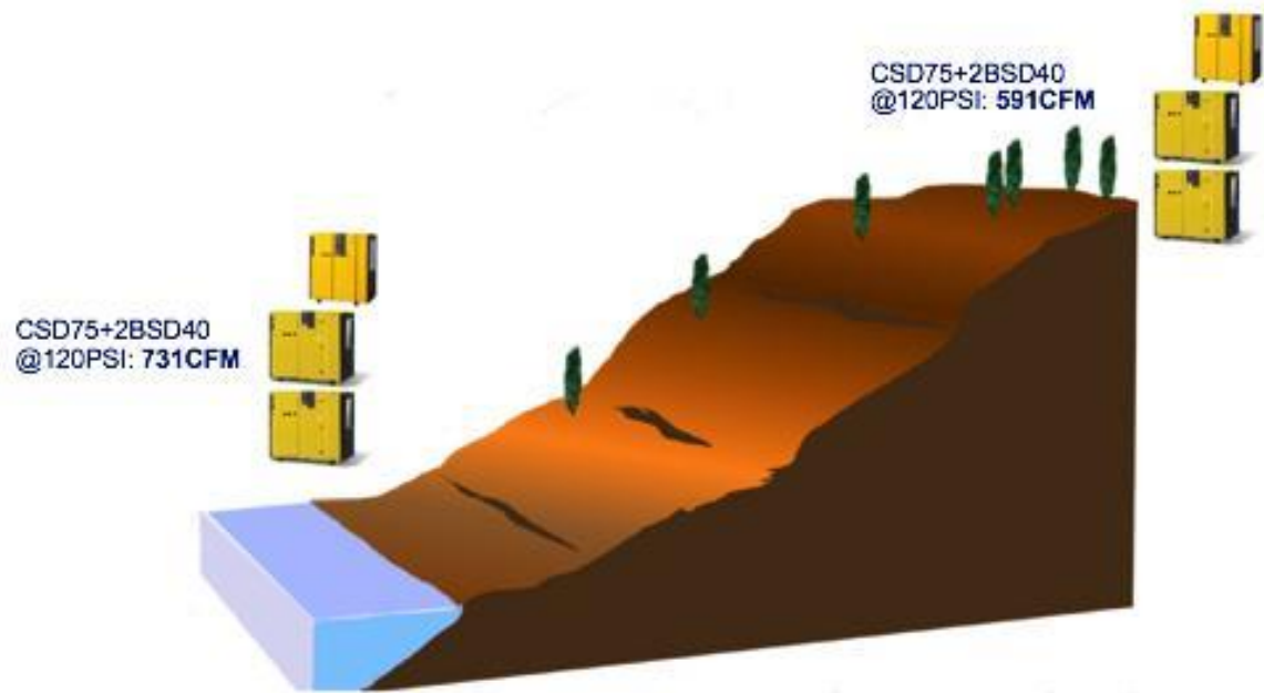
Figura 3. Ejemplo de pérdidas por altura
