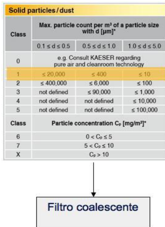
Figura 17. Selección del filtro de partículas
