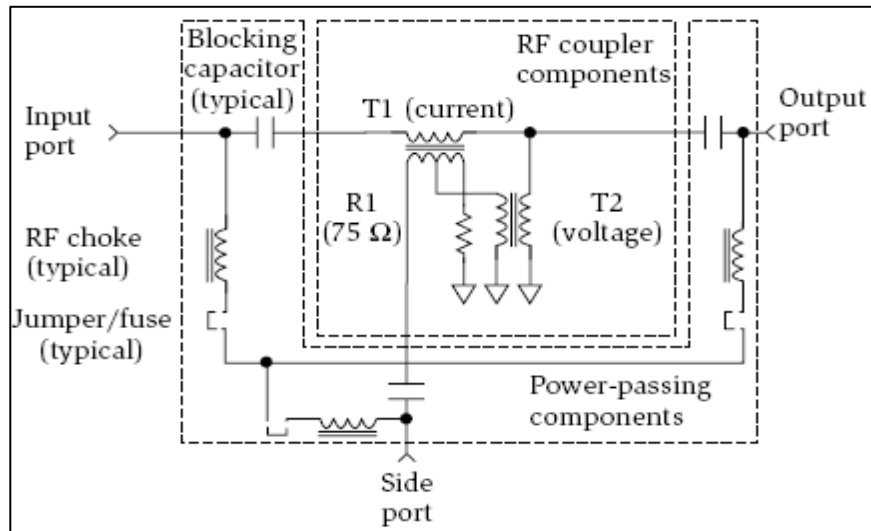
Figura 8. Diagrama de bloques de una copla direccional
