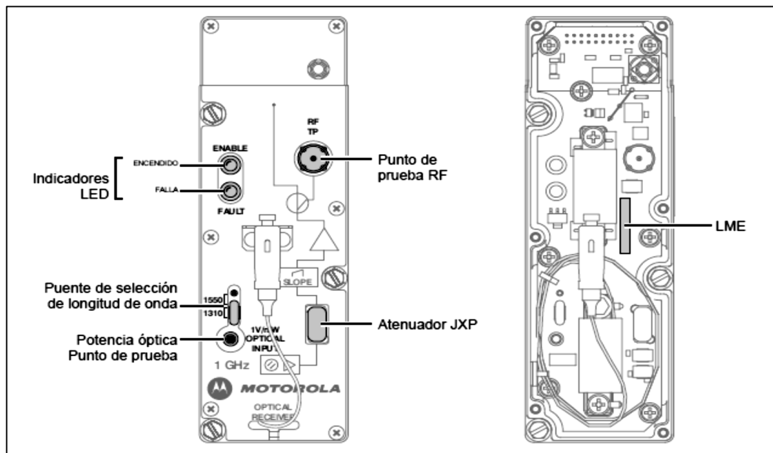
Figura 5. Tarjeta o módulos ópticos real: (a) receptor, (b) transmisor
