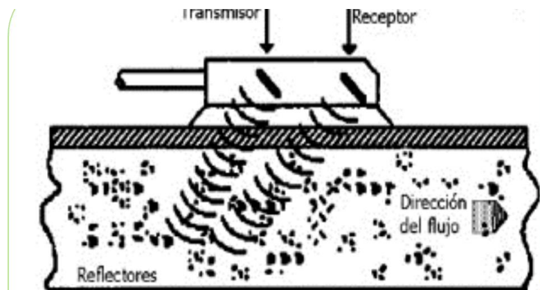
Figura 9. Medidor de caudal ultrasónico
