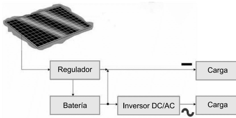
Figura 11. Sistema solar fotovoltaico aislado
