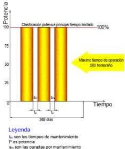
Figura 4. Potencia principal por tiempo limitado (LTP)
