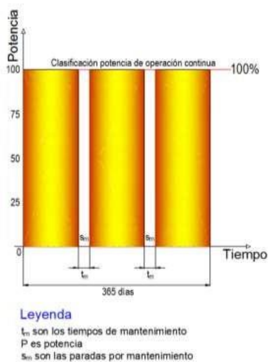
Figura 6. potencia operativa continua (COP)
