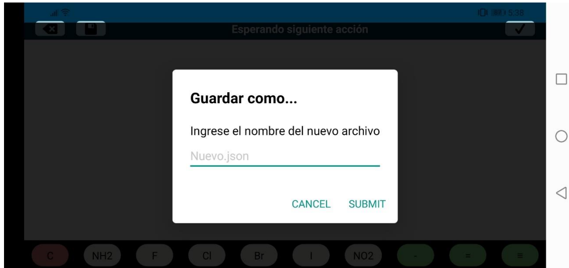
Figura 31. Cuadro de diálogo “Guardar como...”, Lienzo
