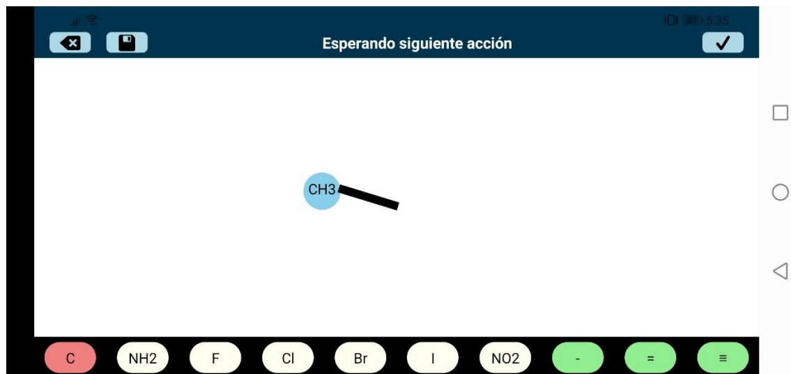
Figura 21. Inserción de nuevo enlace simple, Lienzo
