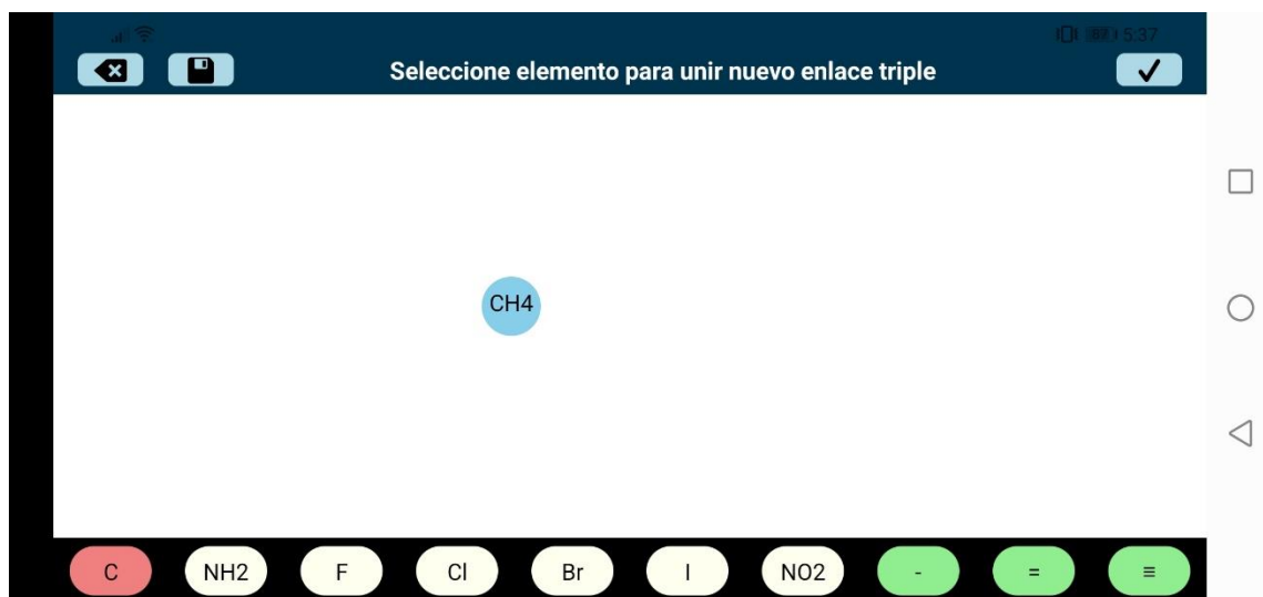
Figura 24. Nuevo enlace triple, Lienzo
