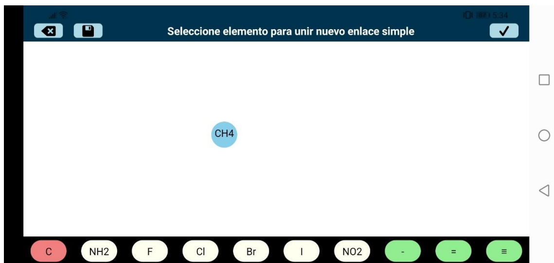
Figura 20. Nuevo enlace simple, Lienzo
