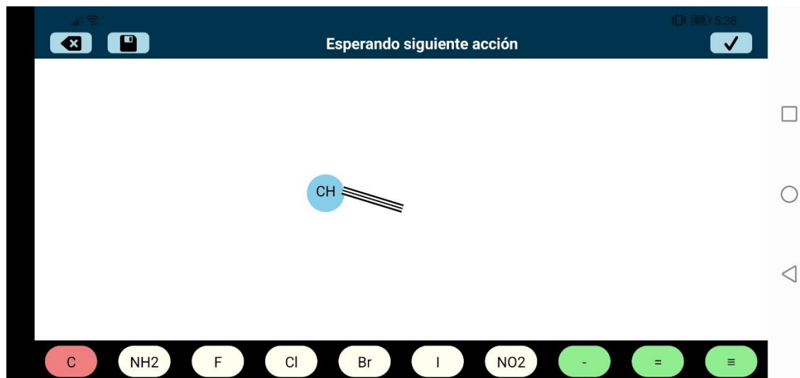
Figura 25. Inserción de nuevo enlace triple, Lienzo
