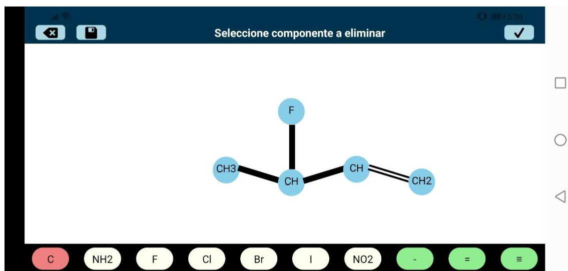
Figura 29. Componente para eliminar, Lienzo
