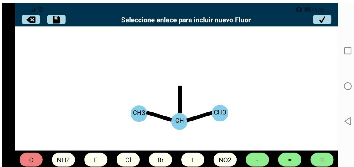
Figura 26. Nuevo elemento Flúor, Lienzo
