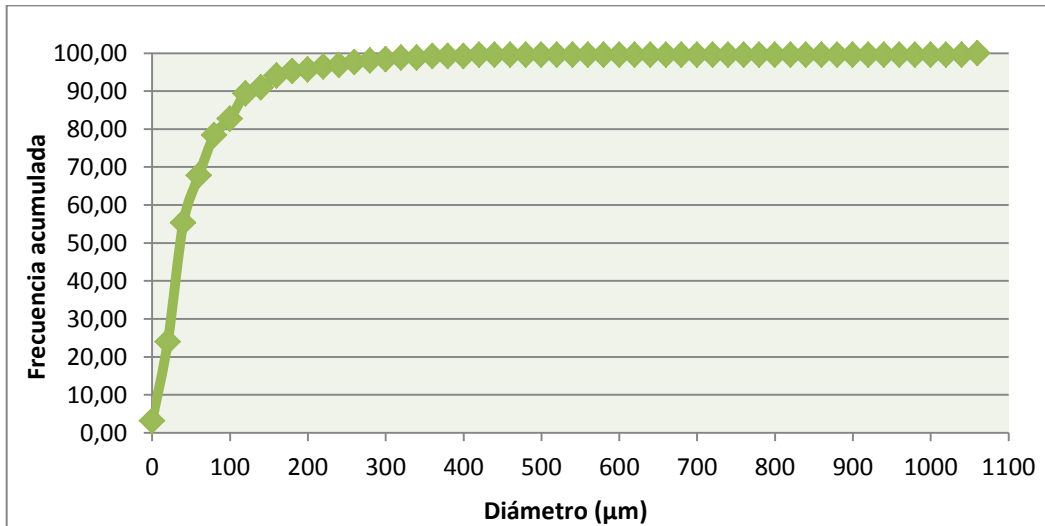
Figura 50. Frecuencia acumulada de diámetro de poro para la membrana 3 A, parte inferior
