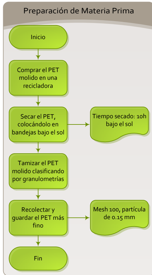
Apéndice 1. Diagrama de flujo de la preparación de materia prima
