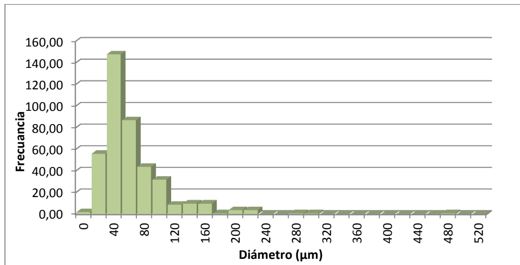
Figura 43. Histograma de frecuencia de diámetro de poro para la membrana 4 A, parte inferior
