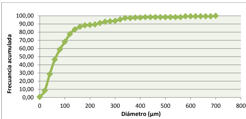
Figura 48. Frecuencia acumulada de diámetro de poro para la membrana 1 A, parte inferior
