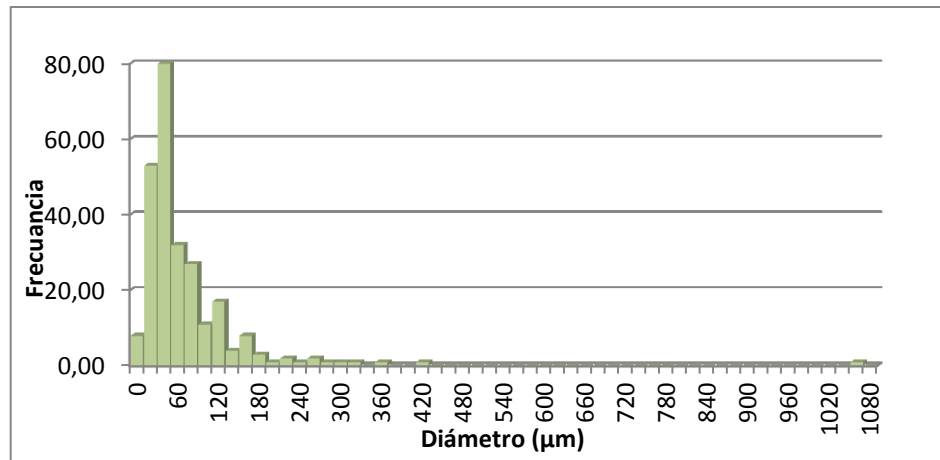
Figura 42. Histograma de frecuencia de diámetro de poro para la membrana 3 A, parte inferior
