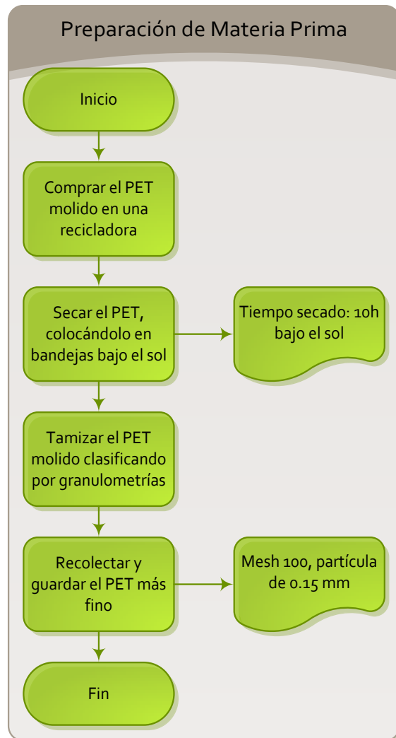
Figura 11. Diagrama de flujo de procedimiento para preparar la materia prima
