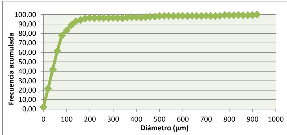
Figura 49. Frecuencia acumulada de diámetro de poro para la membrana 2 A, parte inferior
