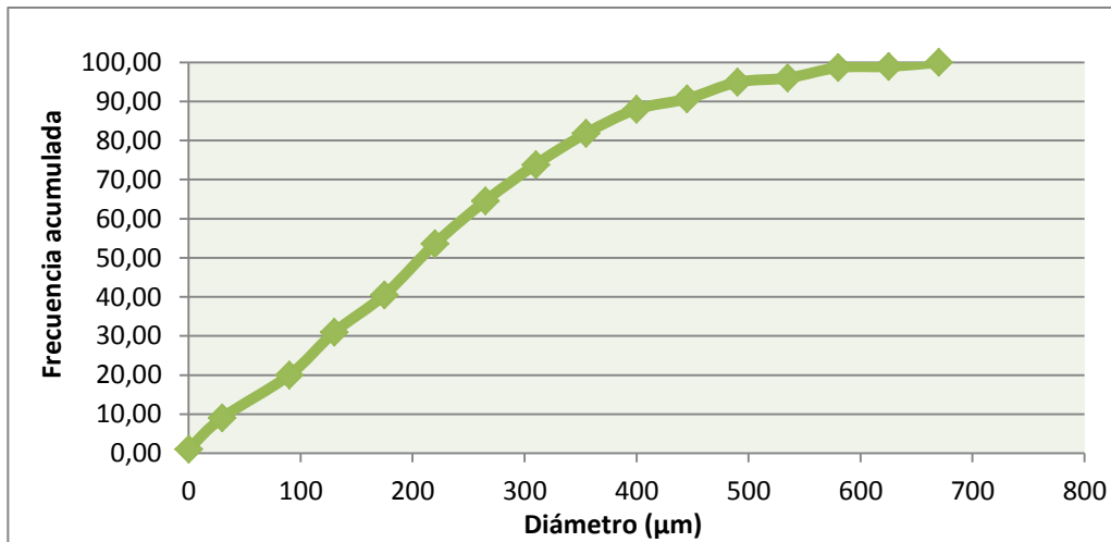
Figura 47. Frecuencia acumulada de diámetro de poro para la membrana 4 A, parte superior
