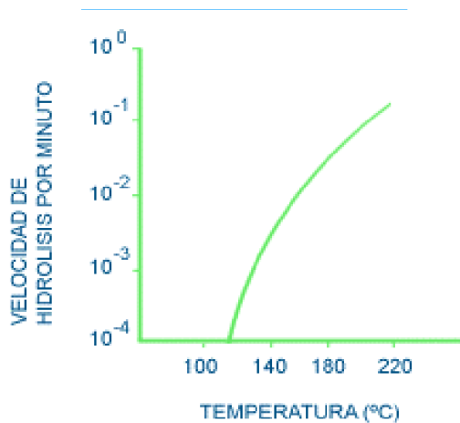
Figura 5. Hidrólisis del PET
