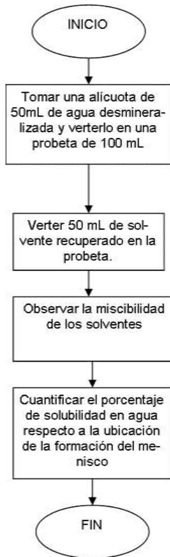
Figura 7. Diagrama para la determinación del porcentaje de solubilidad en agua de los solventes recuperados
