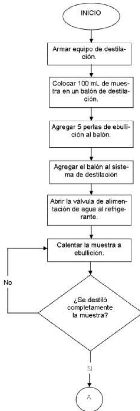
Figura 3. Diagrama del procedimiento experimental para la destilación de solvente
