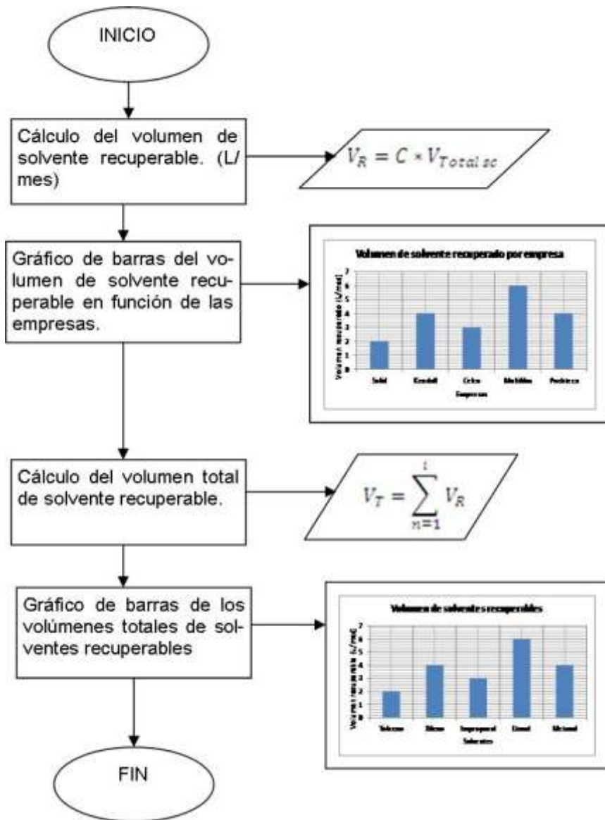
Figura 2. Diagrama de cálculo de la cantidad de solvente recuperable
