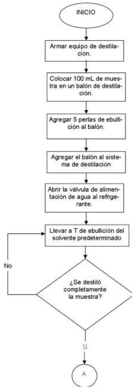
Figura 5. Diagrama para la determinación de la pureza los solventes recuperados
