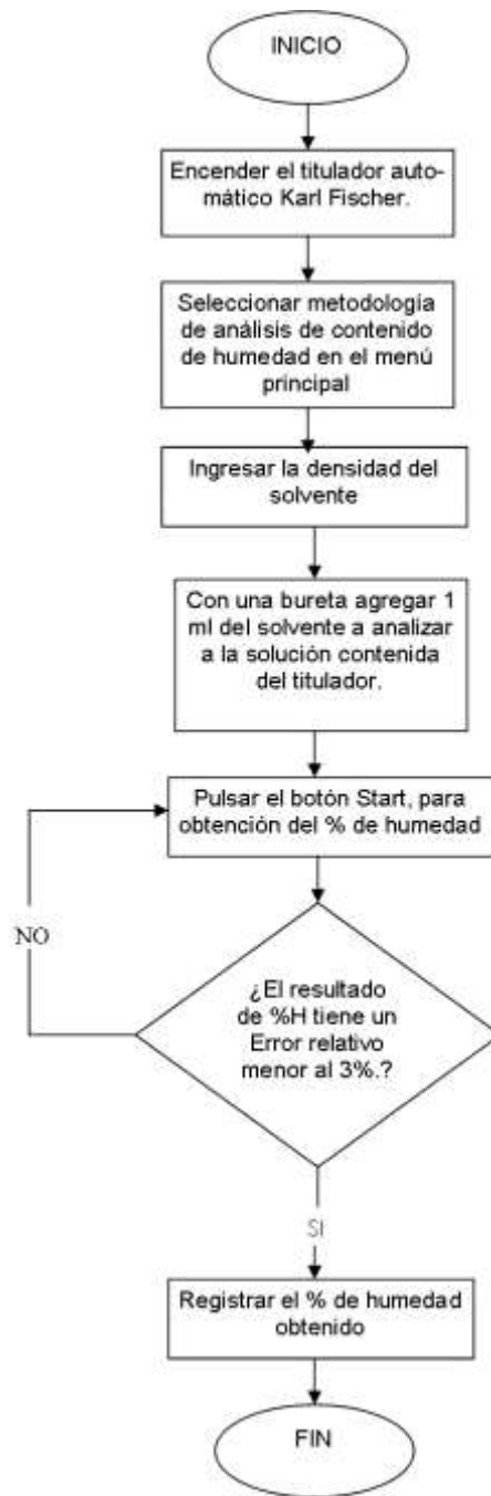
Figura 8. Determinación del contenido de humedad en los solventes recuperados
