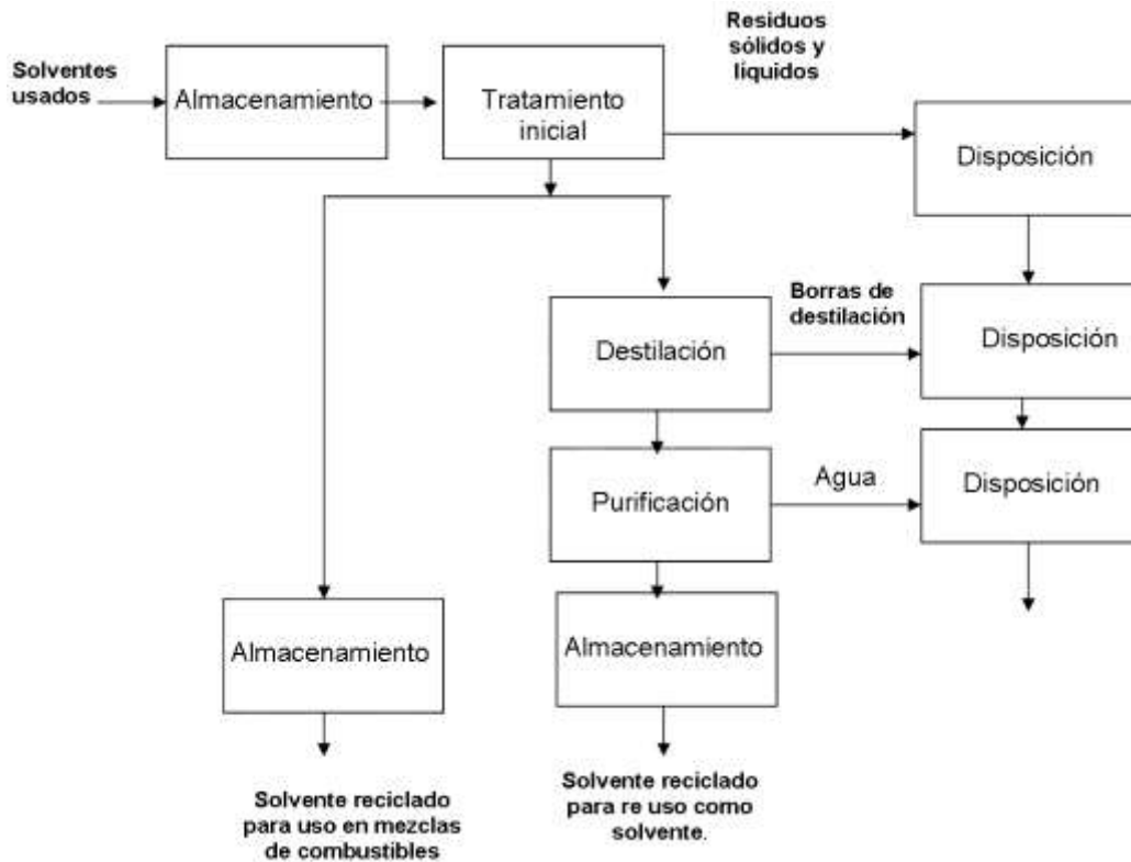
Figura 1. Esquema general del proceso de recuperación de solvente
