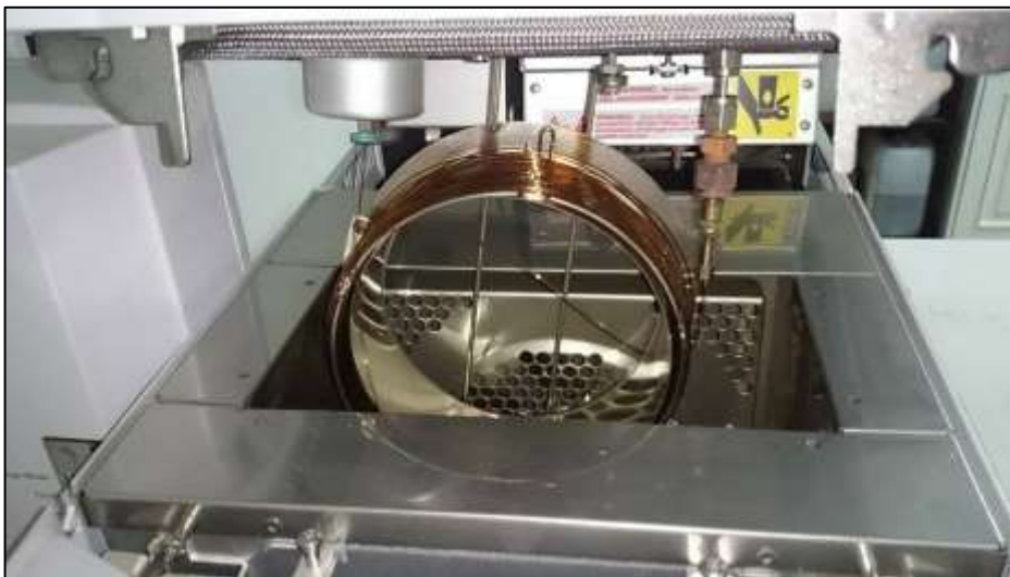
Fotografía de la columna del cromatógrafo.
