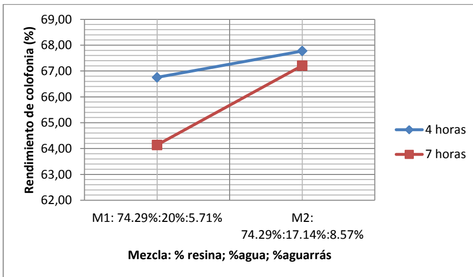
Figura 8. Rendimiento de colofonia obtenida de la resina de pino ocote ( Pinus oocarpa schiede ex schltdl ) respecto a la formulación de la mezcla trabajada para cada tiempo de extracción
