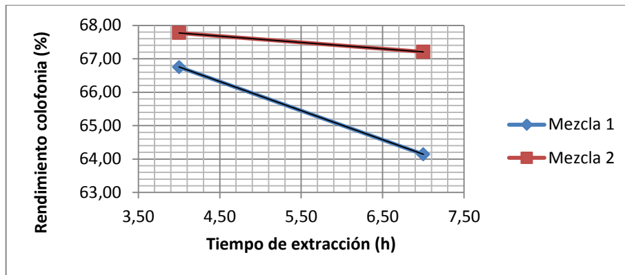
Figura 11. Rendimiento de colofonia obtenida de la resina de pino ocote ( Pinus oocarpa schiede ex schtdl ) en función del tiempo de extracción en cada mezcla trabajada
