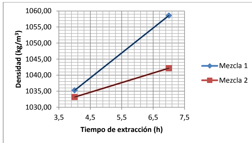
Figura 9. Densidad de colofonia obtenida de la resina de pino ocote ( Pinus oocarpa schiede ex schltdl ) en función del tiempo de extracción en cada mezcla trabajada
