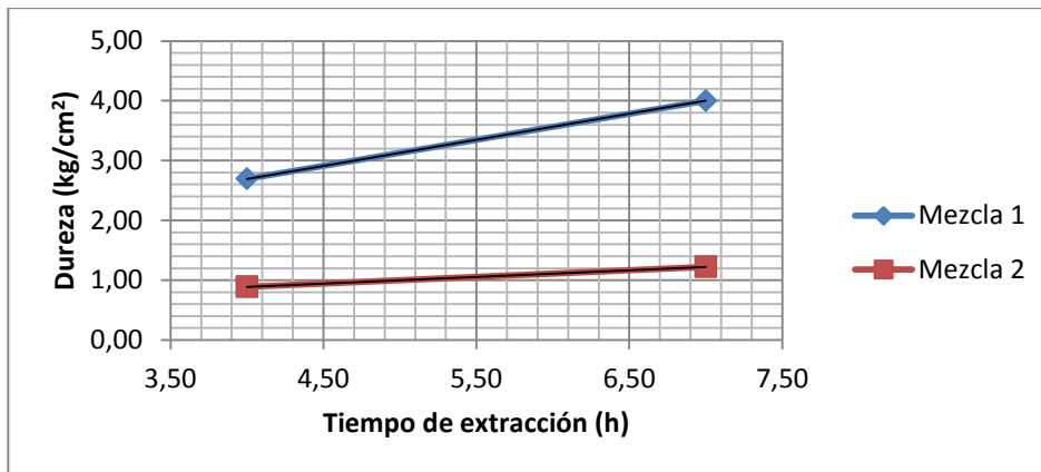
Figura 10. Dureza de colofonia obtenida de la resina de pino ocote ( Pinus oocarpa schiede ex schltdl ) en función del tiempo de extracción en cada mezcla trabajada
