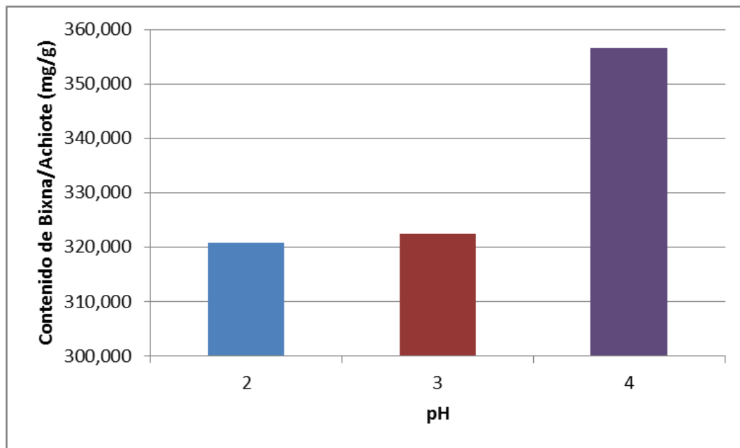
Figura 25. Cuantificación de bixina en el extracto colorante de achiote ( Bixa orellana L. ) a nivel laboratorio en función del pH de precipitación
