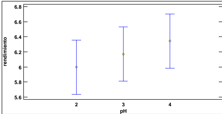
Figura 6. Medias y 95 % de Fisher LSD para el rendimiento extractivo del colorante en función del pH de precipitación
