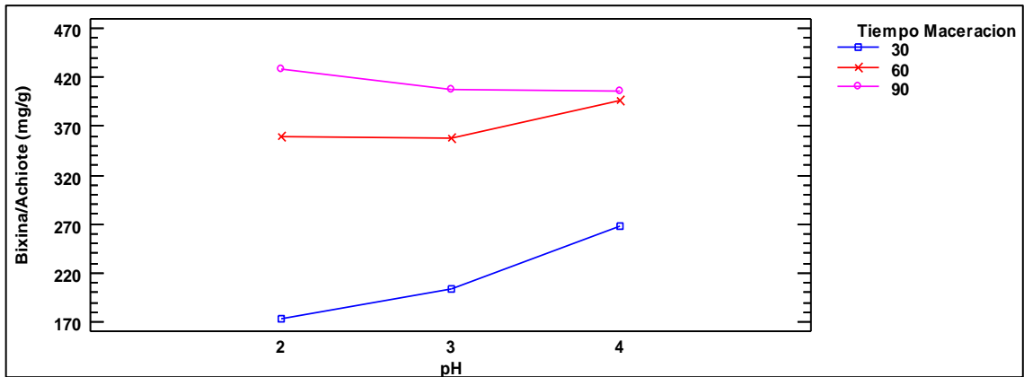
Figura 16. Gráfico de interacciones para cuantificación de bixina en relación a las medias de los factores tiempo de maceración y pH de precipitación
