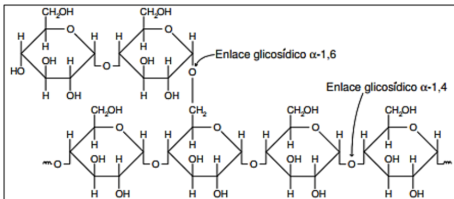
Figura 2. Estructura de segmentos de la amilopectina
