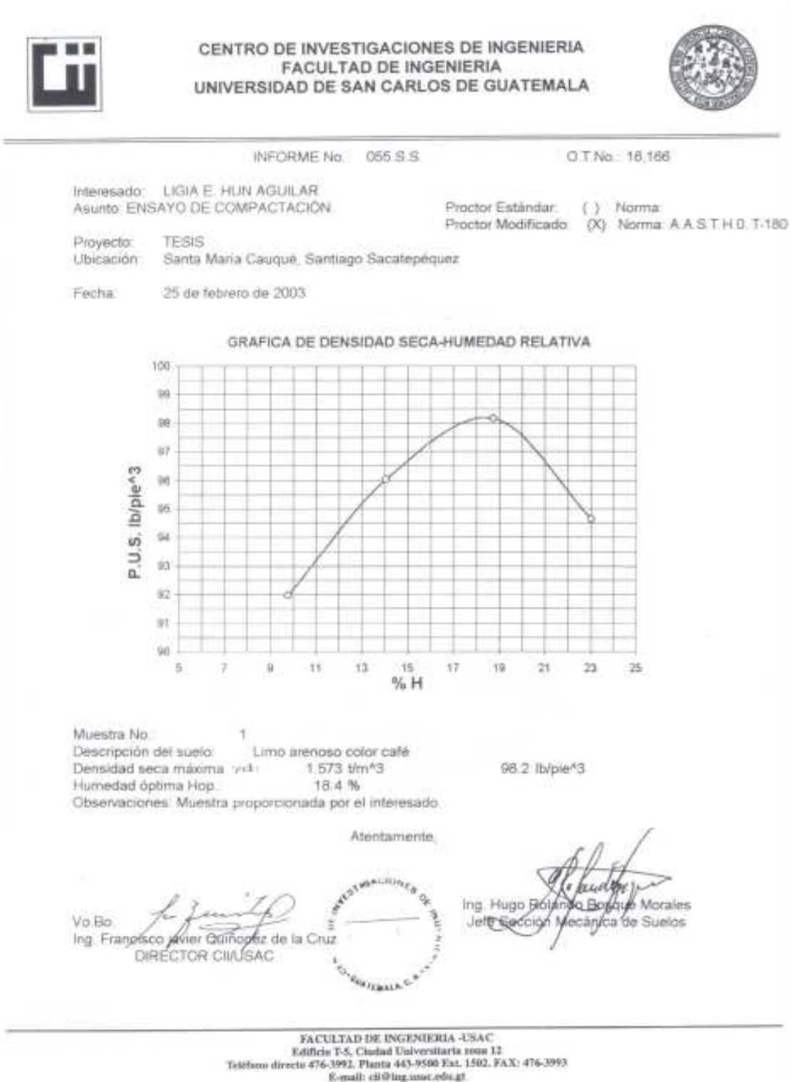
Figura 20. Ensayo de compactación
