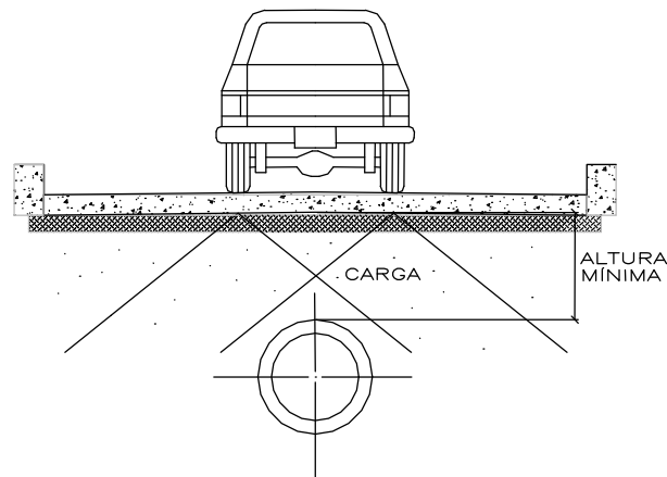
Figura 7. Profundidad de la tubería
