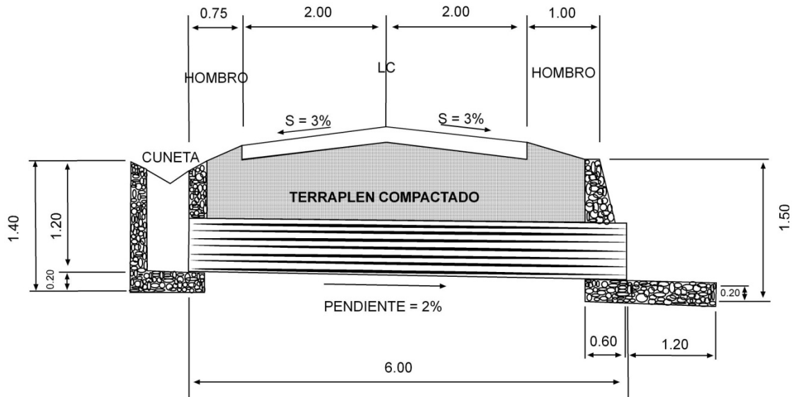
Figura 16 Sección de drenaje transversal
