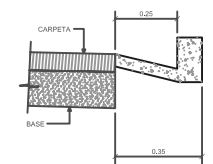
DETALLE DE CUNETETA ESC. 1:10
