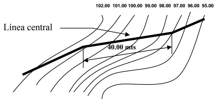
Figura 5 Conservación de Pendiente
