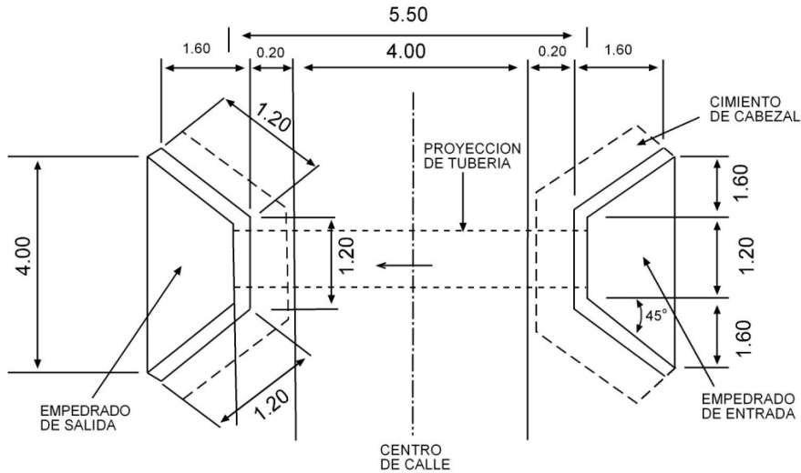
Figura 21 Planta tubería Ø 36” con aletones
