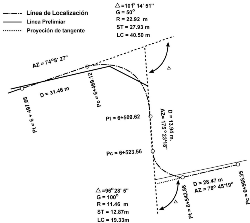
Figura 11 Ejemplo de curvas horizontales
