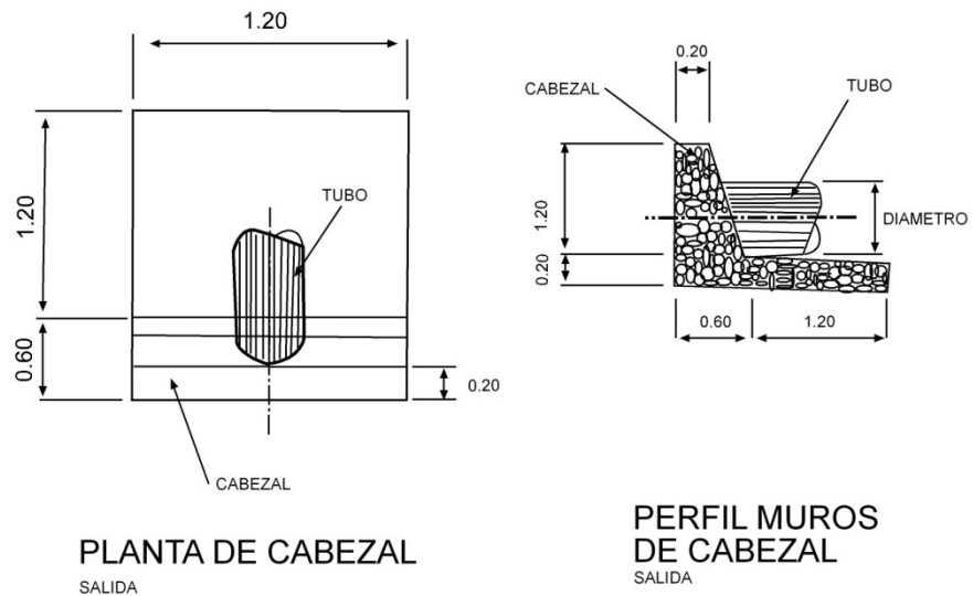
Figura 19 Detalles de cabezales de salida
