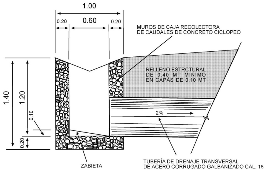
Figura 18 Sección de caja colectora de caudales o caja de cabecera
