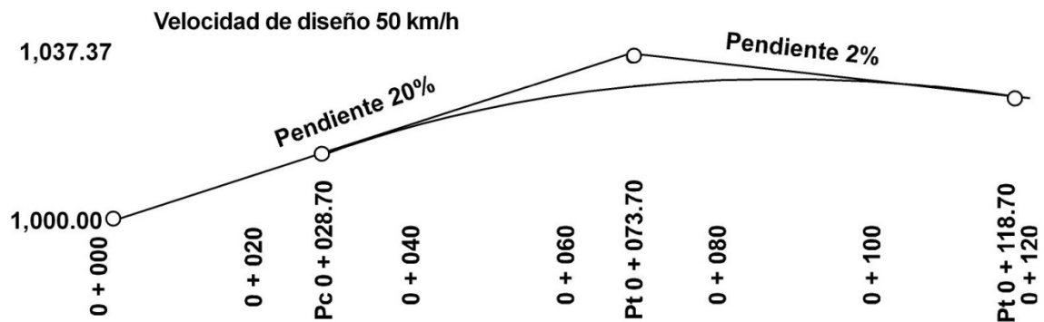
Figura 13 Ejemplo de curva vertical
