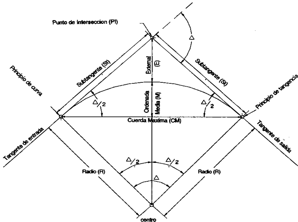
Figura 10 Elementos que conforman una curva horizontal
