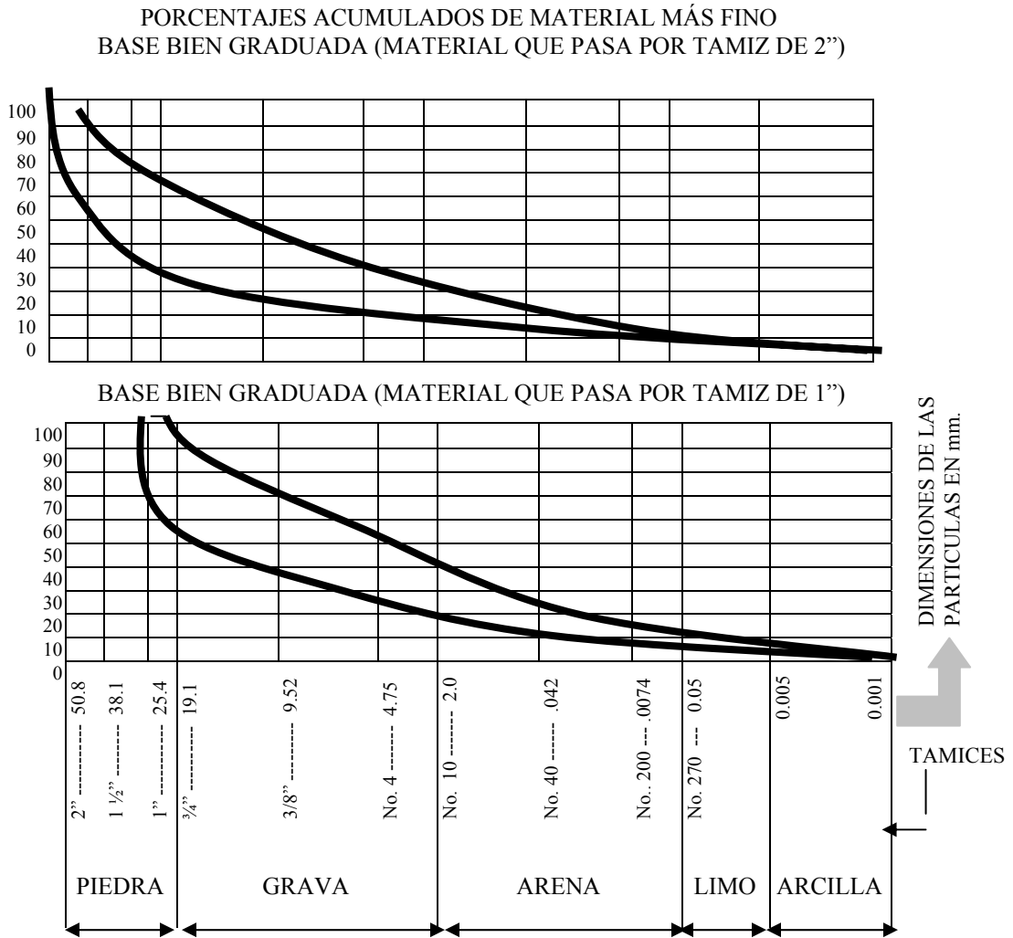
Figura 22 Curvas de granulometría para bases.
