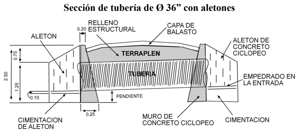
Figura 20 Detalle de drenaje transversal con aletones
