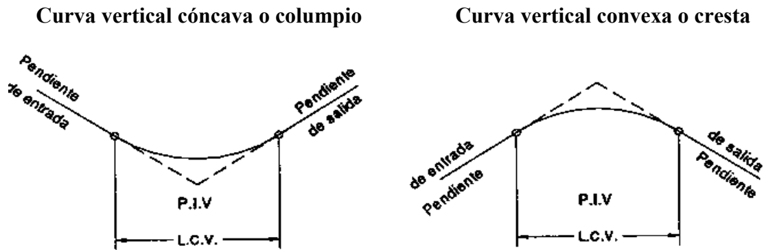
Figura 12 Tipos de curva vertical
