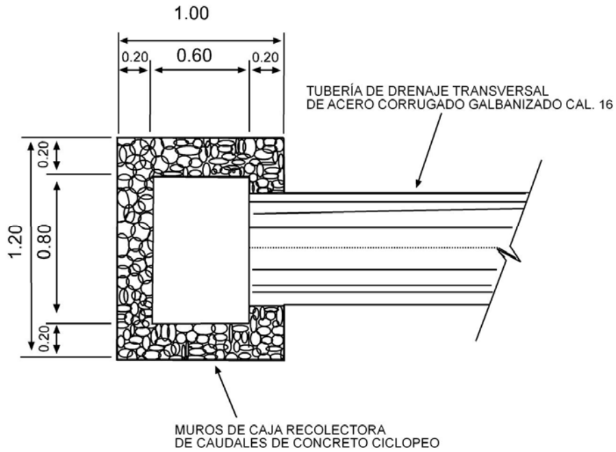
Figura 17 Planta de caja colectora de caudales o caja de cabecera.
