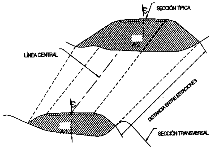
Figura 14 Volumen de relleno
