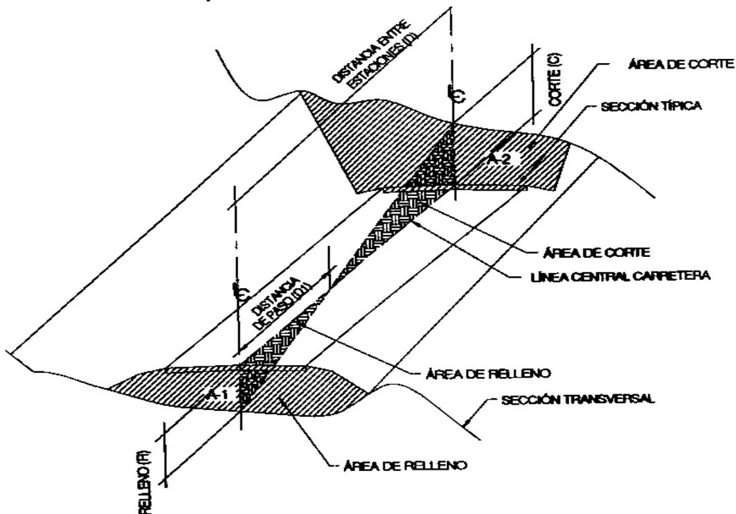
Figura 15 Distancia de paso
