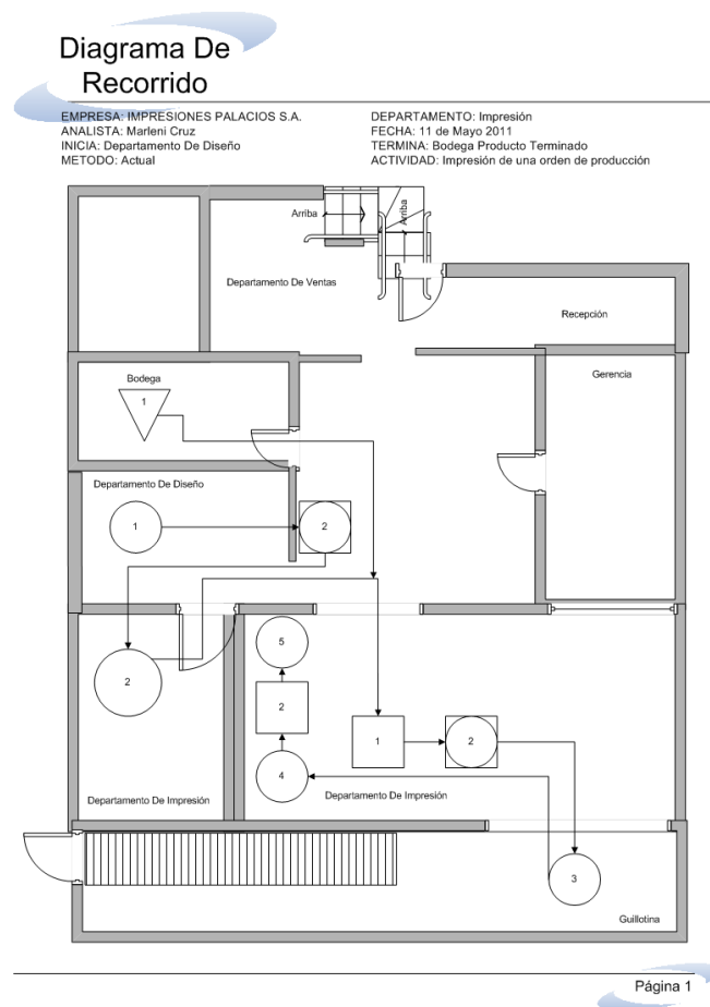
Figura 8. Diagrama de recorrido
