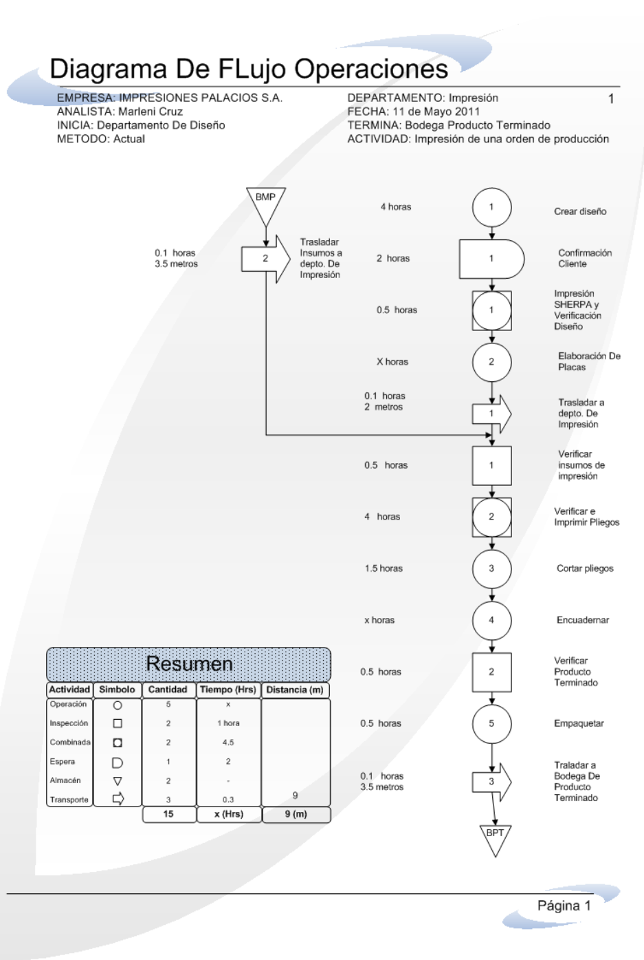
Figura 6. Diagrama de flujo de operaciones
