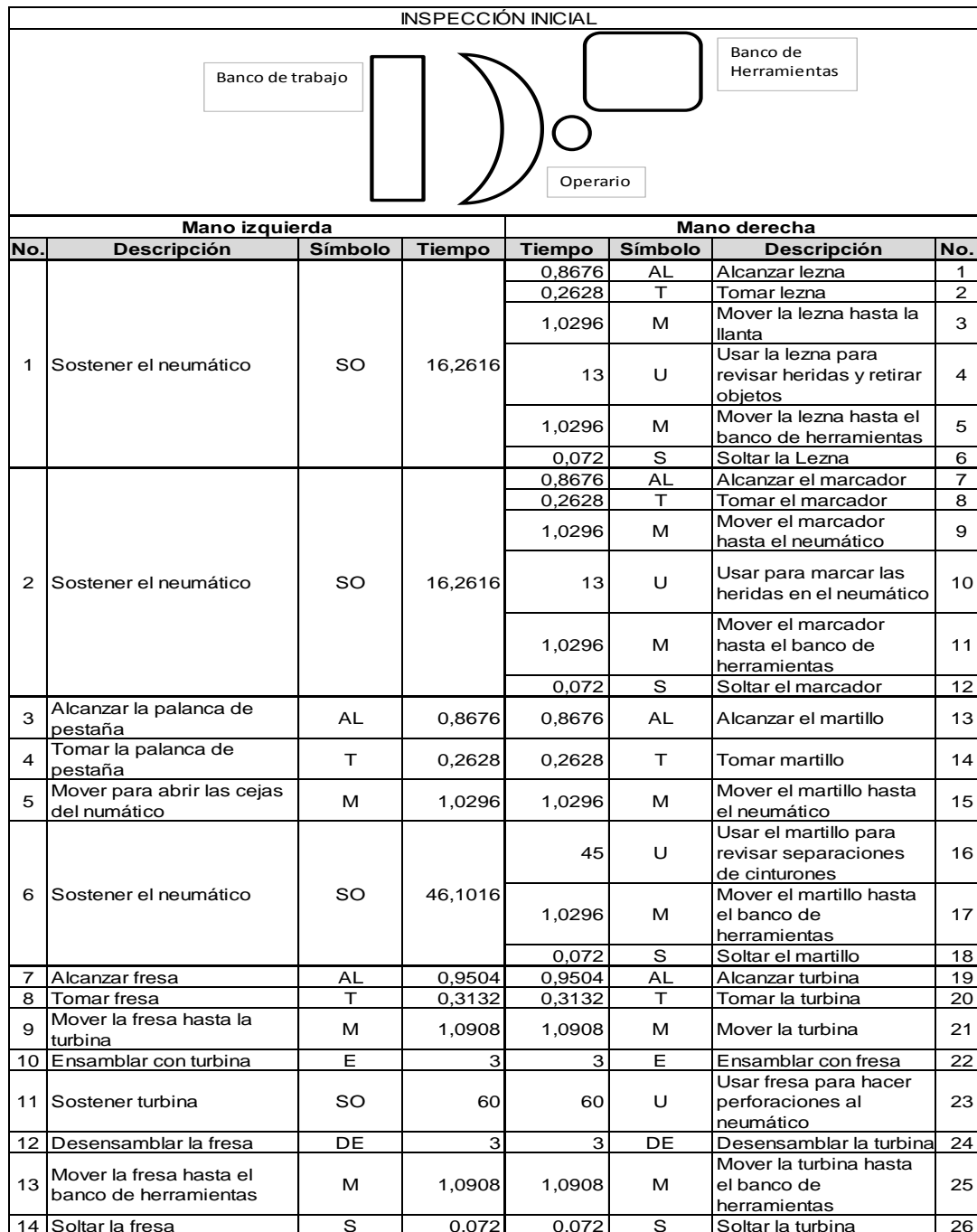
Figura 51. Diagrama bimanual de inspección inicial
