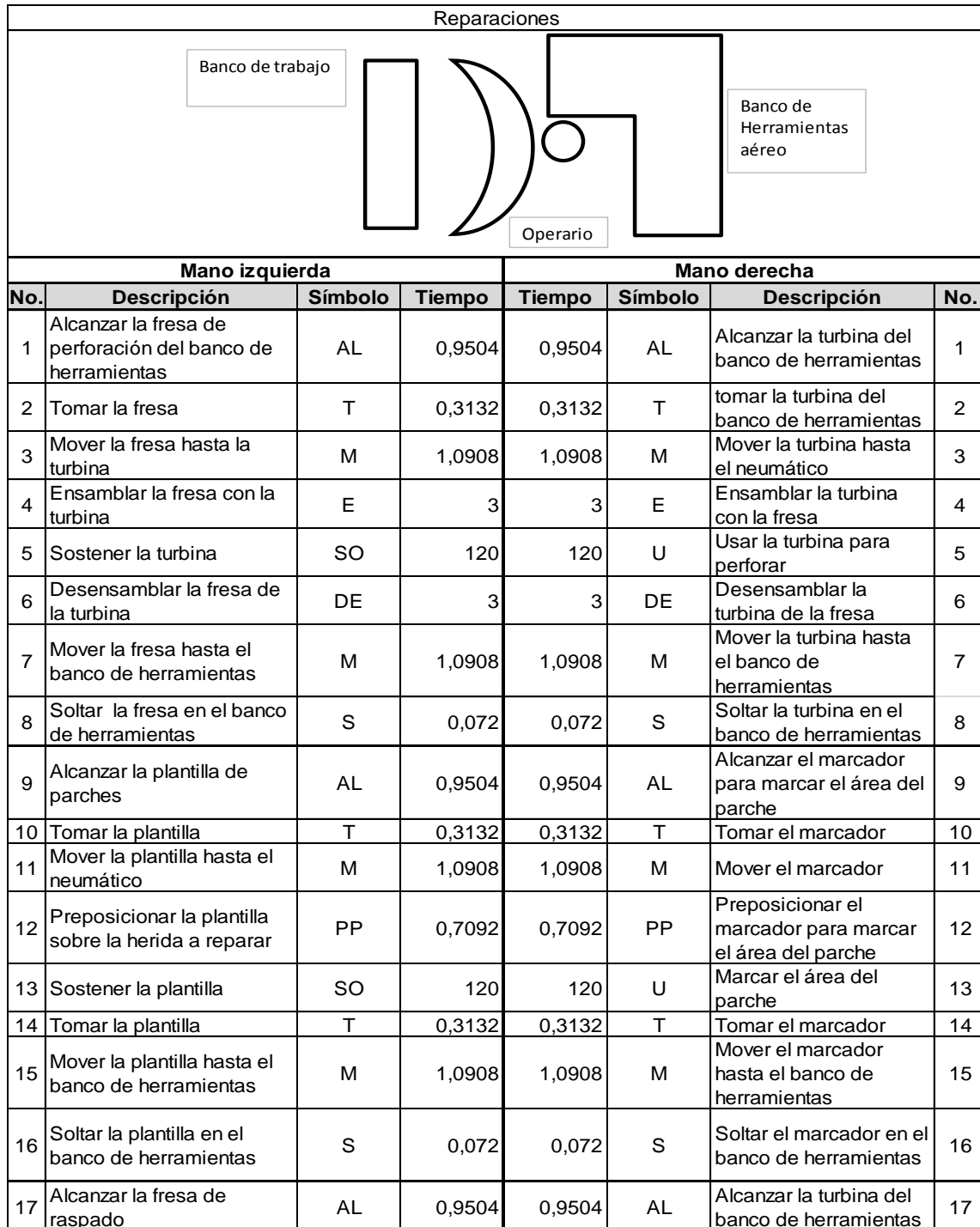
Figura 53. Diagrama bimanual de reparaciones
