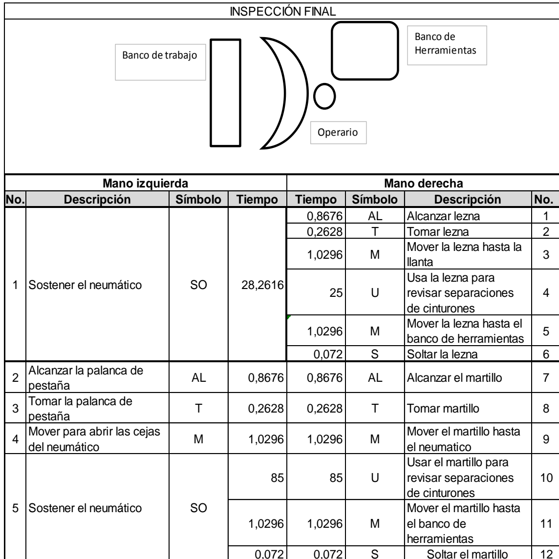
Figura 55. Diagrama bimanual de inspección final
