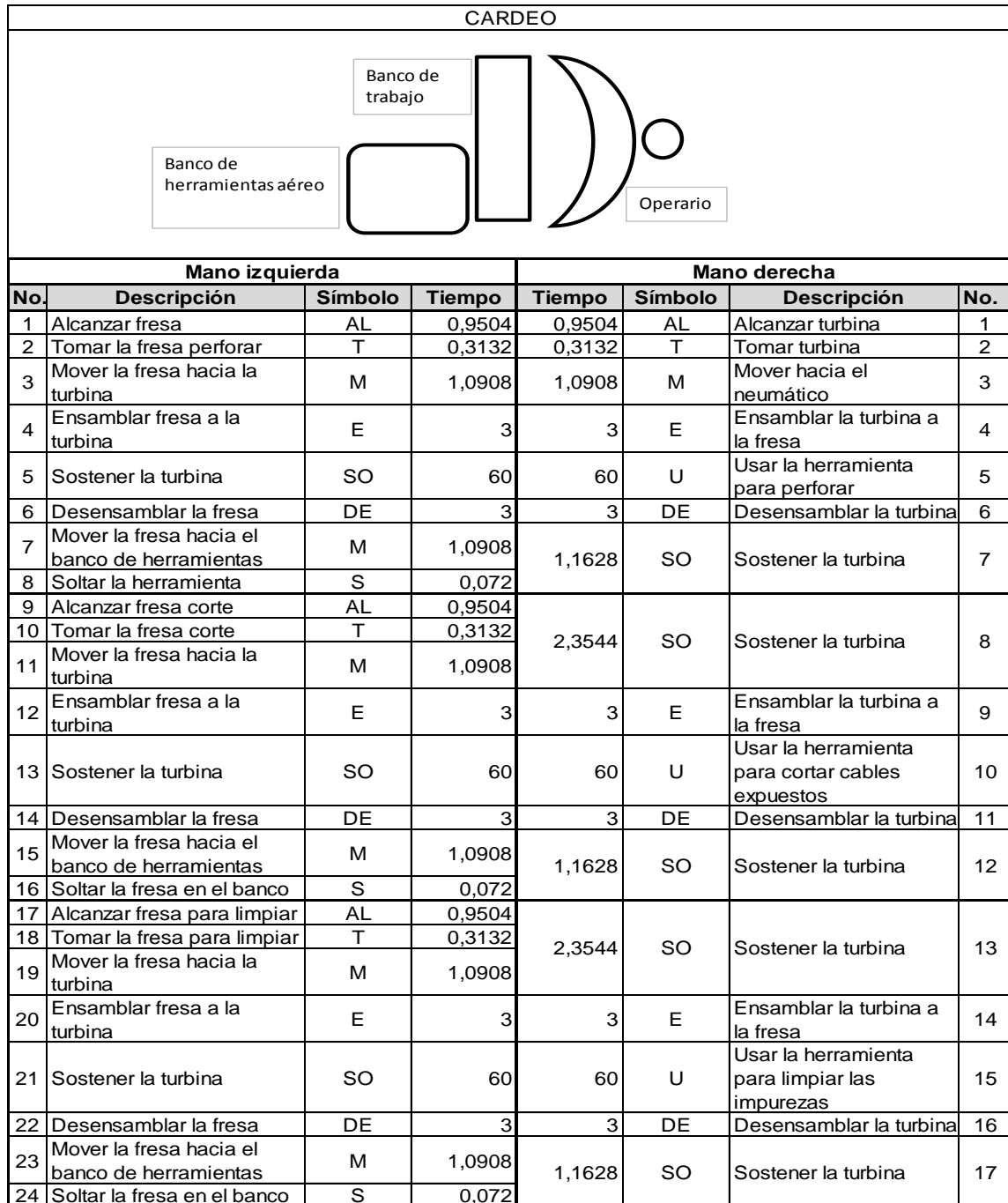
Figura 52. Diagrama bimanual de Cardeo
