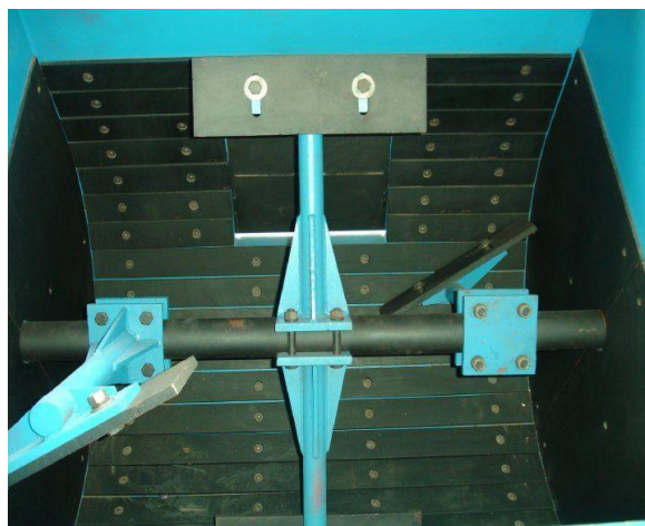
Figura 40. Interior de mezcladora horizontal
