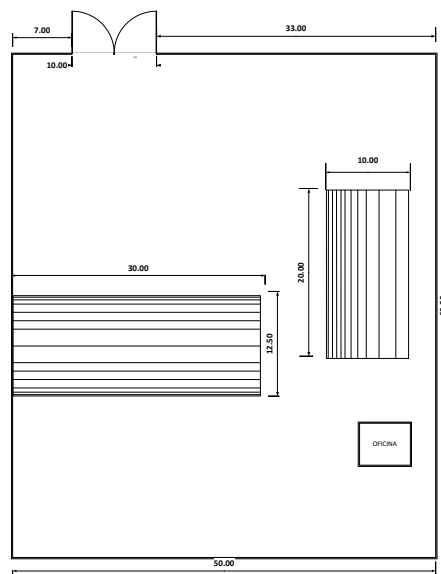
Figura 50. Techo planta piloto
