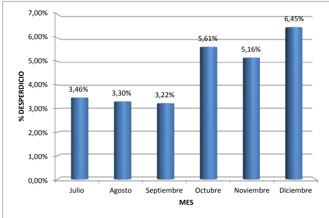
Figura 20. Gráfica de merma de laminado maquinaria tipo 3
