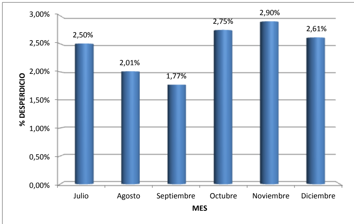
Figura 19. Gráfica de merma de laminado maquinaria tipo 2
