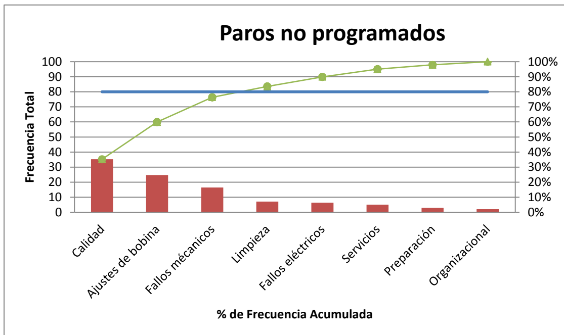
Figura 6. Pareto de maquinaria tipo 3
