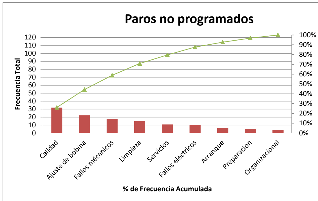
Figura 5. Pareto de maquinaria tipo 2
