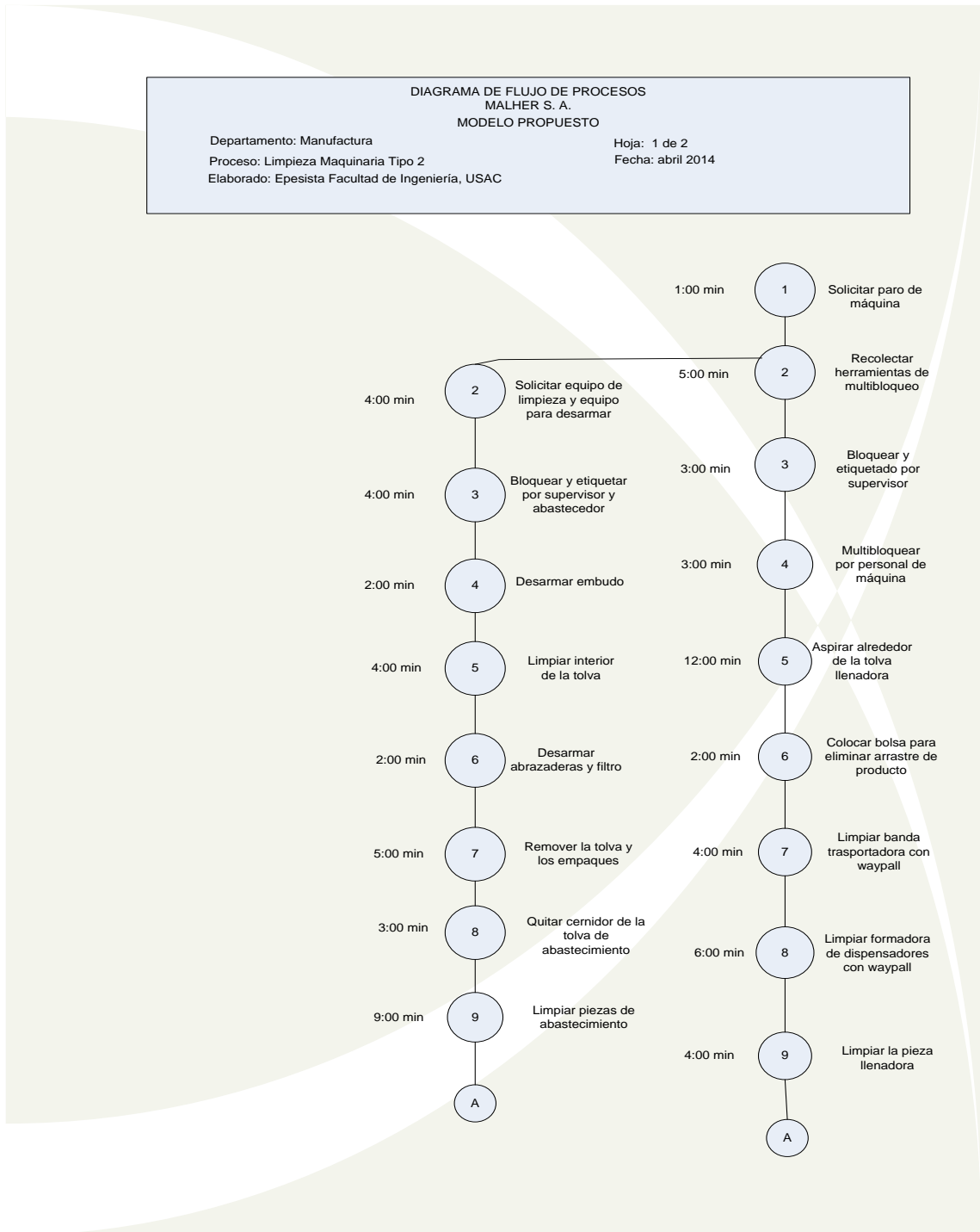
Figura 45. Diagrama de Flujo de operaciones maquinaria tipo 2
