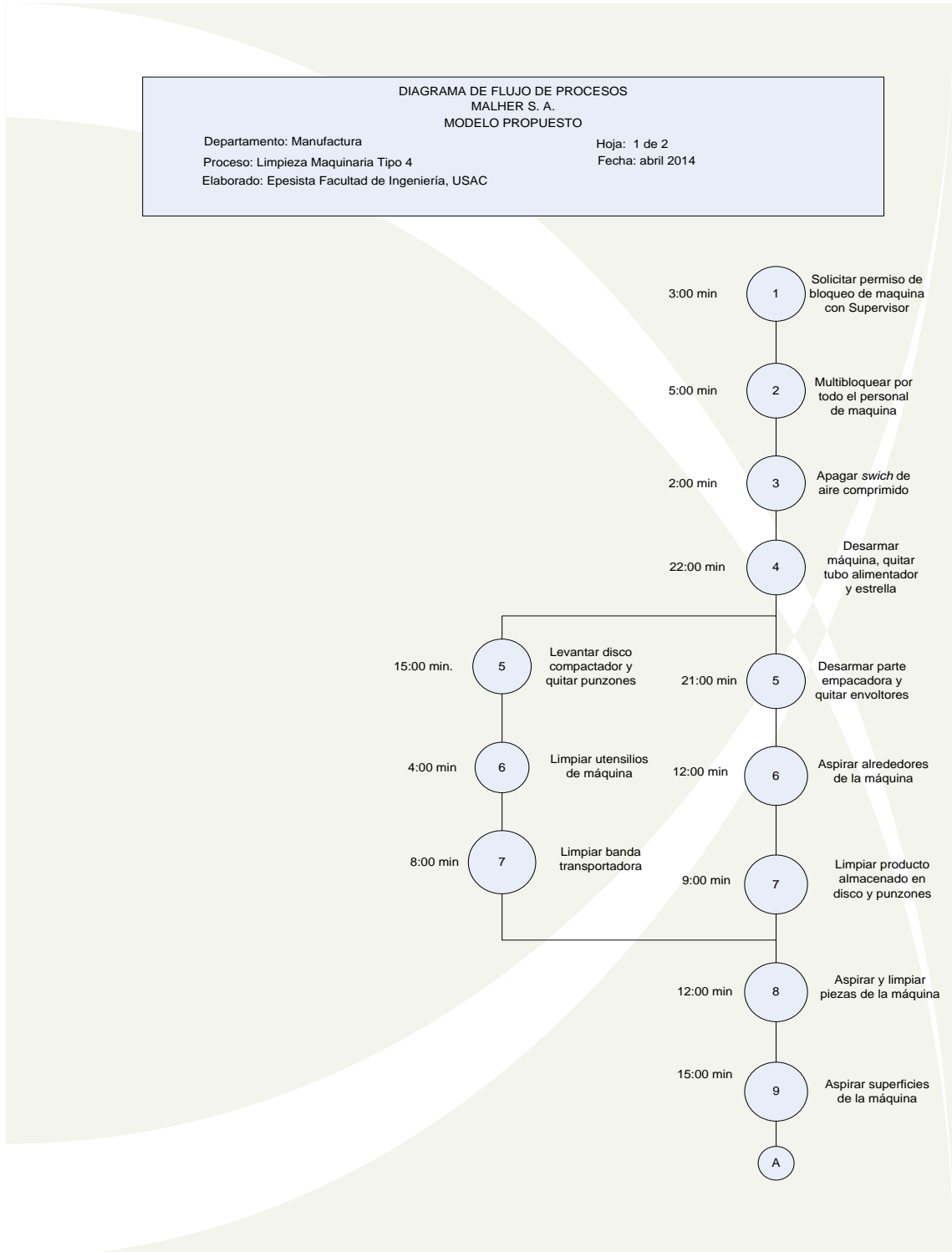
Figura 47. Diagrama de Flujo de limpieza maquinaria tipo 4
