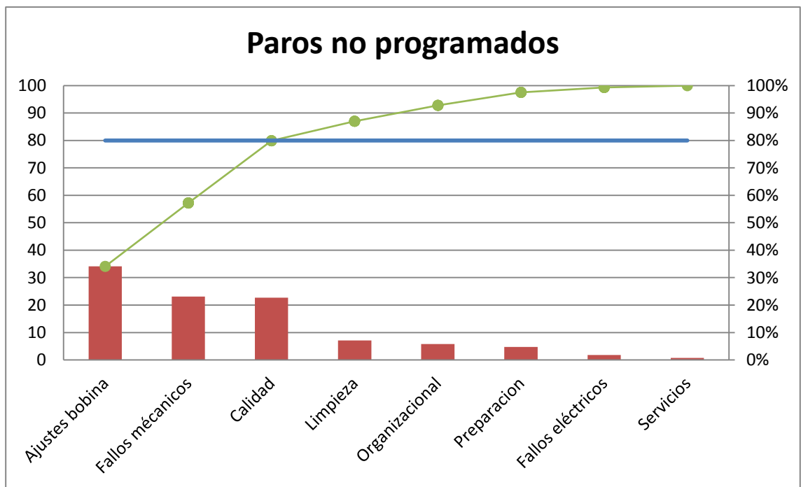
Figura 4. Pareto de maquinaria tipo 1
