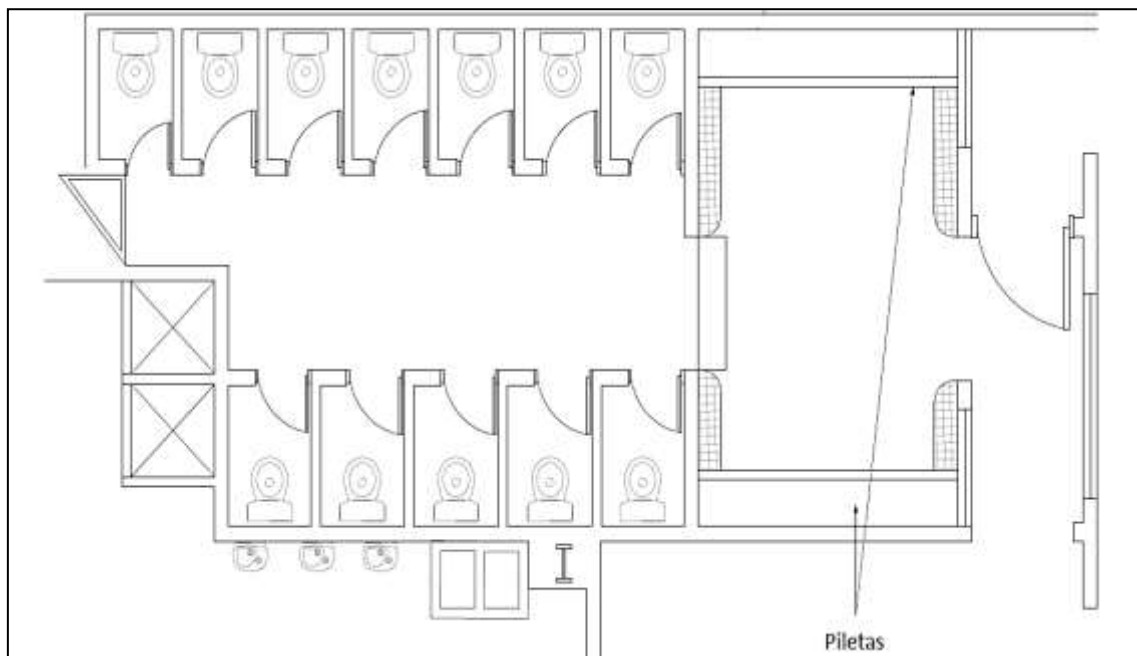
Figura 53. Diseño de sanitarios de damas
