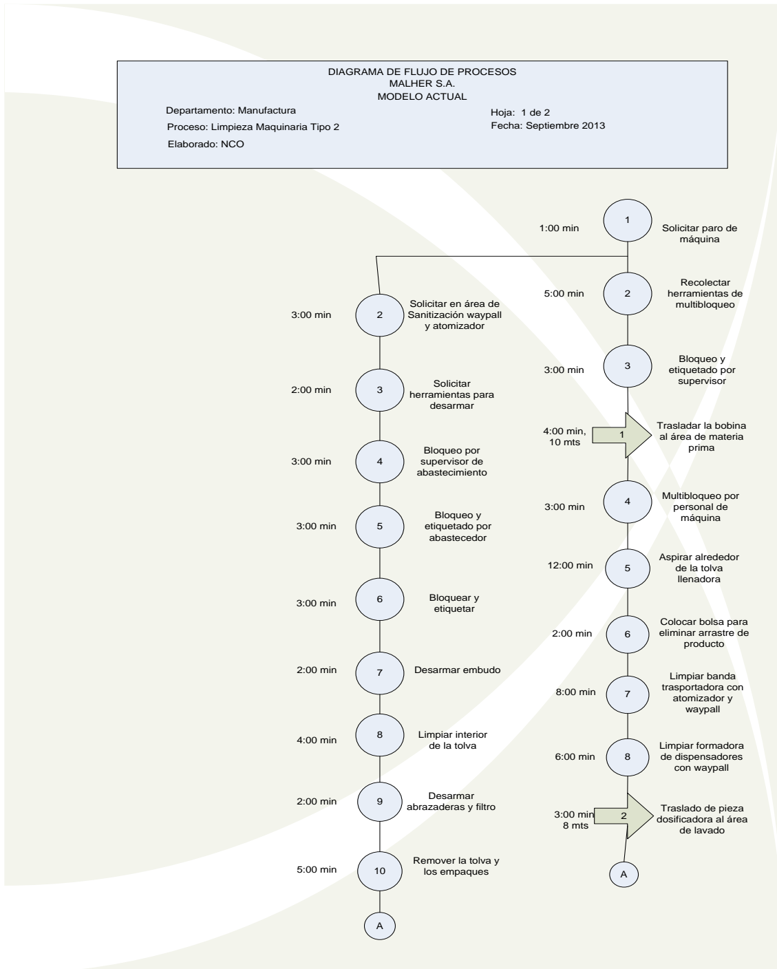
Figura 25. Diagrama de Flujo limpieza de maquinaria tipo 2
