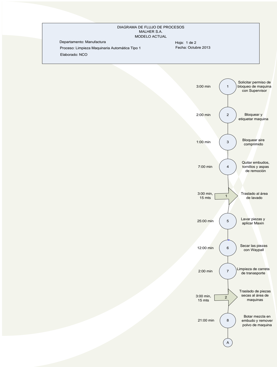
Figura 23. Diagrama de Flujo de limpieza maquinaria tipo 1 automática
