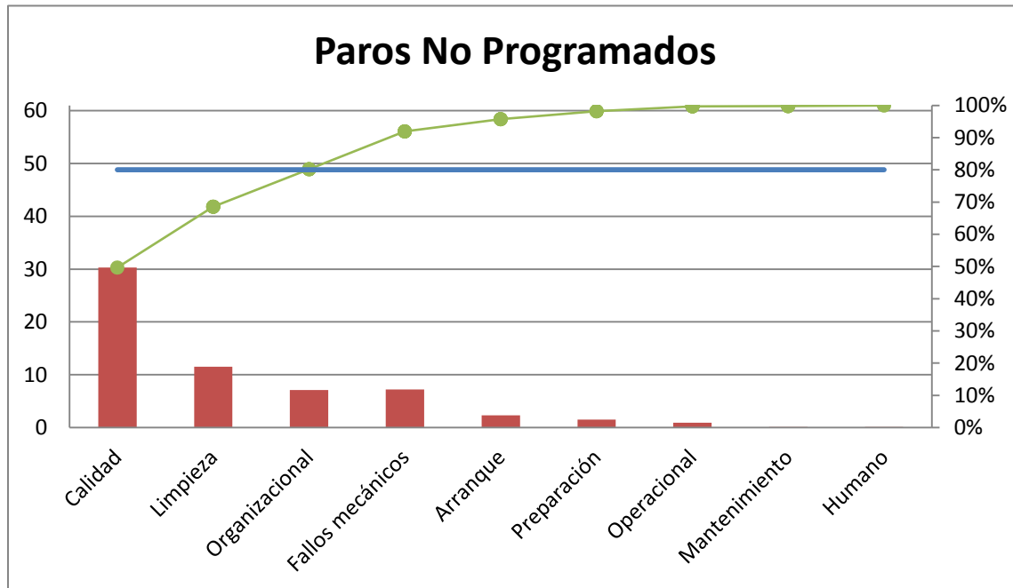
Figura 7. Pareto de maquinaria tipo 4
