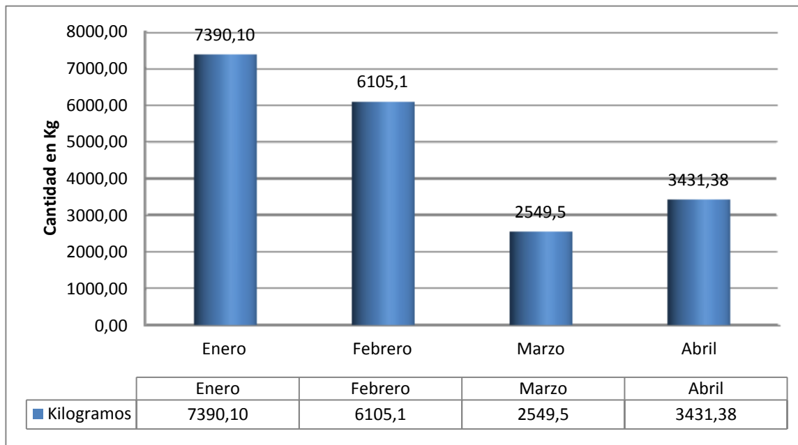
Figura 37. Gráfica de reproceso de maquinaria tipo 3
