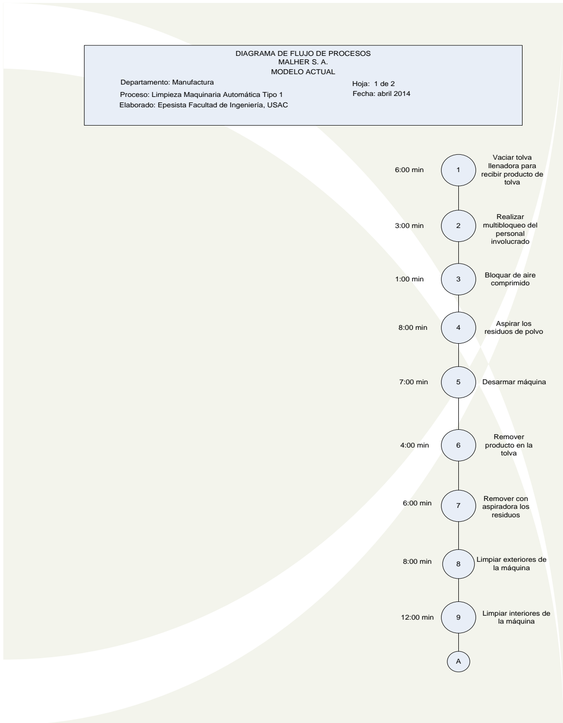
Figura 44. Diagrama de Flujo de limpieza maquinaria automática tipo 1
