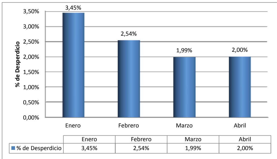
Figura 39. Gráfica de merma de laminado maquinaria tipo 2
