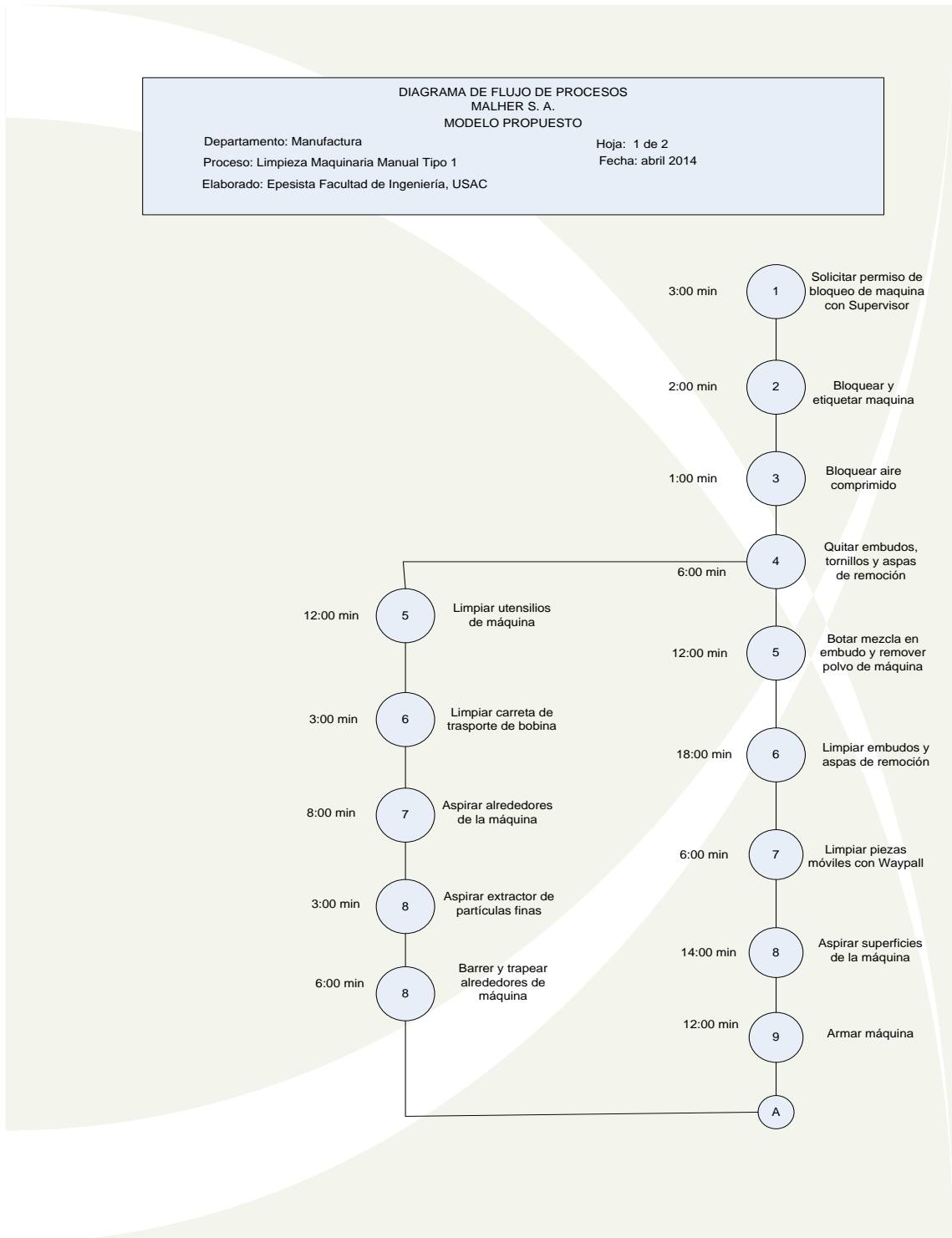
Figura 43. Diagrama de Flujo de limpieza maquinaria manual tipo 1
