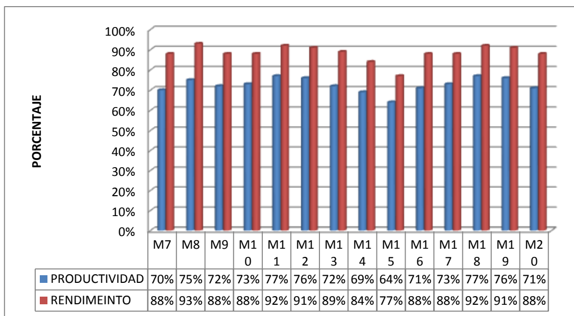
Figura 10. Productividad y rendimiento maquinaria tipo 2
