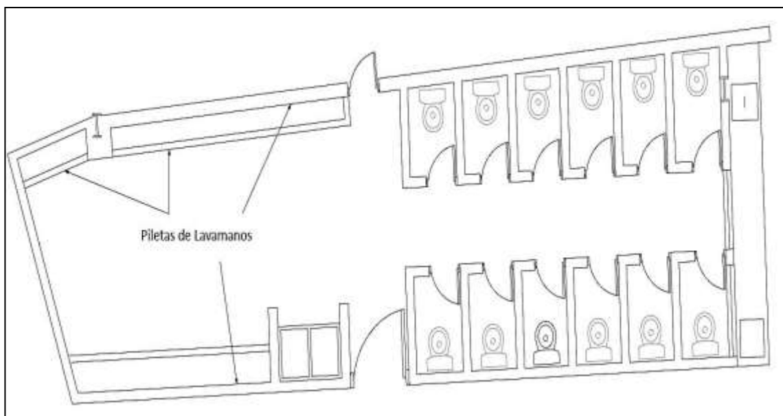
Figura 52. Diseño de sanitarios de caballeros
