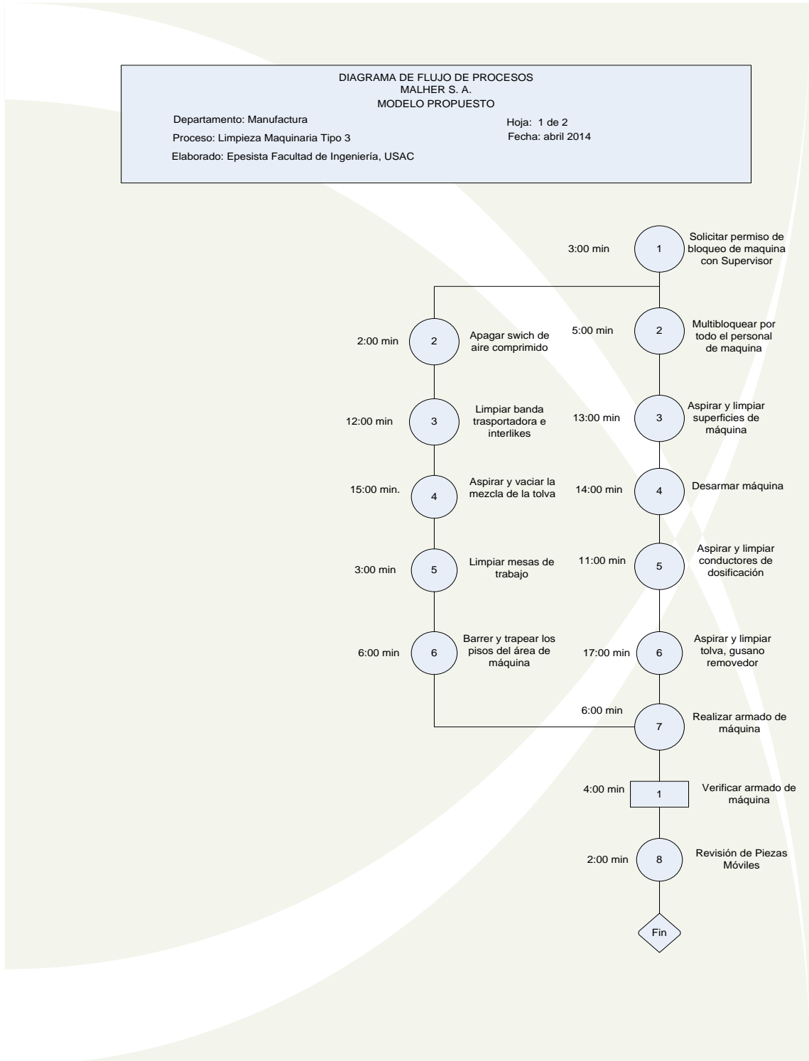
Figura 46. Diagrama de Flujo de limpieza maquinaria tipo 3
