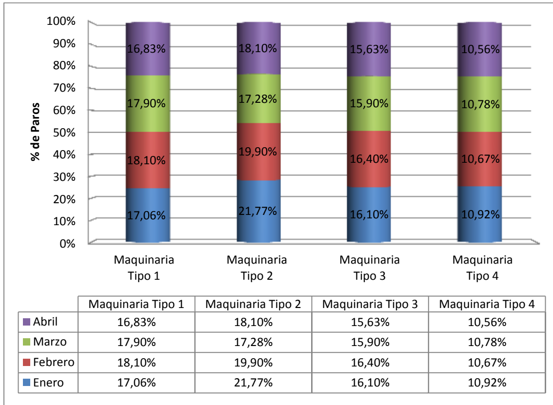
Figura 33. Gráfica paros no programados enero – abril 2014
