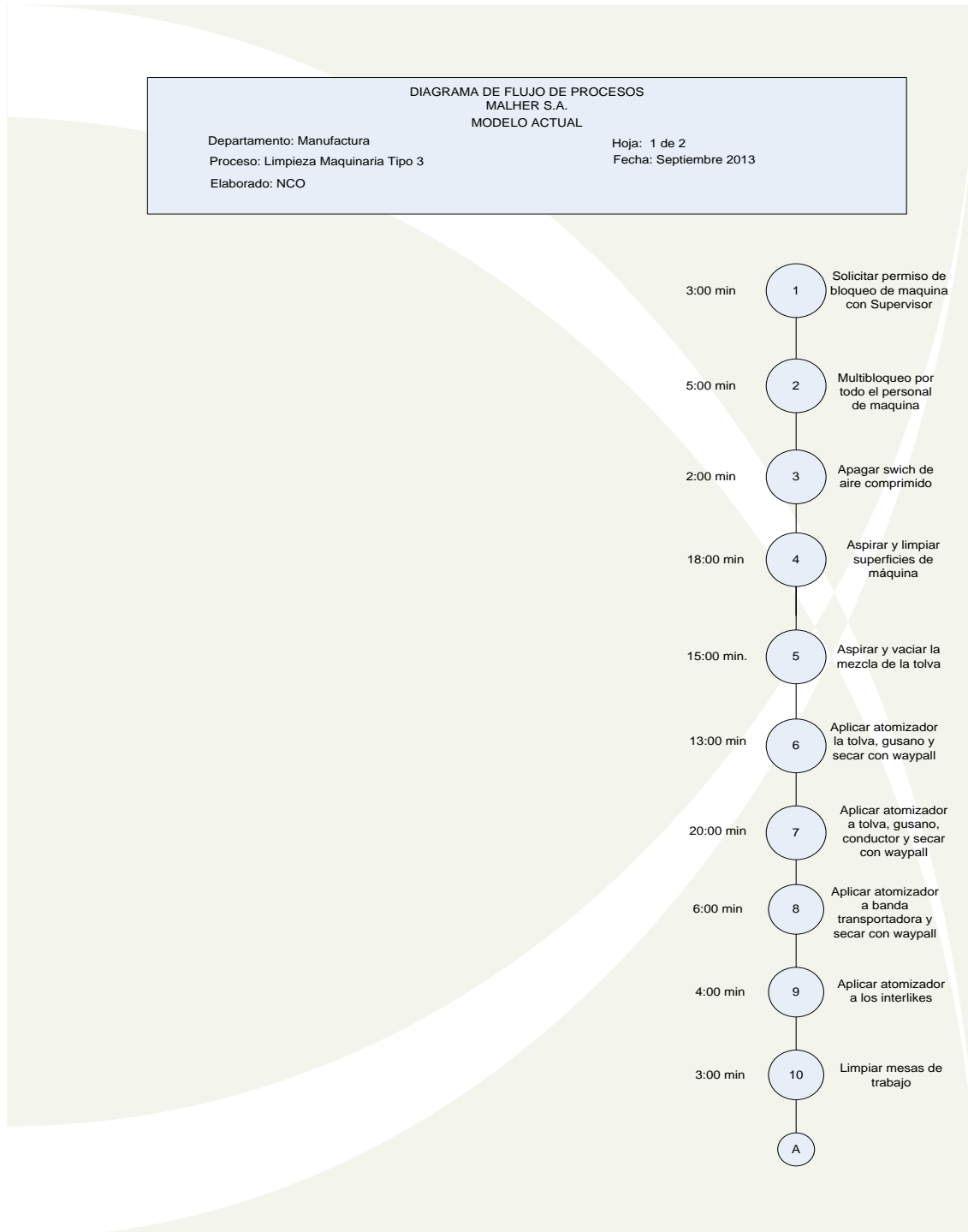
Figura 26. Diagrama de Flujo de limpieza de maquinaria tipo 3
